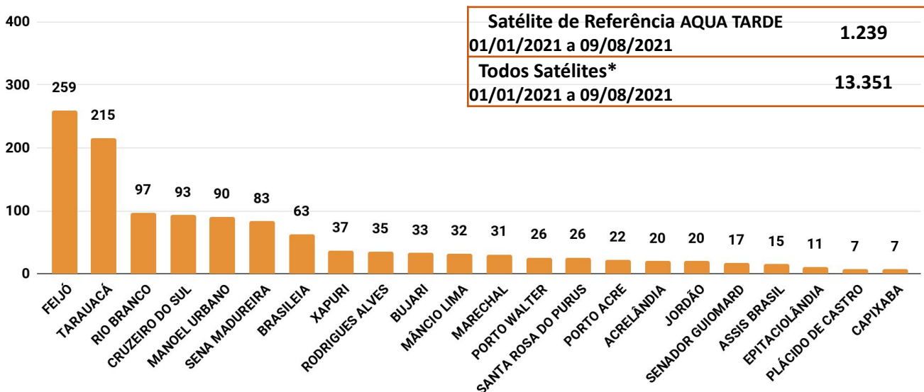
Figura 3 – Distribuição dos focos de queimadas acumulados de 01/01/2021 a 09/08/2021, no Estado do Acre. (Satélite de referência AQUA TARDE)
