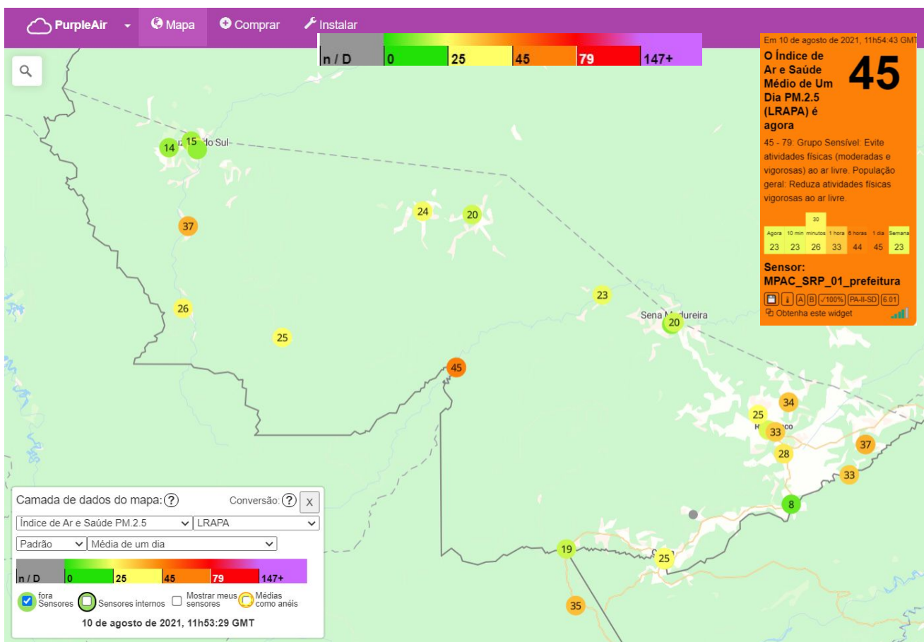
Figura 12 – Média do dia 10/08/2021 com Índice de Ar e Saúde relacionado à concentração do Material Particulado Raw PM 2.5 \mu\text{g}/\text{m}^3
