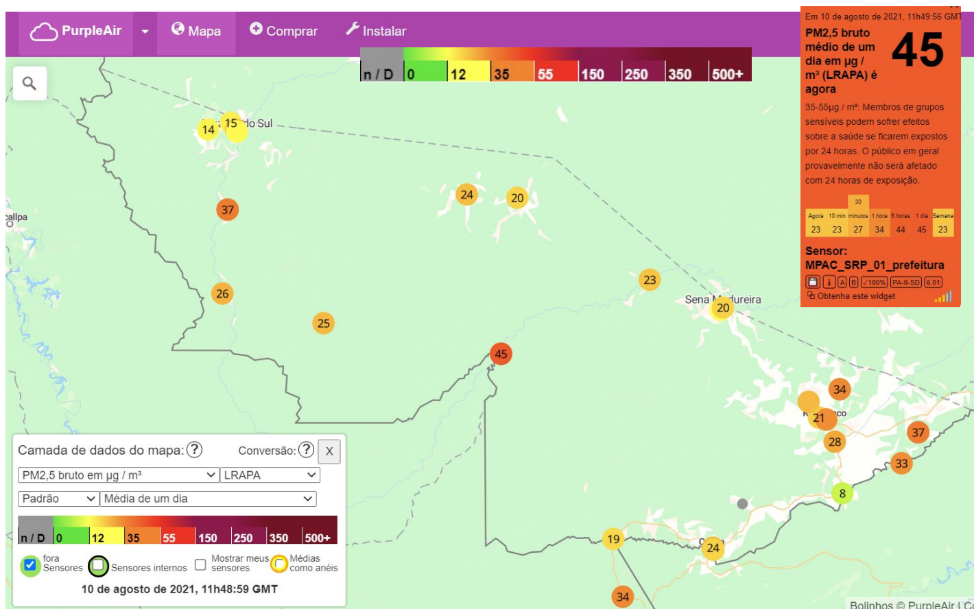
Figura 11 – Concentração de Material Particulado Raw PM 2.5 bruto \mu\text{g}/\text{m}^3 média para dia 10/08/2021
