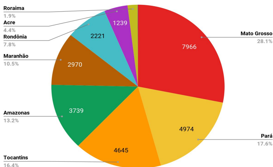
Figura 1 – Distribuição percentual dos focos de queimadas acumulados em 01/01/2021 a 09/08/2021 na Amazônia legal (Satélite de Referência AQUA Tarde)
