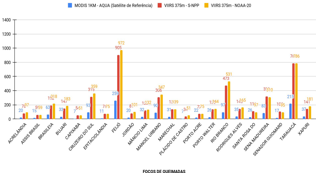
Figura 5 – Distribuição dos focos de queimadas acumulados de 01/01/2021 a 09/08/2021 , no Estado do Acre. Satélite de referência AQUA (Barra de cor azul), VIIRS 375m/S-NPP (Cor vermelha) e VIIRS 375m/NOAA-20 (Cor amarela)
