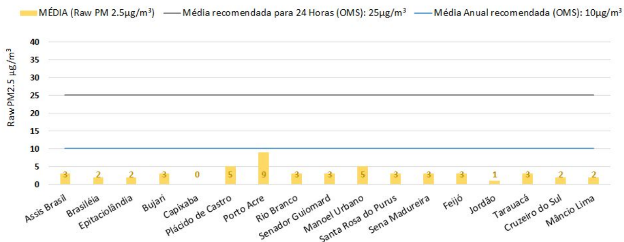
Rede de Monitoramento de Qualidade do Ar, Material Particulado Fino Raw PM2.5 \mu\text{g}/\text{m}^3 Dia: 29/07/2021 - Fonte: PurpleAir
