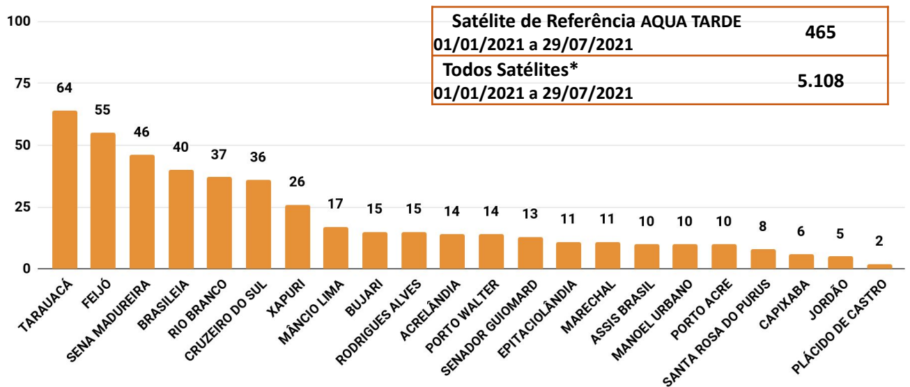
Figura 3 – Distribuição dos focos de queimadas acumulados de 01/01/2021 a 29/07/2021, no Estado do Acre. (Satélite de referência AQUA TARDE)
