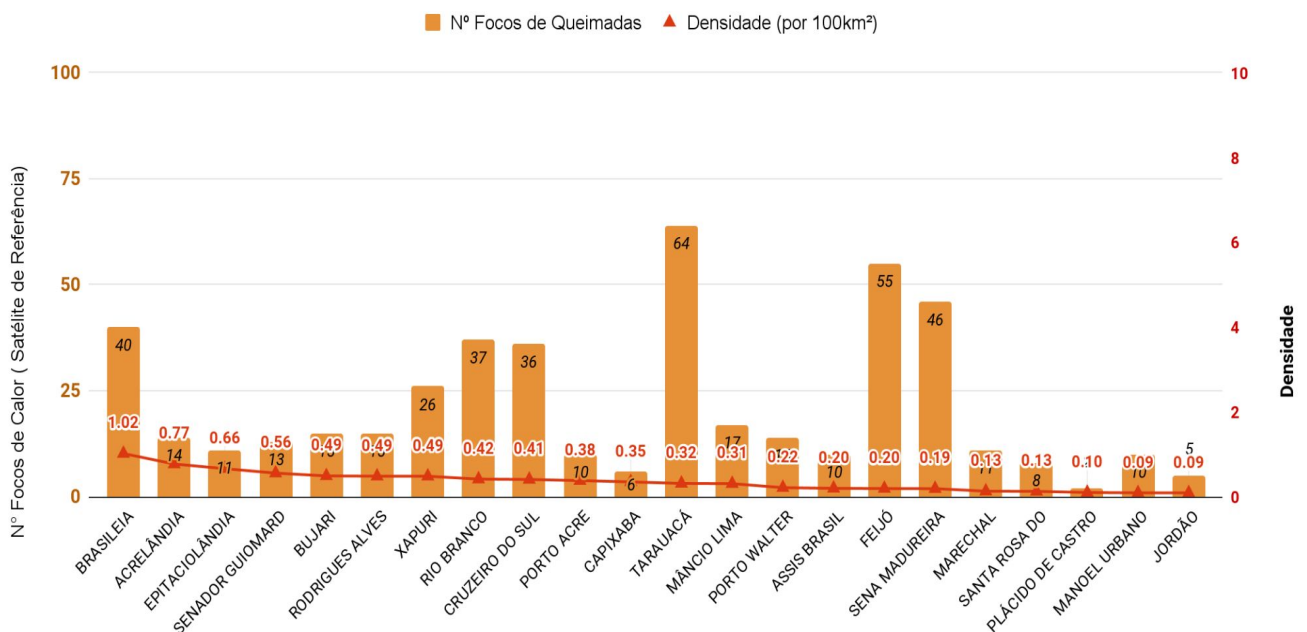
Figura 8 – Ocorrência de focos de queimadas e densidade por km 2 , por município em 01/01/2021 a 29/07/2021 (Satélite de referência AQUA)
