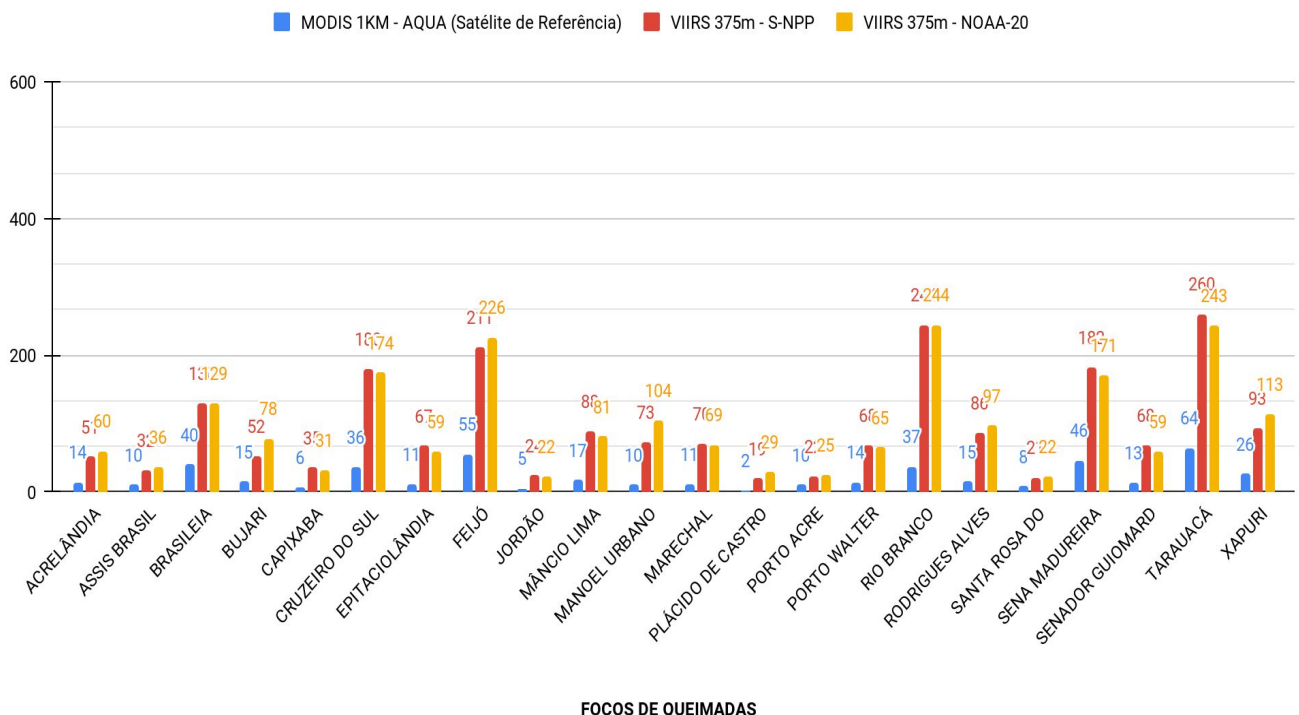
Figura 5 – Distribuição dos focos de queimadas acumulados de 01/01/2021 a 29/07/2021 , no Estado do Acre. Satélite de referência AQUA (Barra de cor azul), VIIRS 375m/S-NPP (Cor vermelha) e VIIRS 375m/NOAA-20 (Cor amarela)
