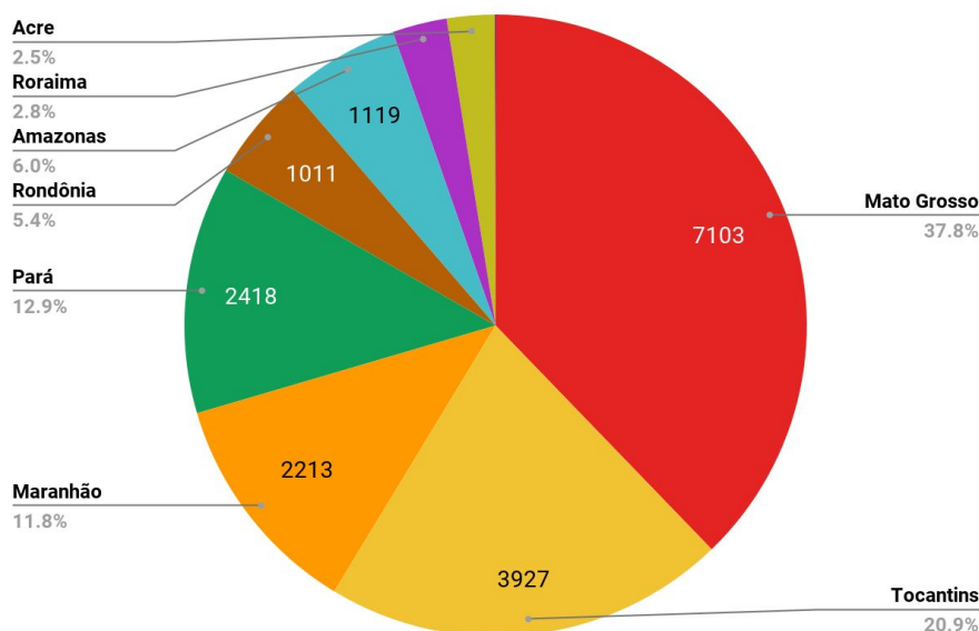
Figura 1 – Distribuição percentual dos focos de queimadas acumulados em 01/01/2021 a 29/07/2021 na Amazônia legal (Satélite de Referência AQUA Tarde)
