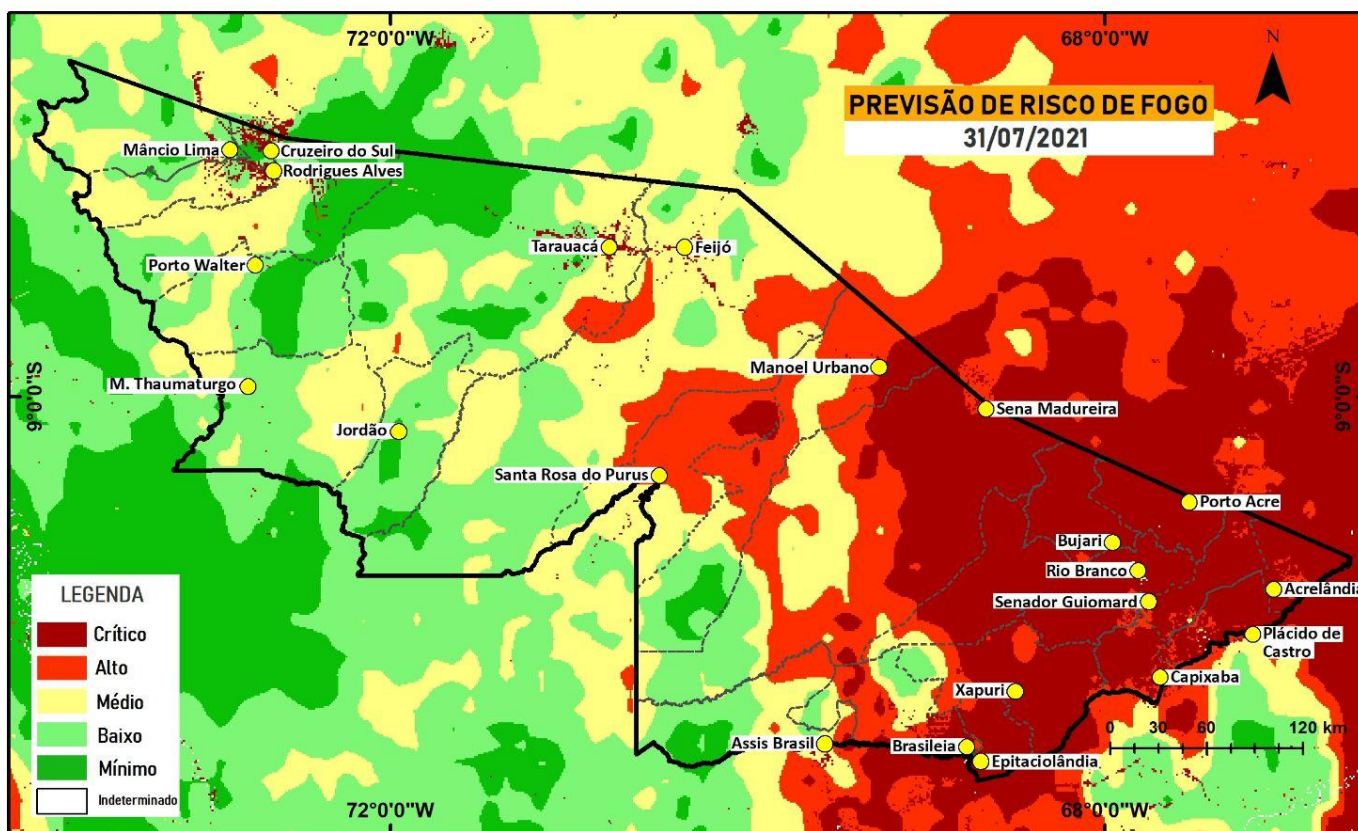
Figura 10 – Risco de Fogo previsto para o estado do Acre para amanhã 31/07/2021
