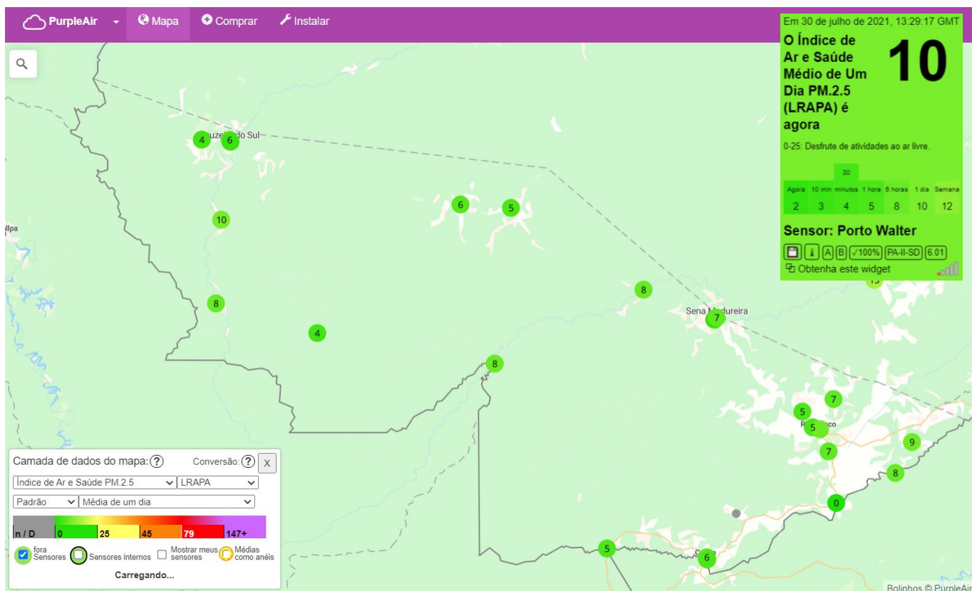
Figura 13 – Média do dia 30/07/2021 de Material Particulado Raw PM 2.5 \mu\text{g}/\text{m}^3
