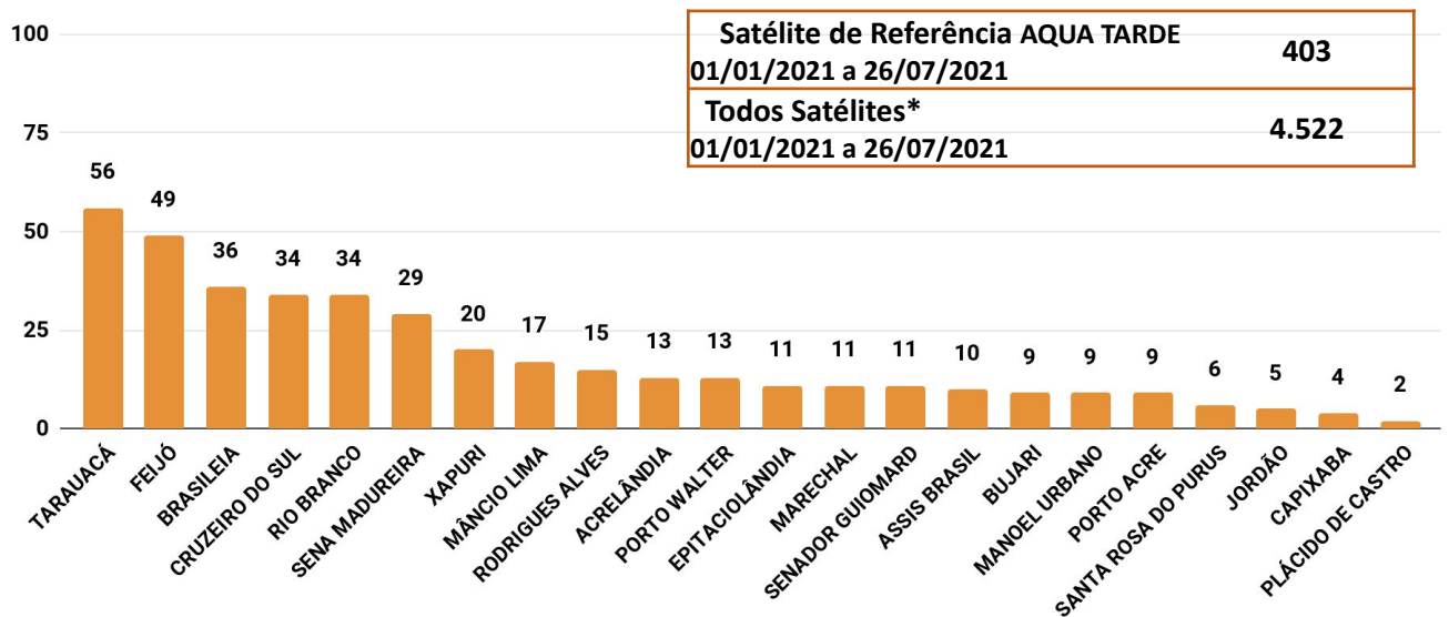
Figura 3 – Distribuição dos focos de queimadas acumulados de 01/01/2021 a 26/07/2021, no Estado do Acre. (Satélite de referência AQUA TARDE)
