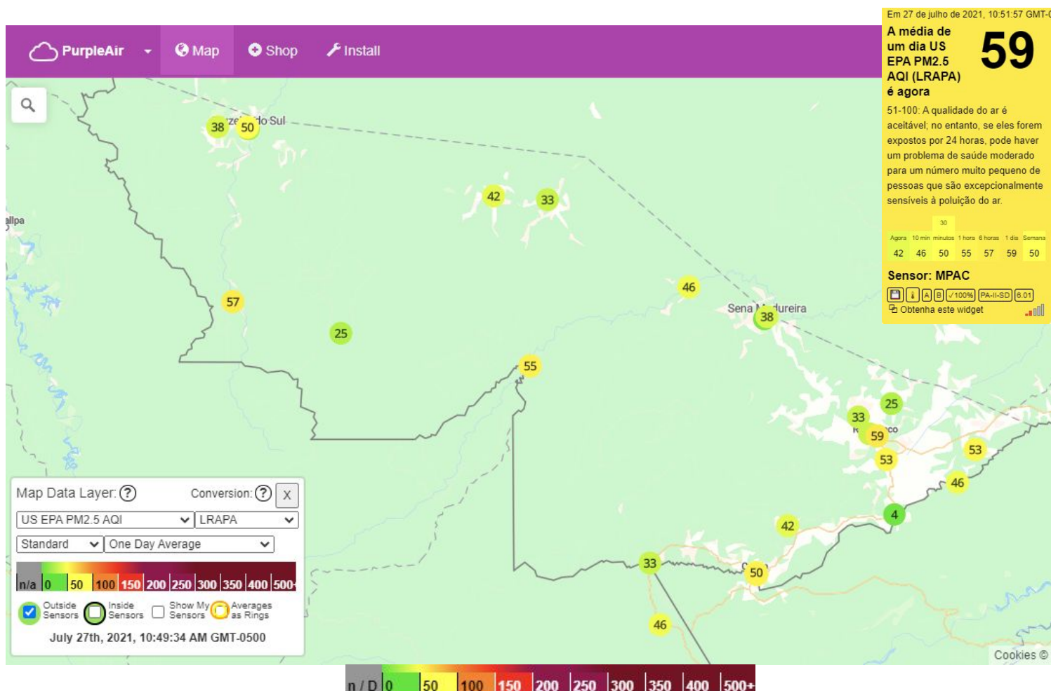
Figura 11 – Média do dia 27/07/2021 de Material Particulado Raw PM 2.5 \mu\text{g}/\text{m}^3
