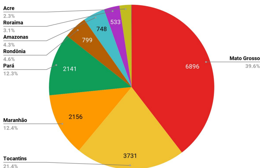
Figura 1 – Distribuição percentual dos focos de queimadas acumulados em 01/01/2021 a 26/07/2021 na Amazônia legal (Satélite de Referência AQUA Tarde)
