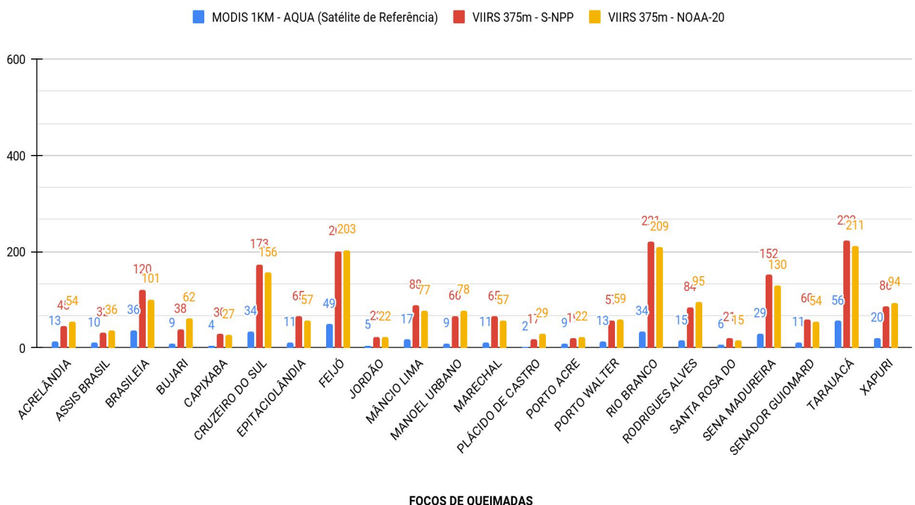
Figura 5 – Distribuição dos focos de queimadas acumulados de 01/01/2021 a 26/07/2021, no Estado do Acre. Satélite de referência AQUA (Barra de cor azul), VIIRS 375m/S-NPP (Cor vermelha) e VIIRS 375m/NOAA-20 (Cor amarela)
