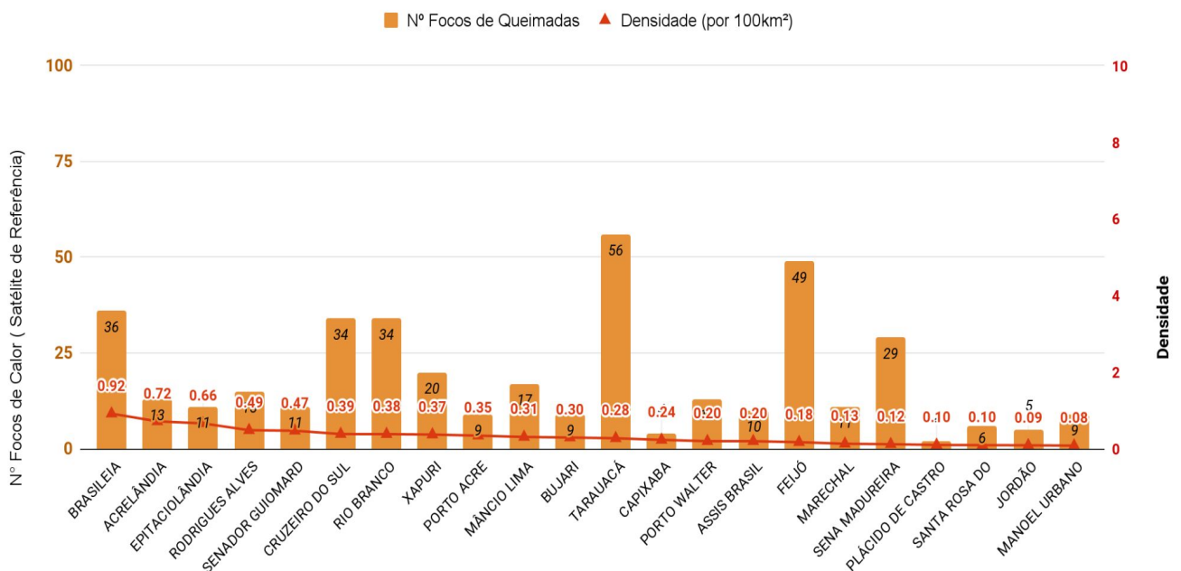
Figura 8 – Ocorrência de focos de queimadas e densidade por km 2 , por município em 01/01/2021 a 26/07/2021 (Satélite de referência AQUA)
