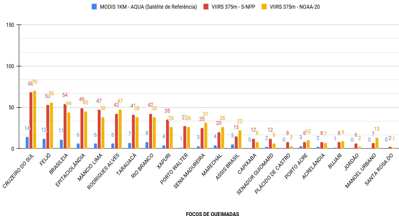
Figura 5 – Distribuição dos focos de queimadas acumulados de 01/01/2021 a 30/06/2021 , no Estado do Acre. Satélite de referência AQUA (Barra de cor azul), VIIRS 375m/S-NPP (Cor vermelha) e VIIRS 375m/NOAA-20 (Cor amarela)
