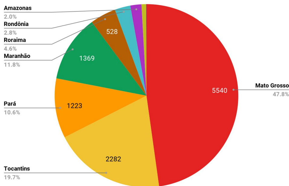
Figura 1 – Distribuição percentual dos focos de queimadas acumulados em 01/01/2021 a 30/06/2021 na Amazônia legal (Satélite de Referência AQUA Tarde)
