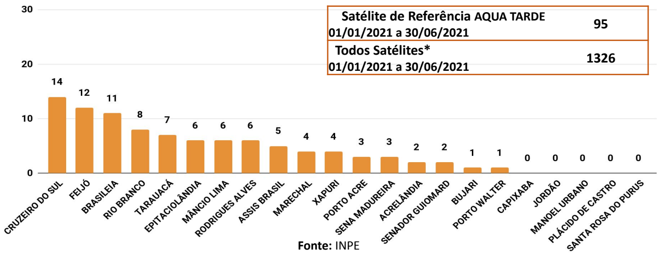
Figura 3 – Distribuição dos focos de queimadas acumulados de 01/01/2021 a 30/06/2021, no Estado do Acre. (Satélite de referência AQUA TARDE)
