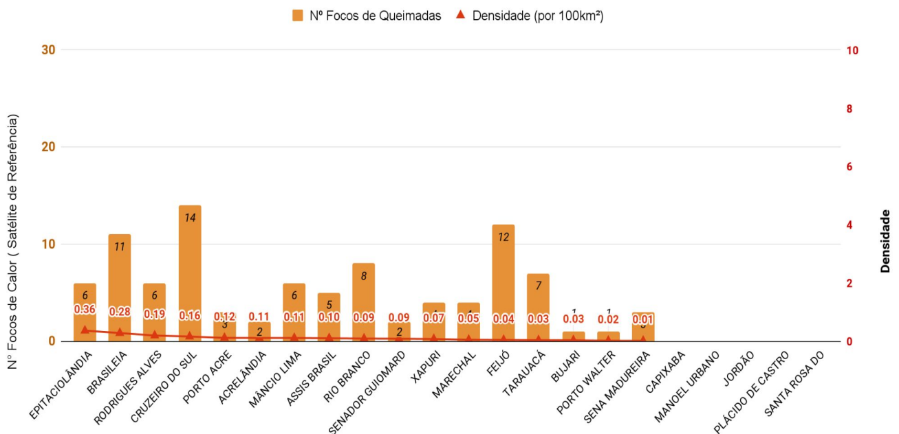
Figura 8 – Ocorrência de focos de queimadas e densidade por km 2 , por município em 01/01/2021 a 30/06/2021 (Satélite de referência AQUA)
