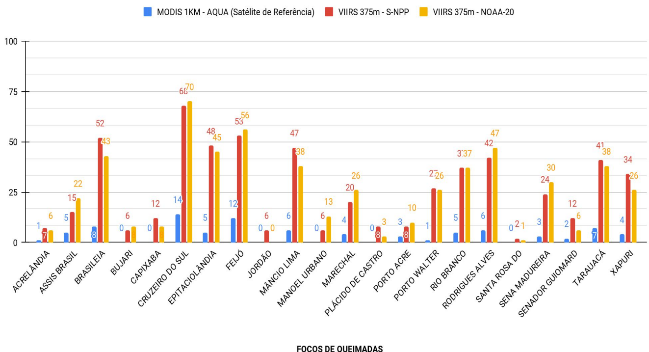
Figura 5 – Distribuição dos focos de queimadas acumulados de 01/01/2021 a 28/06/2021, no Estado do Acre. Satélite de referência AQUA (Barra de cor azul), VIIRS 375m/S-NPP (Cor vermelha) e VIIRS 375m/NOAA-20 (Cor amarela)
