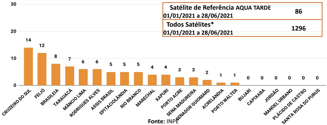
Figura 3 – Distribuição dos focos de queimadas acumulados de 01/01/2021 a 28/06/2021, no Estado do Acre. (Satélite de referência AQUA TARDE)
