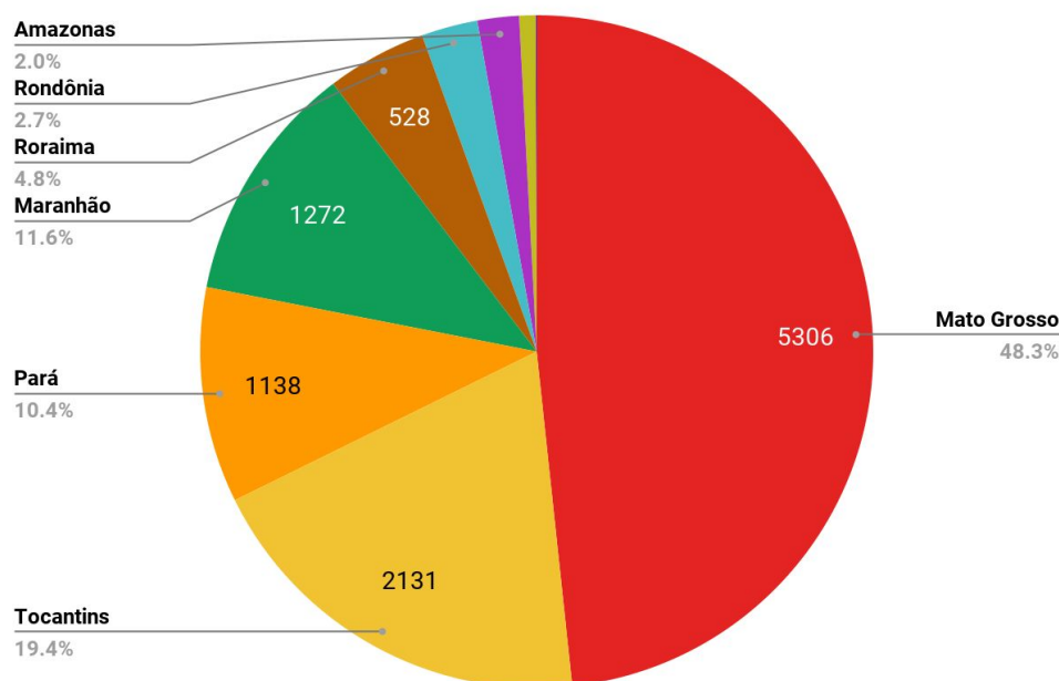
Figura 1 – Distribuição percentual dos focos de queimadas acumulados em 01/01/2021 a 28/06/2021 na Amazônia legal (Satélite de Referência AQUA Tarde)
