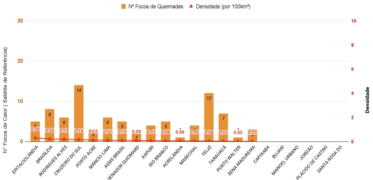
Figura 8 – Ocorrência de focos de queimadas e densidade por km 2 , por município em 01/01/2021 a 28/06/2021 (Satélite de referência AQUA)
