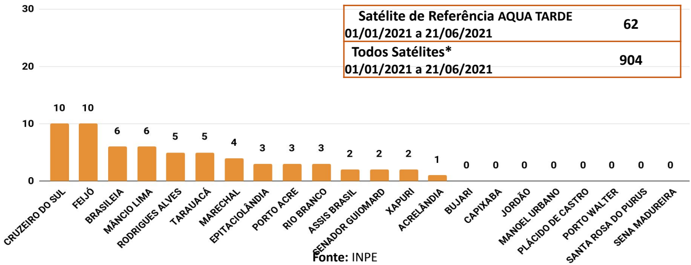
Figura 3 – Distribuição dos focos de queimadas acumulados de 01/01/2021 a 21/06/2021, no Estado do Acre. (Satélite de referência AQUA TARDE)
