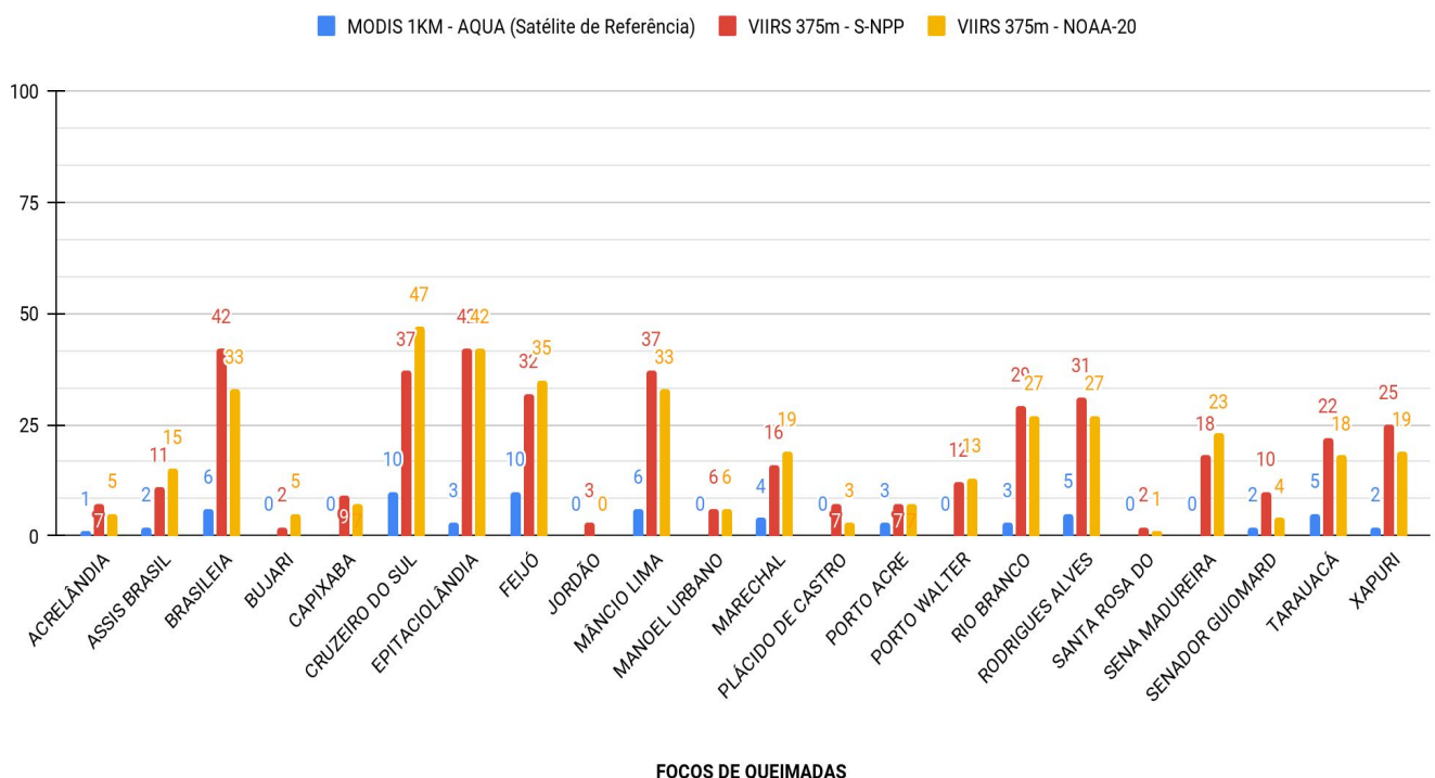
Figura 5 – Distribuição dos focos de queimadas acumulados de 01/01/2021 a 21/06/2021 , no Estado do Acre. Satélite de referência AQUA (Barra de cor azul), VIIRS 375m/S-NPP (Cor vermelha) e VIIRS 375m/NOAA-20 (Cor amarela)
