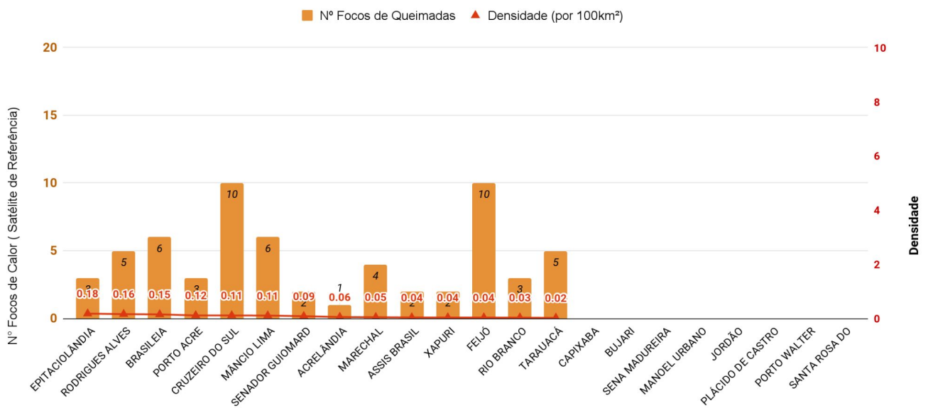
Figura 8 – Ocorrência de focos de queimadas e densidade por km 2 , por município em 01/01/2021 a 21/06/2021 (Satélite de referência AQUA)
