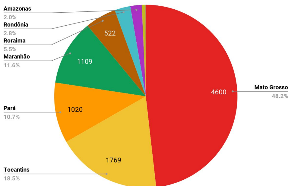
Figura 1 – Distribuição percentual dos focos de queimadas acumulados em 01/01/2021 a 21/06/2021 na Amazônia legal (Satélite de Referência AQUA Tarde)
