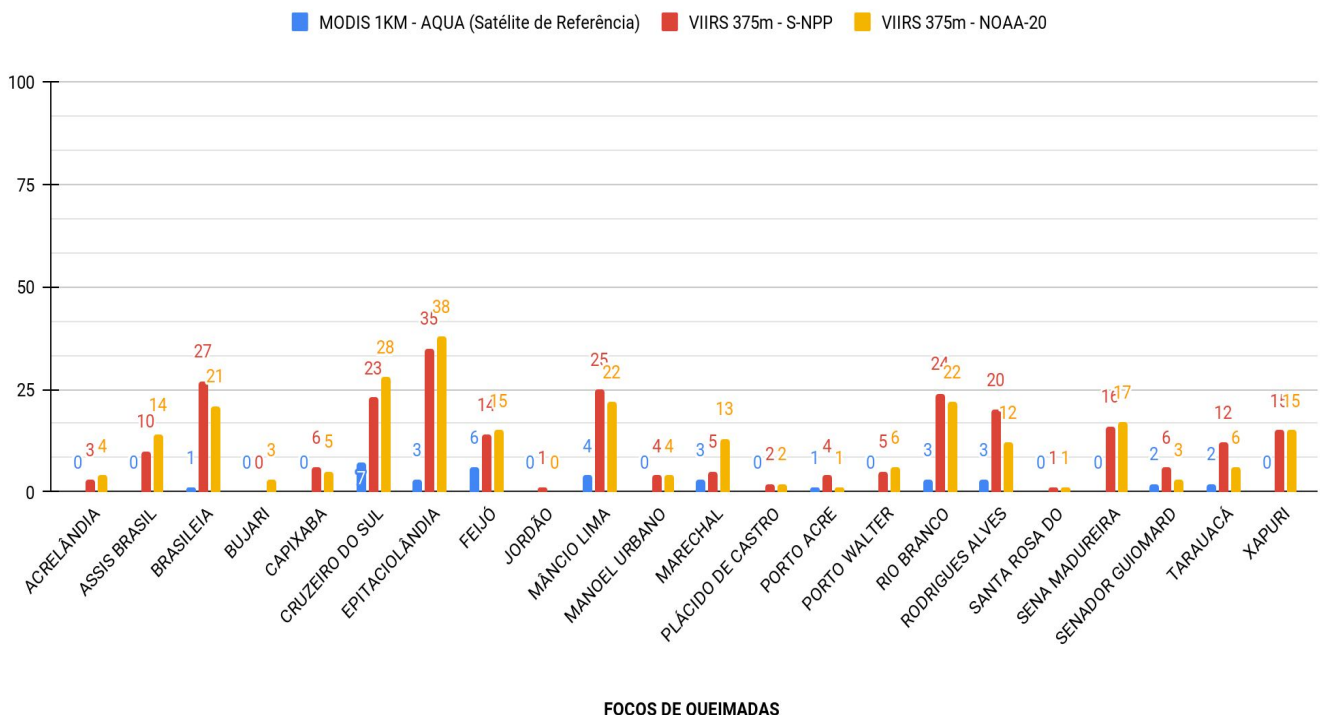
Figura 5 – Distribuição dos focos de queimadas acumulados de 01/01/2021 a 27/05/2021 , no Estado do Acre. Satélite de referência AQUA (Barra de cor azul), VIIRS 375m/S-NPP (Cor vermelha) e VIIRS 375m/NOAA-20 (Cor amarela)
