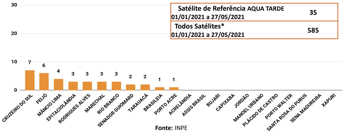
Figura 3 – Distribuição dos focos de queimadas acumulados de 01/01/2021 a 27/05/2021, no Estado do Acre. (Satélite de referência AQUA TARDE)
