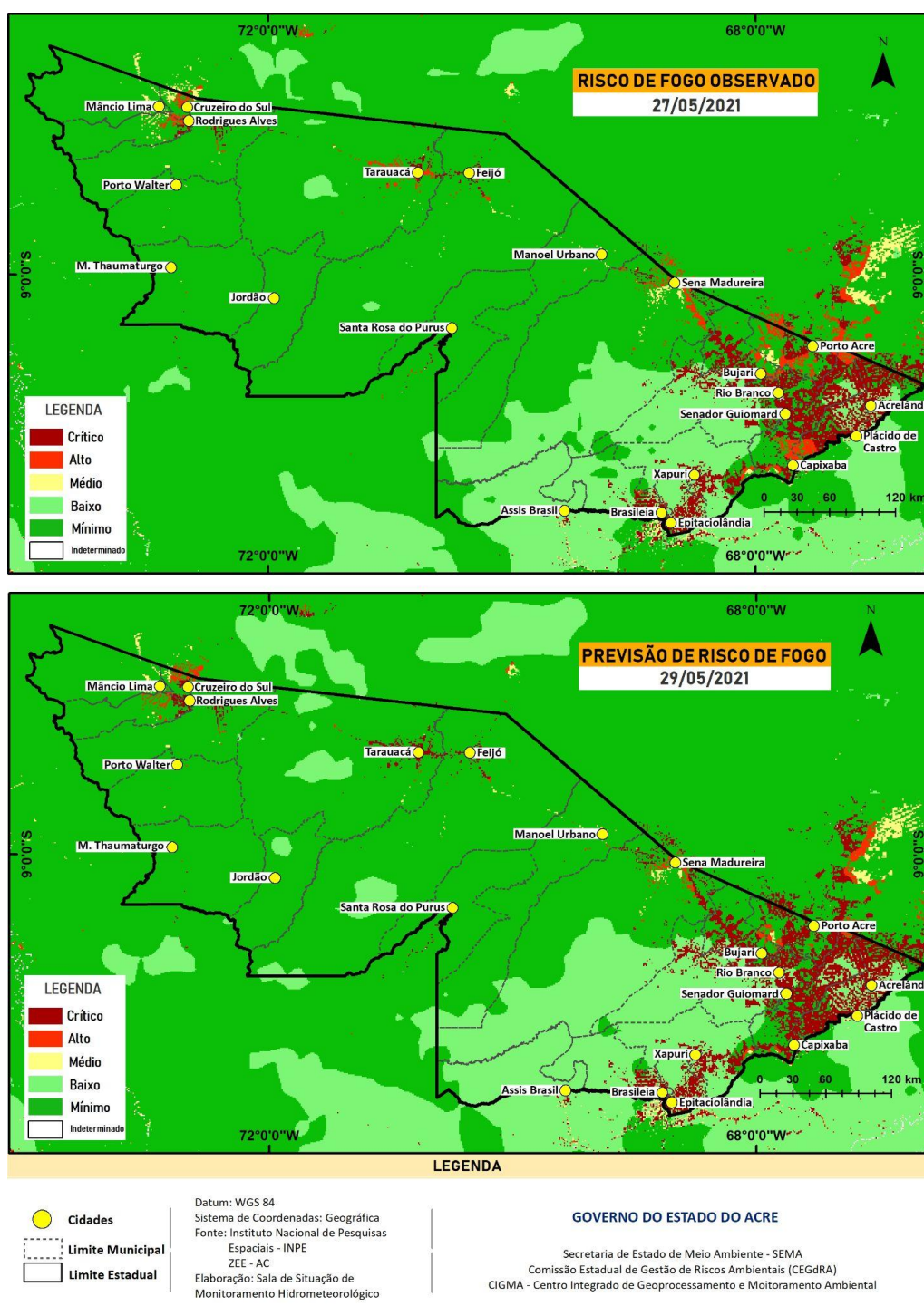
Figura 10 – Risco de Fogo observado no dia 28/05 e previsto para o estado do Acre para dia 29/05/2021
