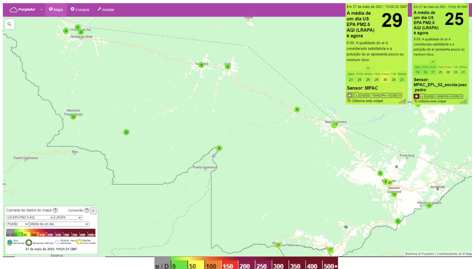
Figura 11 – Média do dia 27/05/2021 de Material Particulado PM 2,5 \mu\text{g}/\text{m}^3
