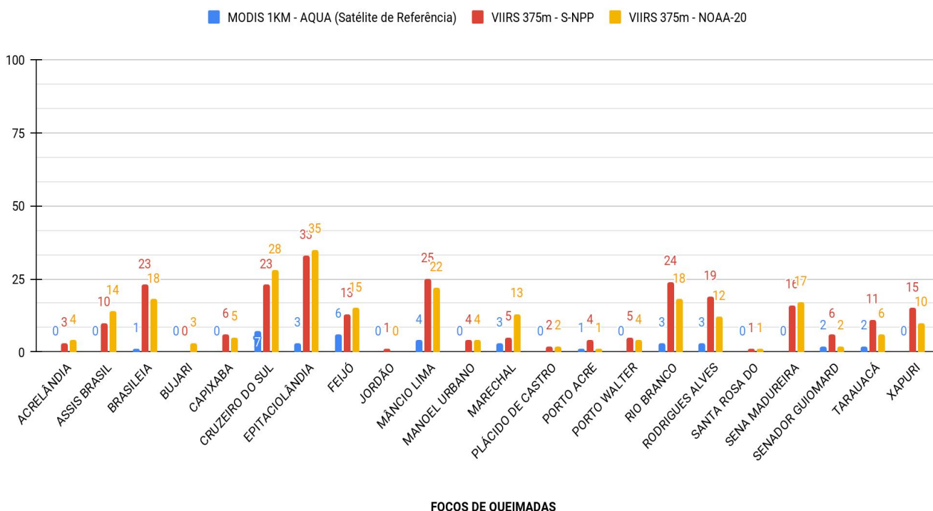
Figura 5 – Distribuição dos focos de queimadas acumulados de 01/01/2021 a 24/05/2021, no Estado do Acre. Satélite de referência AQUA (Barra de cor azul), VIIRS 375m/S-NPP (Cor vermelha) e VIIRS 375m/NOAA-20 (Cor amarela)
