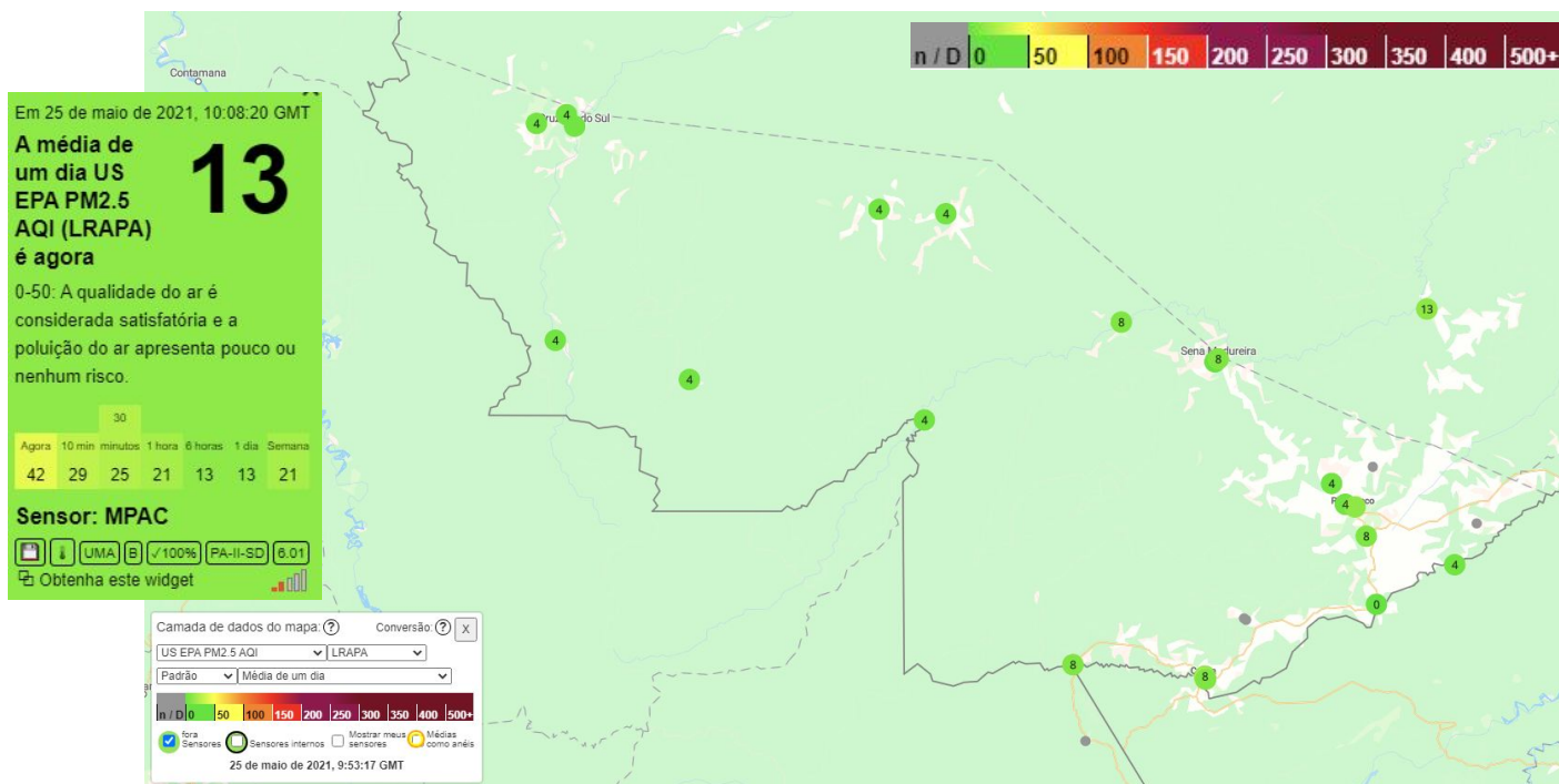
Figura 11 – Média do dia 25/05/2021 de Material Particulado PM 2,5 \mu\text{g}/\text{m}^3
