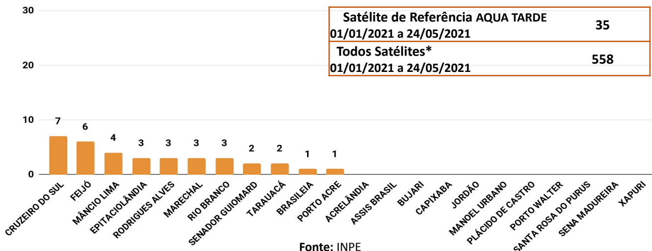
Figura 3 – Distribuição dos focos de queimadas acumulados de 01/01/2021 a 24/05/2021, no Estado do Acre. (Satélite de referência AQUA TARDE)
