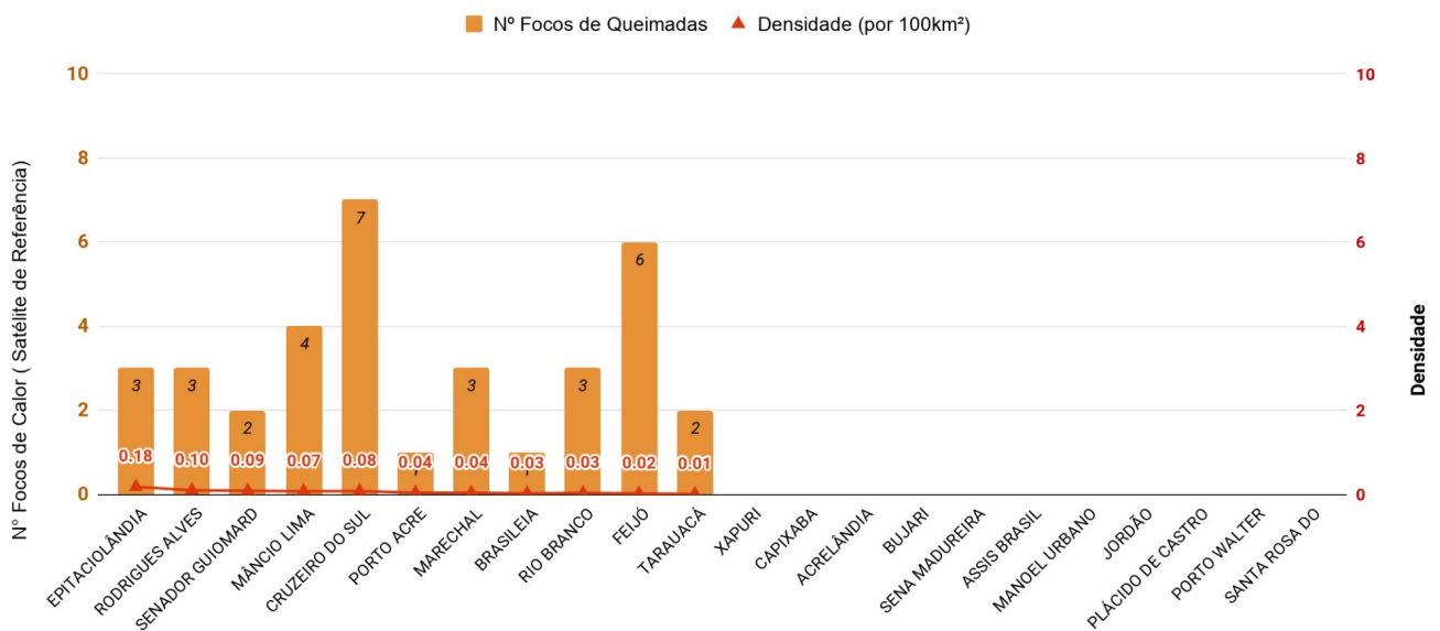
Figura 8 – Ocorrência de focos de queimadas e densidade por km 2 , por município em 01/01/2021 a 24/05/2021 (Satélite de referência AQUA)
