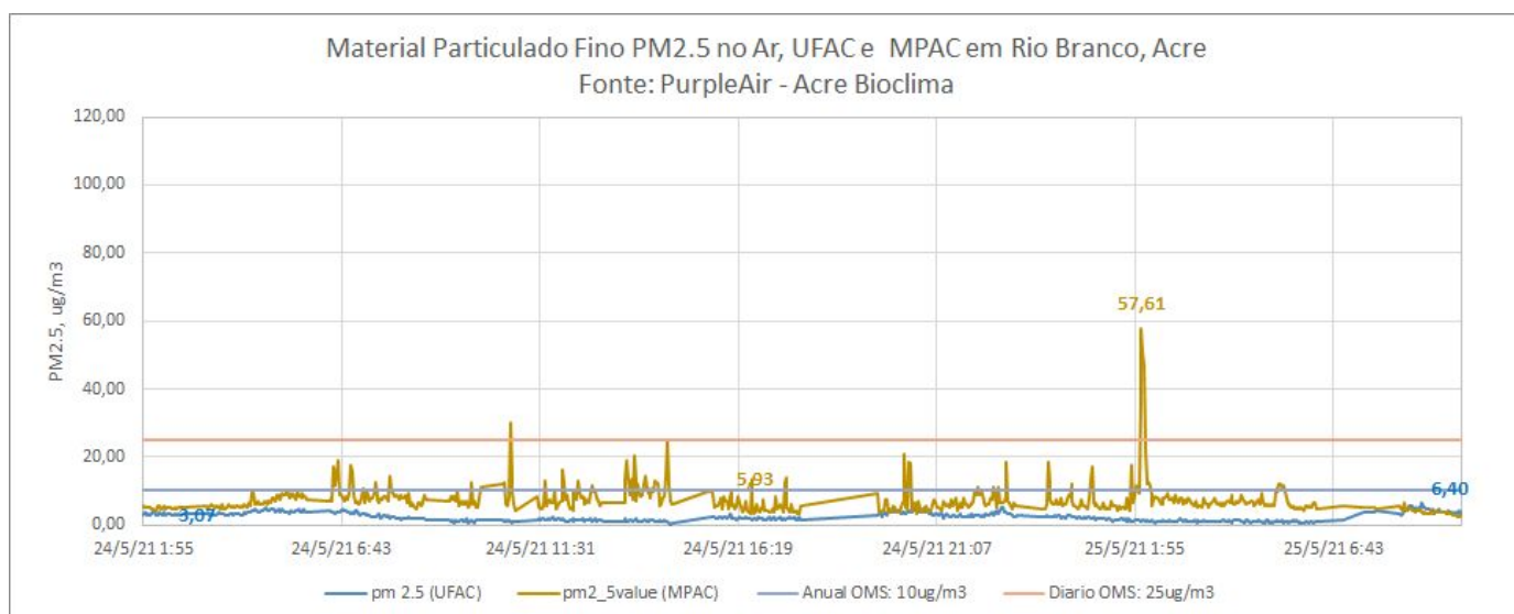
Figura 12 – Gráfico de material Particulado PM 2,5 \mu\text{g}/\text{m}^3
