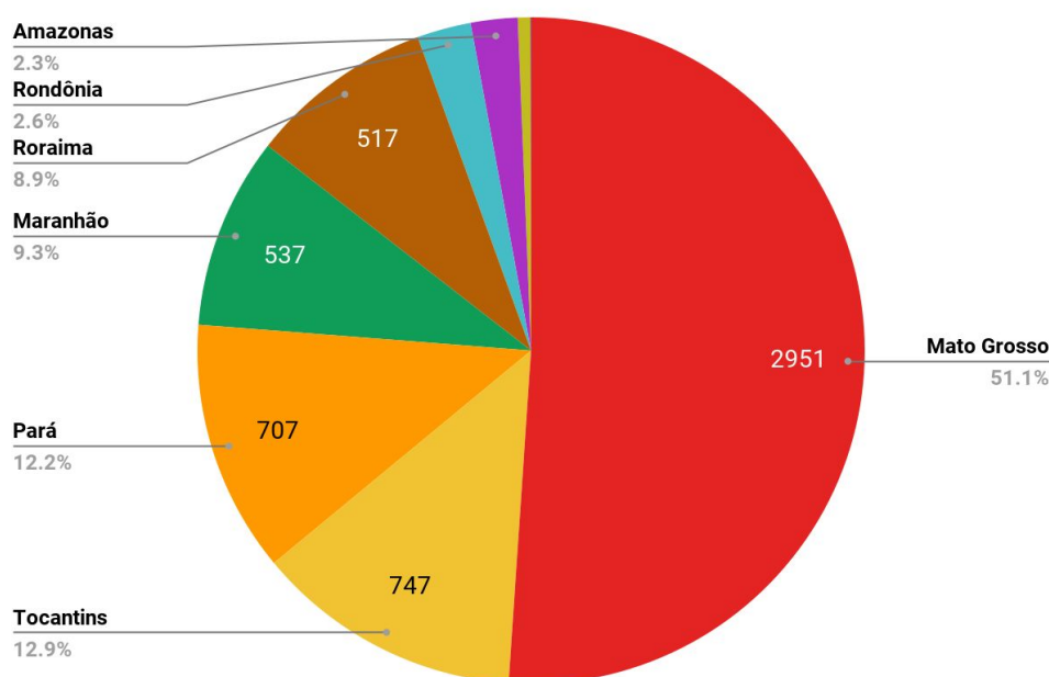
Figura 1 – Distribuição percentual dos focos de queimadas acumulados em 01/01/2021 a 24/05/2021 na Amazônia legal (Satélite de Referência AQUA Tarde)
