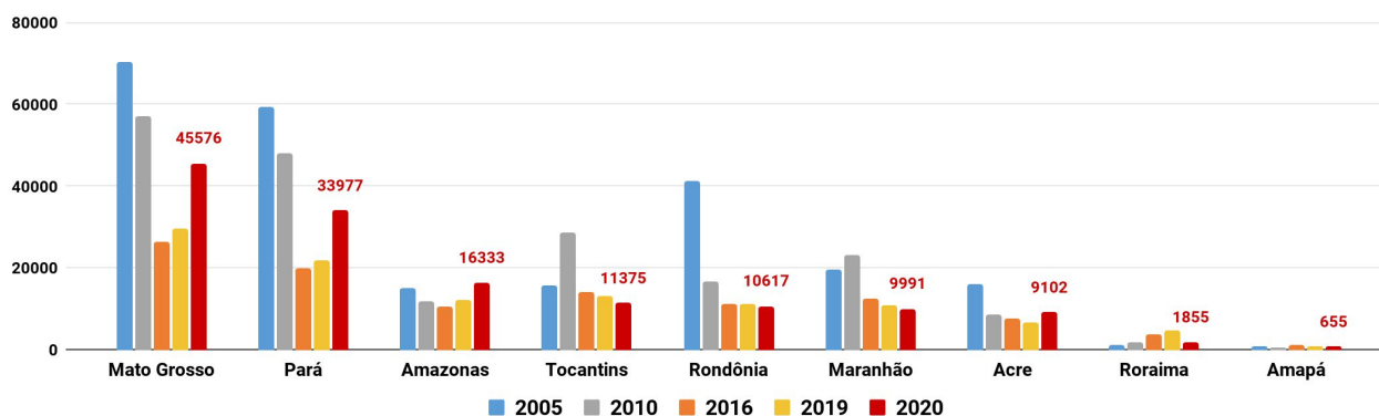
Figura 2 – Distribuição comparativa dos focos de queimadas acumulados de 01/01 a 04/11 na Amazônia legal, nos anos de 2005, 2010, 2016, 2019 e 2020 (Satélite de Referência AQUA Tarde)
