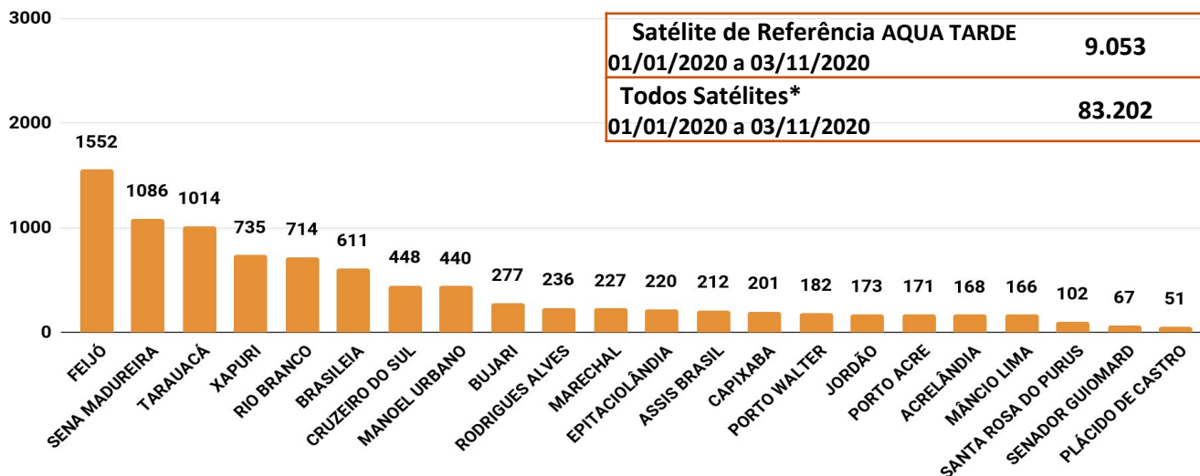
Figura 3 – Distribuição dos focos de queimadas acumulados de 01/01/2020 a 03/11/2020, no Estado do Acre. (Satélite de referência AQUA TARDE)
