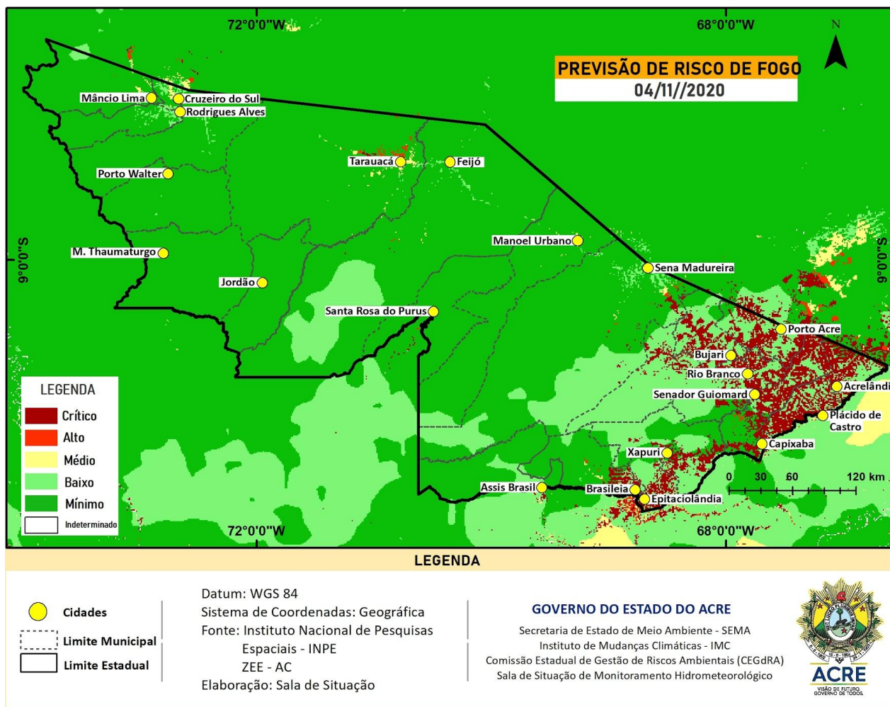
Figura 8 – Risco de Fogo para o estado do Acre em 04/11/2020
