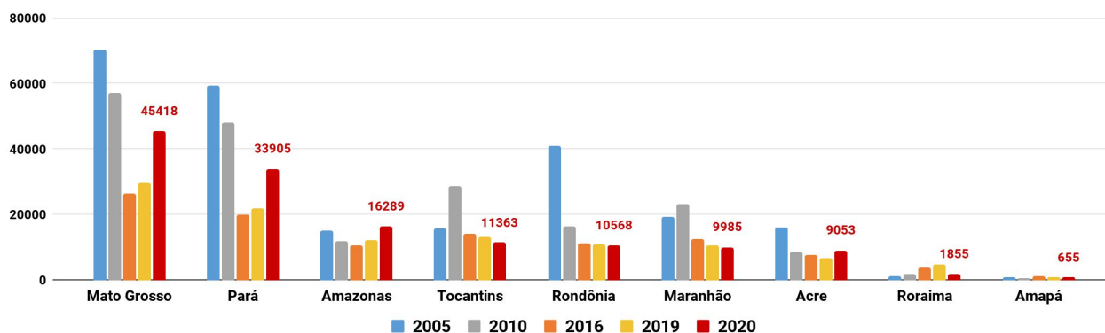
Figura 2 – Distribuição comparativa dos focos de queimadas acumulados de 01/01 a 03/11 na Amazônia legal, nos anos de 2005, 2010, 2016, 2019 e 2020 (Satélite de Referência AQUA Tarde)
