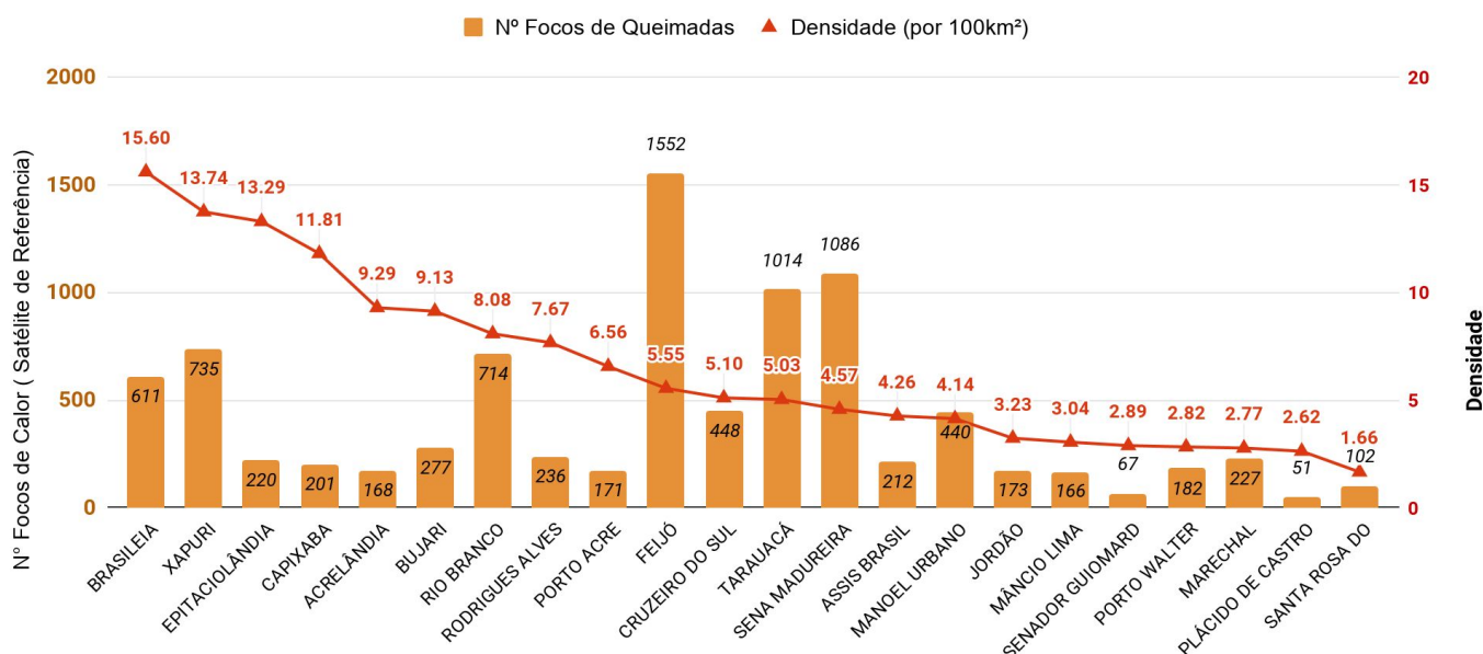
Figura 6 – Ocorrência de focos de queimadas e densidade por km 2 , por município em 01/01/2020 a 03/11/2020 (Satélite de referência AQUA TARDE)
