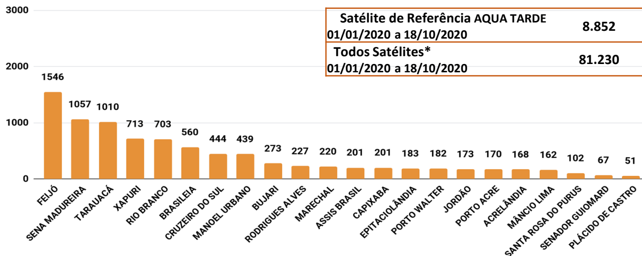
Figura 3 – Distribuição dos focos de queimadas acumulados de 01/01/2020 a 18/10/2020, no Estado do Acre. (Satélite de referência AQUA TARDE)
