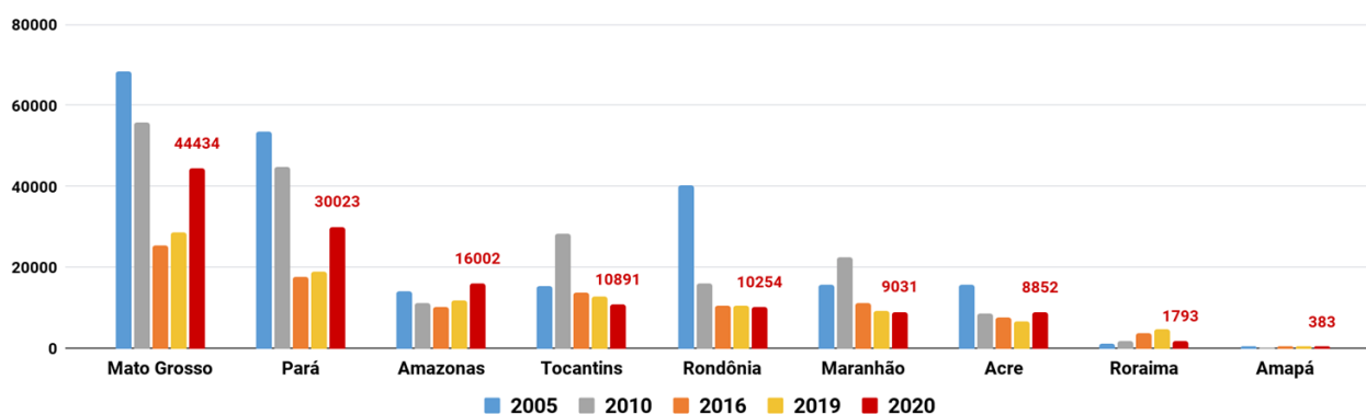
Figura 2 – Distribuição comparativa dos focos de queimadas acumulados de 01/01 a 18/10 na Amazônia legal, nos anos de 2005, 2010, 2016, 2019 e 2020 (Satélite de Referência AQUA Tarde)
