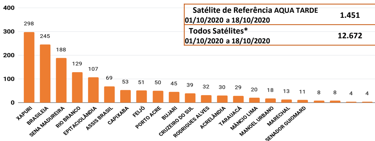
Figura 4 – Distribuição dos focos de queimadas acumulados de 01/10/2020 a 18/10/2020, no Estado do Acre. (Satélite de referência AQUA TARDE)
