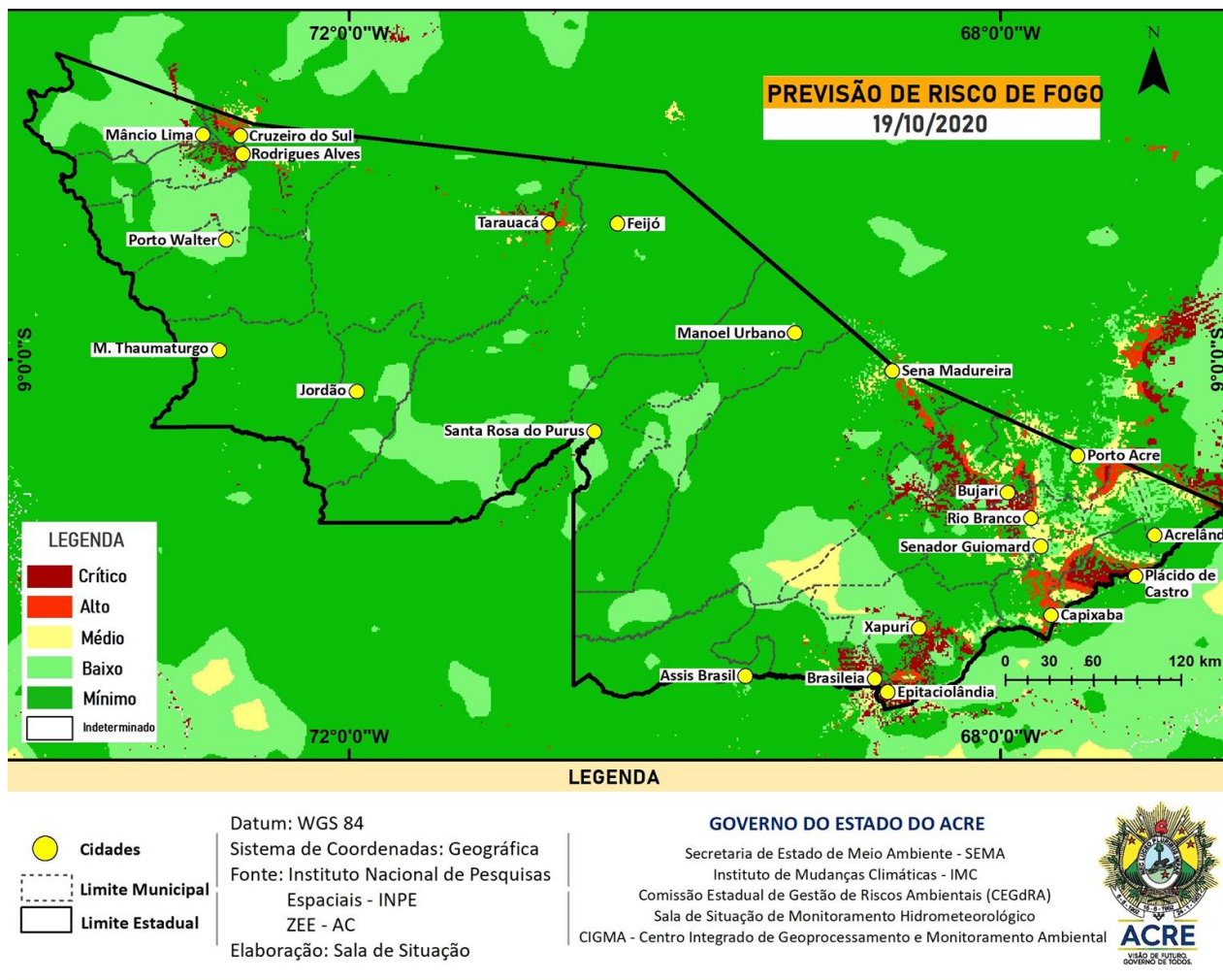
Figura 8 – Risco de Fogo para o estado do Acre em 19/10/2020
