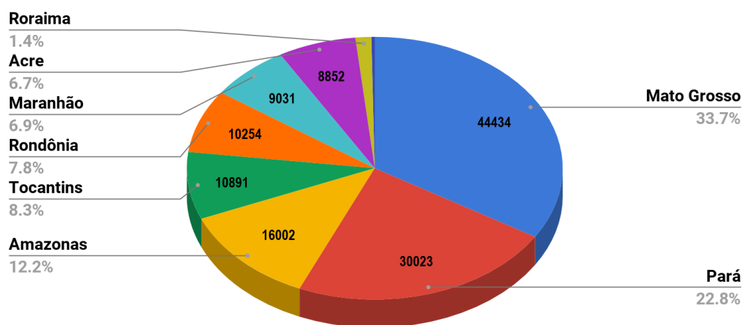
Figura 1 – Distribuição percentual dos focos de queimadas acumulados em 01/01/2020 a 18/10/2020 na Amazônia legal (Satélite de Referência AQUA Tarde)
