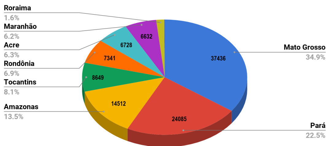
Figura 1 – Distribuição percentual dos focos de queimadas acumulados em 01/01/2020 a 21/09/2020 na Amazônia legal (Satélite de Referência AQUA Tarde)
