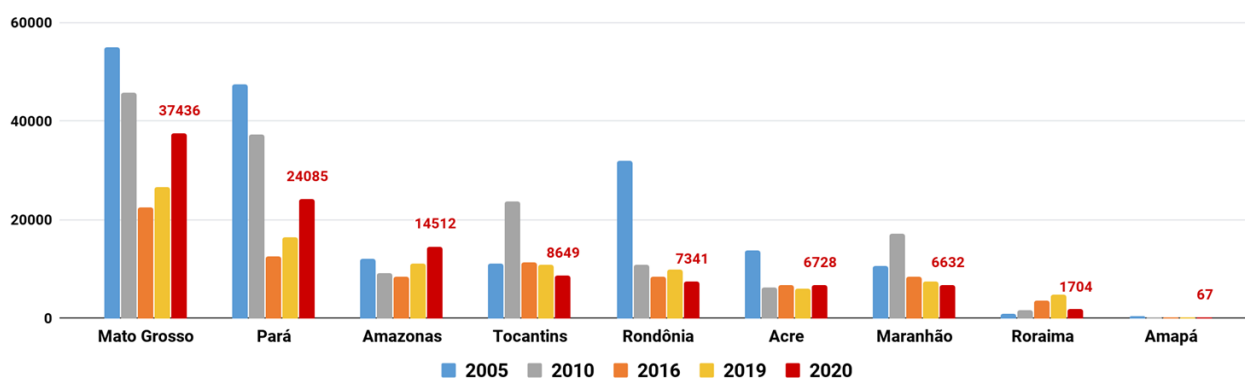
Figura 2 – Distribuição comparativa dos focos de queimadas acumulados de 01/01 a 21/09 na Amazônia legal, nos anos de 2005, 2010, 2016, 2019 e 2020 (Satélite de Referência AQUA Tarde)
