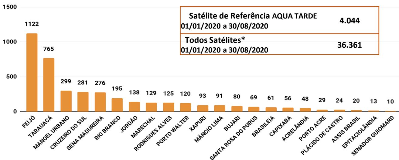
Figura 3 – Distribuição dos focos de queimadas acumulados de 01/01/2020 a 30/08/2020 , no Estado do Acre. (Satélite de referência AQUA TARDE)
