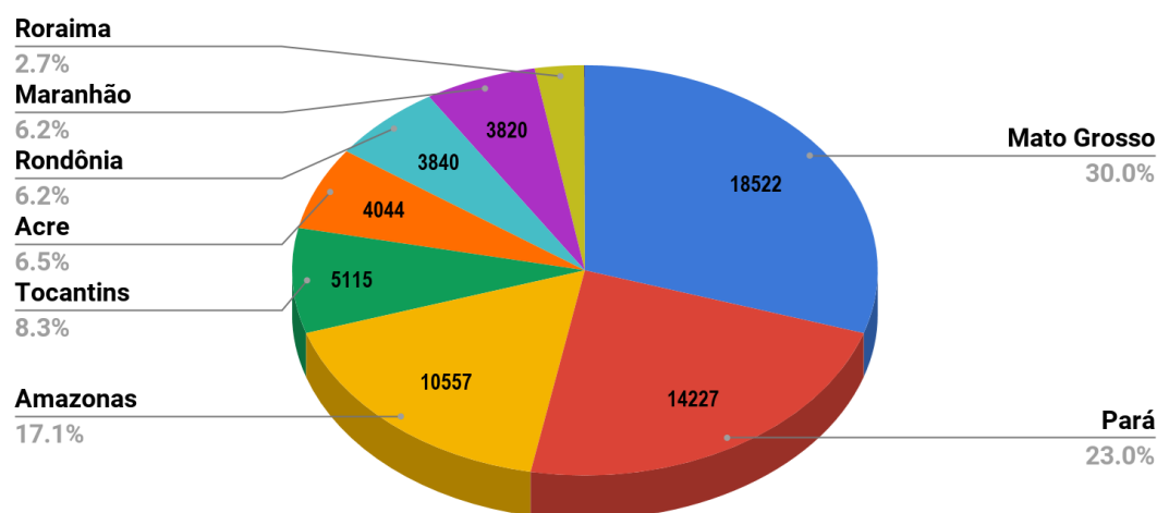
Figura 1 – Distribuição percentual dos focos de queimadas acumulados em 01/01/2020 a 30/08/2020 na Amazônia legal (Satélite de Referência AQUA Tarde)
