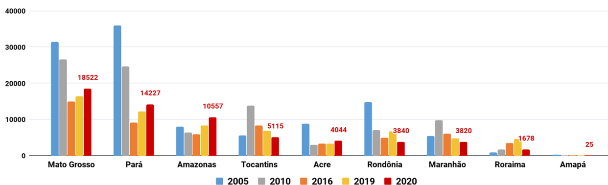
Figura 2 – Distribuição comparativa dos focos de queimadas acumulados de 01/01 a 30/08 na Amazônia legal, nos anos de 2005, 2010, 2016, 2019 e 2020 (Satélite de Referência AQUA Tarde)
