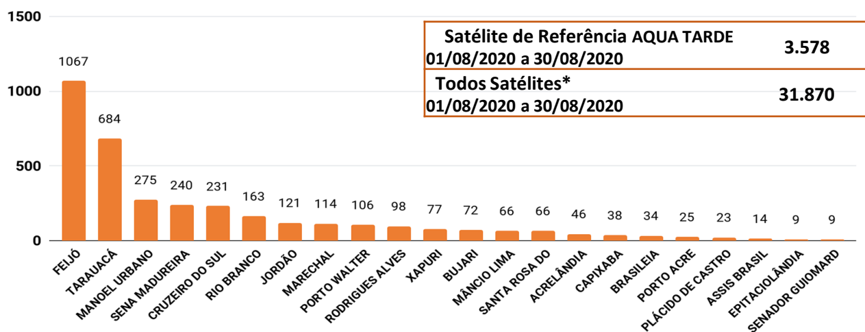
Figura 4 – Distribuição dos focos de queimadas acumulados de 01/08/2020 a 30/08/2020 , no Estado do Acre. (Satélite de referência AQUA TARDE)
