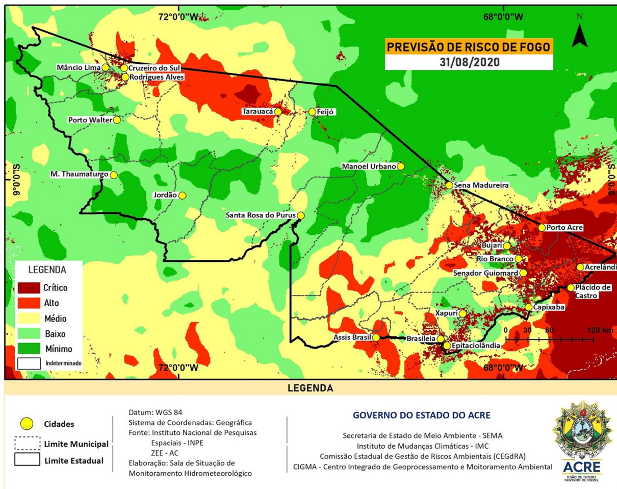
Figura 8 – Risco de Fogo para o estado do Acre em 31/08/2020
