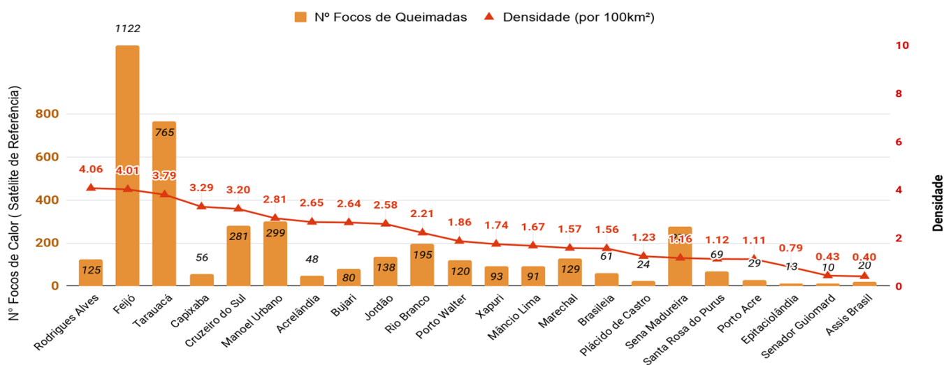
Figura 6 – Ocorrência de focos de queimadas e densidade por km 2 , por município em 01/01/2020 a 30/08/2020 (Satélite de referência AQUA TARDE)
