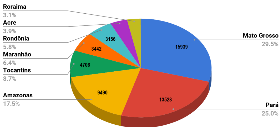
Figura 1 – Distribuição percentual dos focos de queimadas acumulados em 01/01/2020 a 24/08/2020 na Amazônia legal (Satélite de Referência AQUA Tarde)
