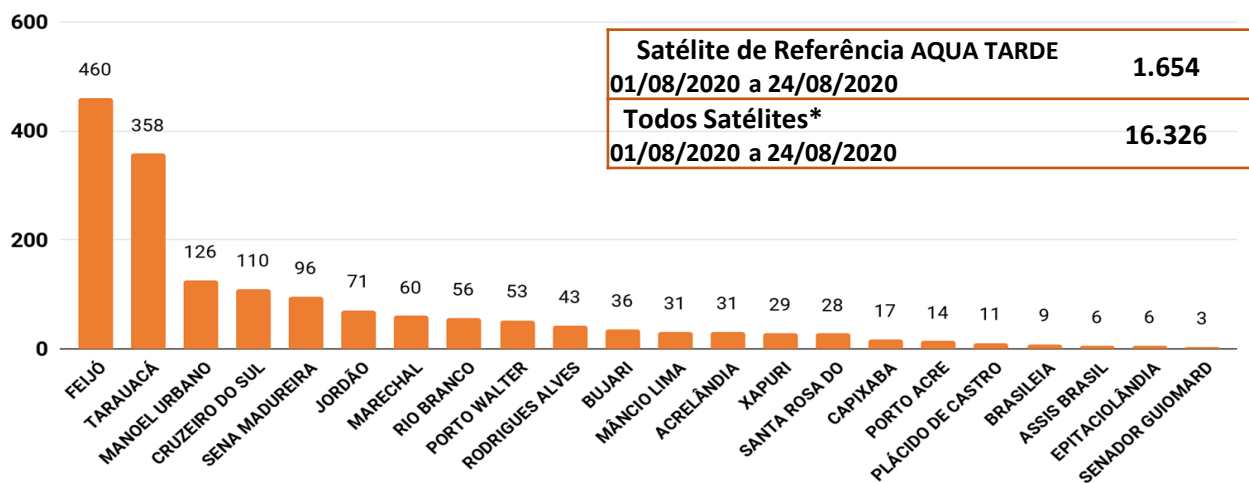
Figura 4 – Distribuição dos focos de queimadas acumulados de 01/08/2020 a 24/08/2020, no Estado do Acre. (Satélite de referência AQUA TARDE)
