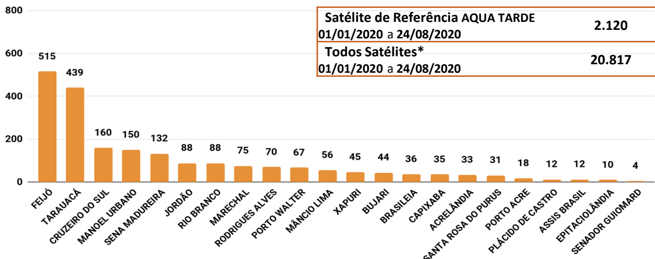
Figura 3 – Distribuição dos focos de queimadas acumulados de 01/01/2020 a 24/08/2020, no Estado do Acre. (Satélite de referência AQUA TARDE)
