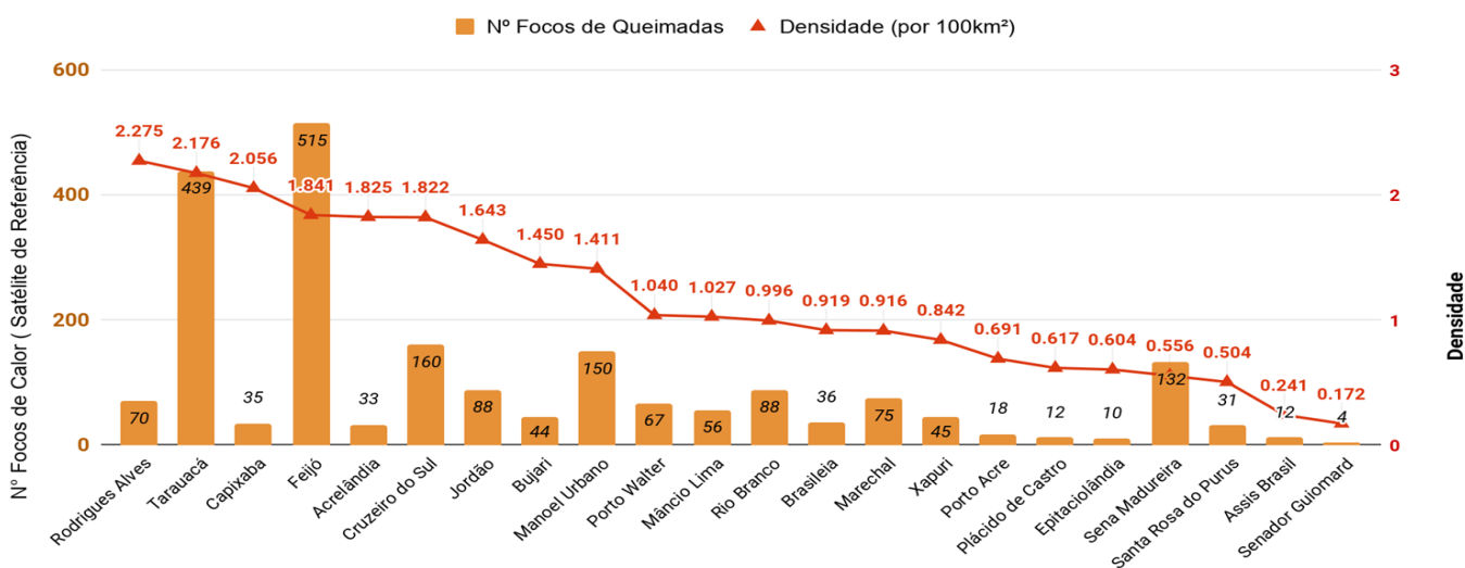
Figura 6 – Ocorrência de focos de queimadas e densidade por km 2 , por município em 01/01/2020 a 24/08/2020 (Satélite de referência AQUA TARDE)
