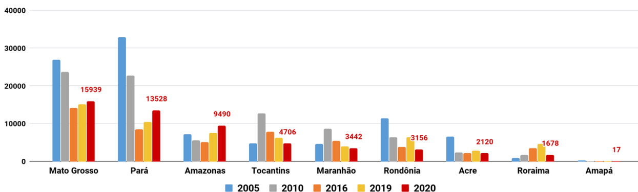
Figura 2 – Distribuição comparativa dos focos de queimadas acumulados de 01/01 a 24/08 na Amazônia legal, nos anos de 2005, 2010, 2016, 2019 e 2020 (Satélite de Referência AQUA Tarde)
