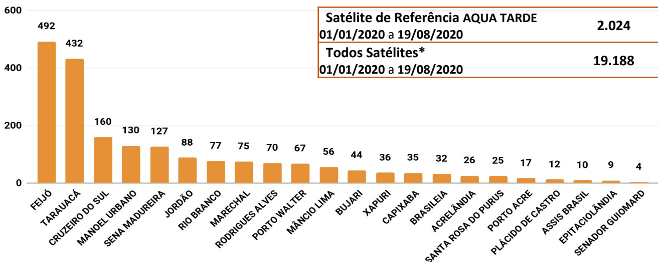
Figura 3 – Distribuição dos focos de queimadas acumulados de 01/01/2020 a 19/08/2020, no Estado do Acre. (Satélite de referência AQUA TARDE)
