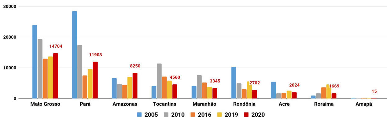
Figura 2 – Distribuição comparativa dos focos de queimadas acumulados de 01/01 a 19/08 na Amazônia legal, nos anos de 2005, 2010, 2016, 2019 e 2020 (Satélite de Referência AQUA Tarde)
