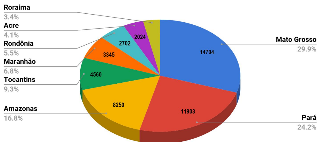
Figura 1 – Distribuição percentual dos focos de queimadas acumulados em 01/01/2020 a 19/08/2020 na Amazônia legal (Satélite de Referência AQUA Tarde)
