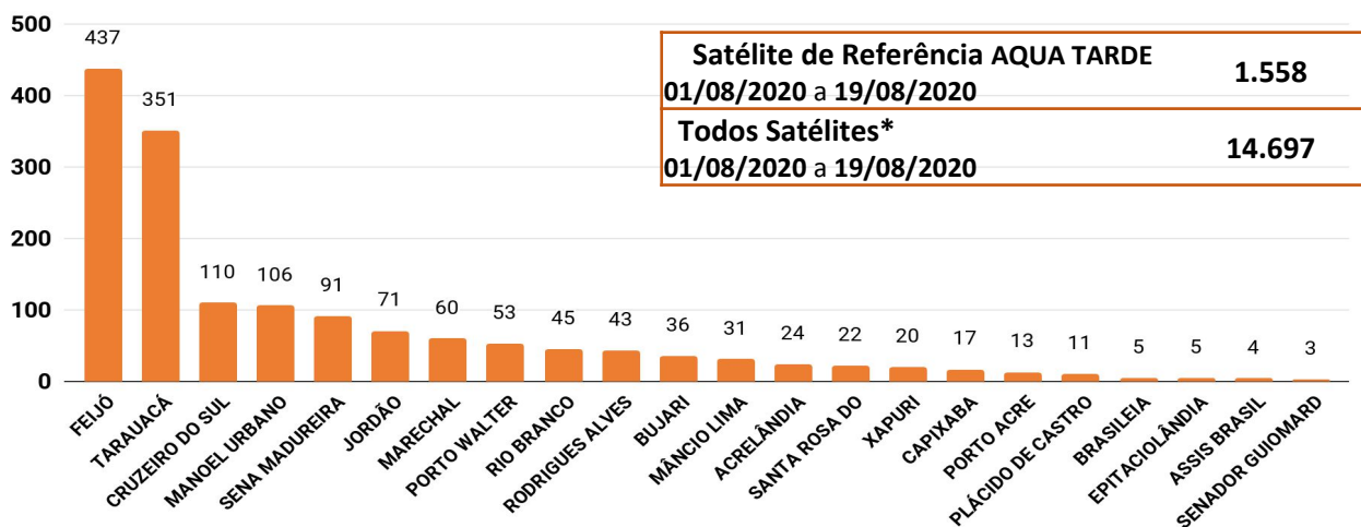
Figura 4 – Distribuição dos focos de queimadas acumulados de 01/08/2020 a 19/08/2020, no Estado do Acre. (Satélite de referência AQUA TARDE)
