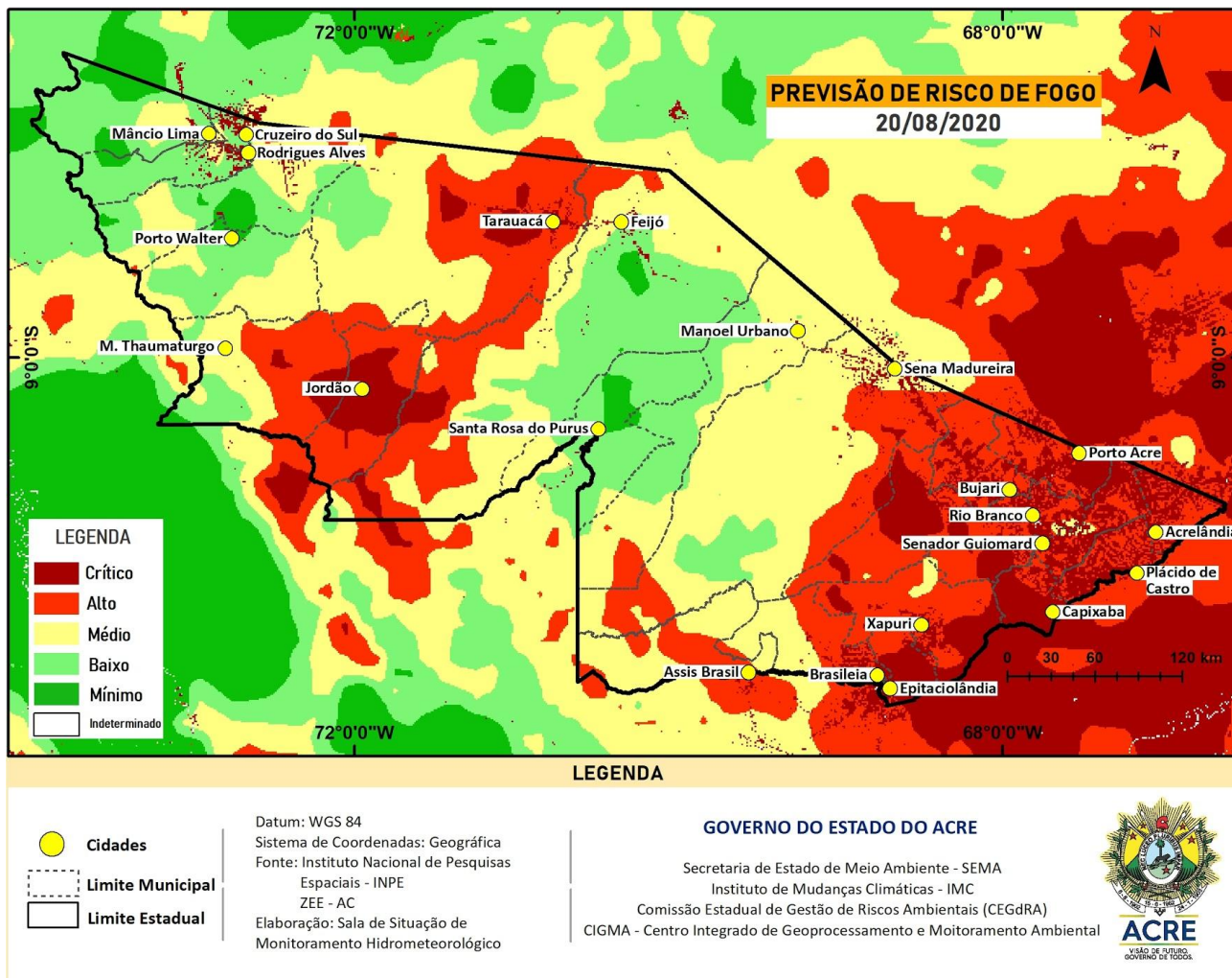
Figura 8 – Risco de Fogo para o estado do Acre em 20/08/2020
