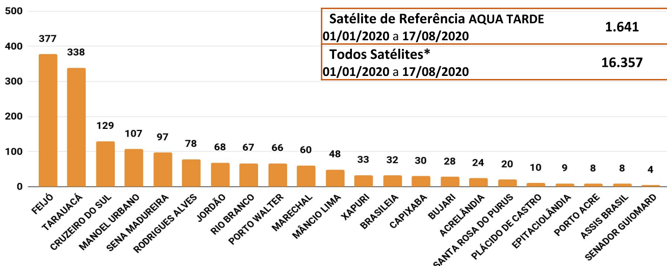
Figura 3 – Distribuição dos focos de queimadas acumulados de 01/01/2020 a 17/08/2020, no Estado do Acre. (Satélite de referência AQUA TARDE)
