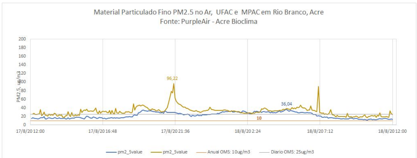
Figura 9 – Gráfico de material Particulado PM 2,5 \mu\text{g}/\text{m}^3
