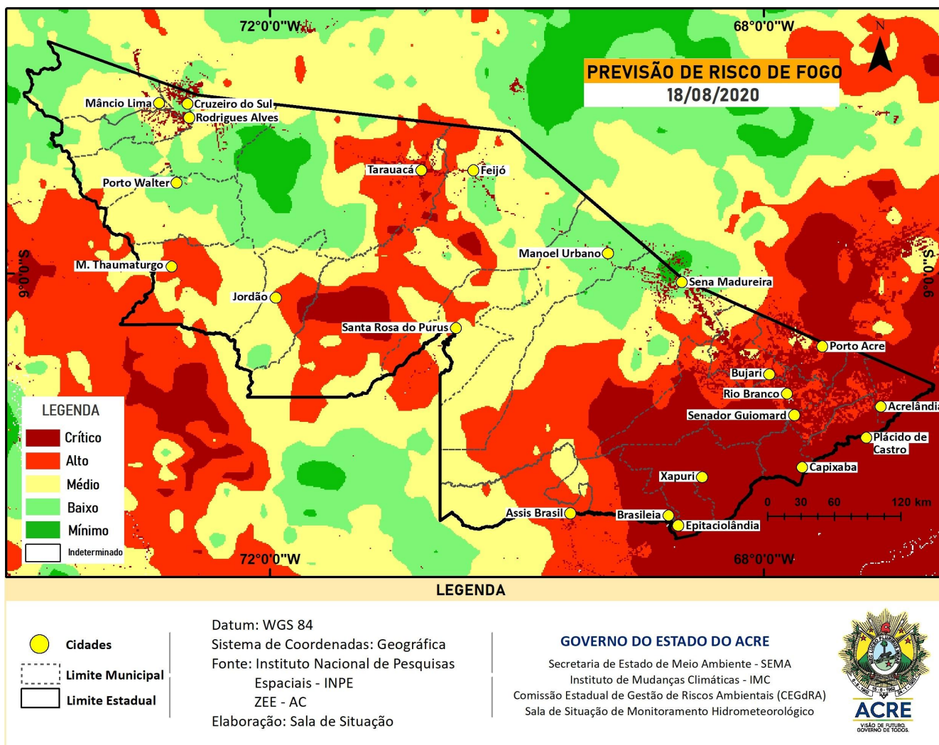
Figura 8 – Risco de Fogo para o estado do Acre em 18/08/2020
