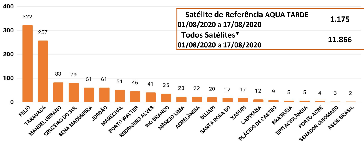
Figura 4 – Distribuição dos focos de queimadas acumulados de 01/08/2020 a 17/08/2020, no Estado do Acre. (Satélite de referência AQUA TARDE)
