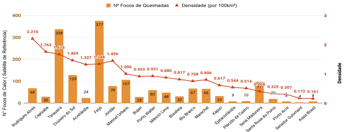
Figura 6 – Ocorrência de focos de queimadas e densidade por km 2 , por município em 01/01/2020 a 17/08/2020 (Satélite de referência AQUA TARDE)
