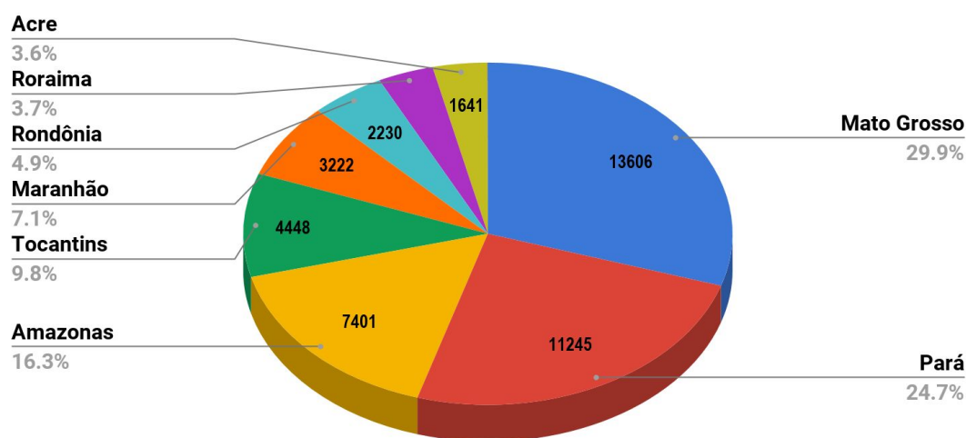
Figura 1 – Distribuição percentual dos focos de queimadas acumulados em 01/01/2020 a 17/08/2020 na Amazônia legal (Satélite de Referência AQUA Tarde)
