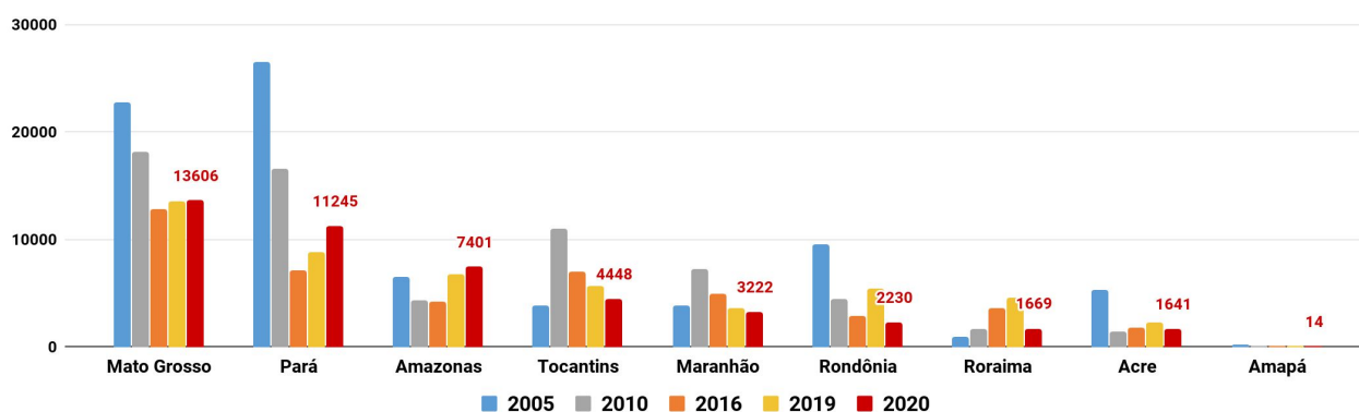
Figura 2 – Distribuição comparativa dos focos de queimadas acumulados de 01/01 a 17/08 na Amazônia legal, nos anos de 2005, 2010, 2016, 2019 e 2020 (Satélite de Referência AQUA Tarde)
