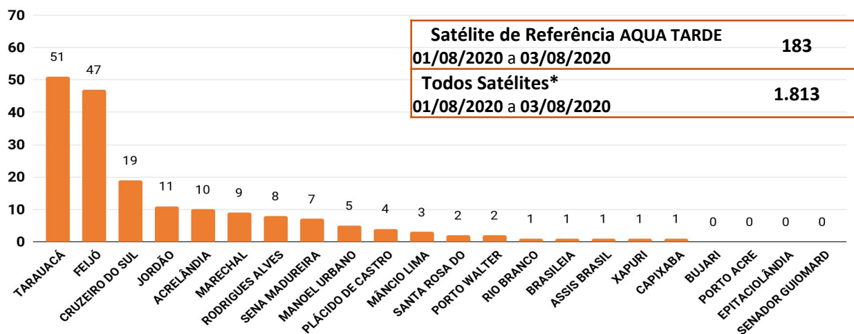
Figura 4 – Distribuição dos focos de queimadas acumulados de 01/08/2020 a 03/08/2020, no Estado do Acre. (Satélite de referência AQUA TARDE)
