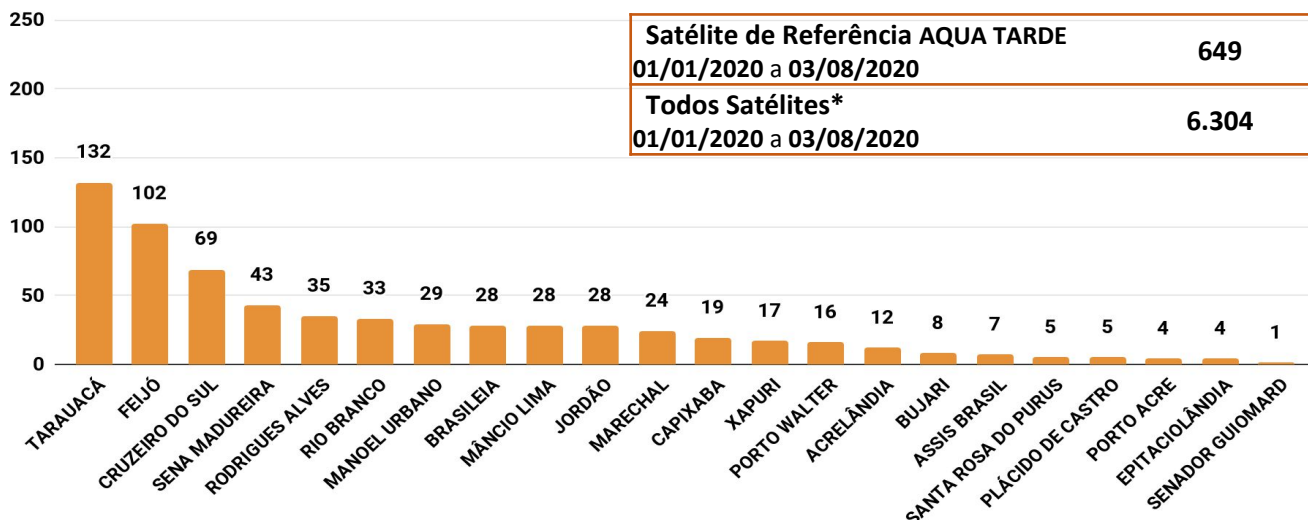
Figura 3 – Distribuição dos focos de queimadas acumulados de 01/01/2020 a 03/08/2020, no Estado do Acre. (Satélite de referência AQUA TARDE)
