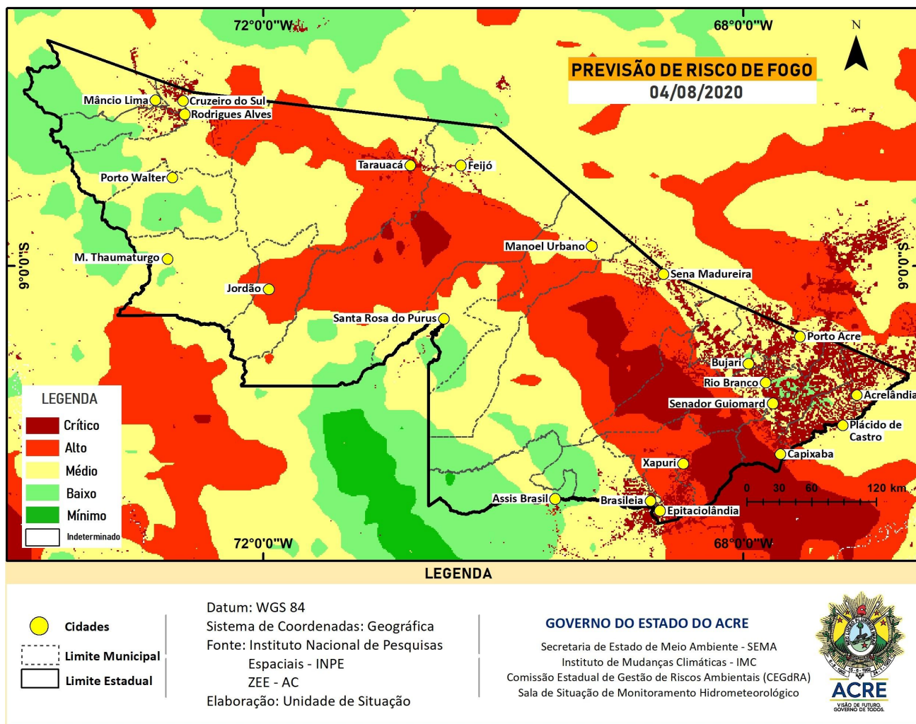
Figura 8 – Risco de Fogo para o estado do Acre em 04/08/2020
