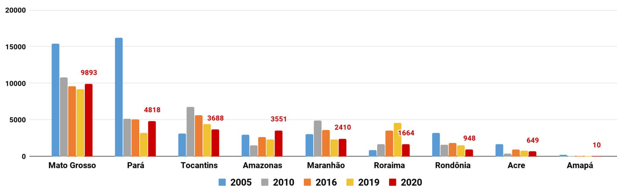
Figura 2 – Distribuição comparativa dos focos de queimadas acumulados de 01/01 a 03/08 na Amazônia legal, nos anos de 2005, 2010, 2016, 2019 e 2020 (Satélite de Referência AQUA Tarde)
