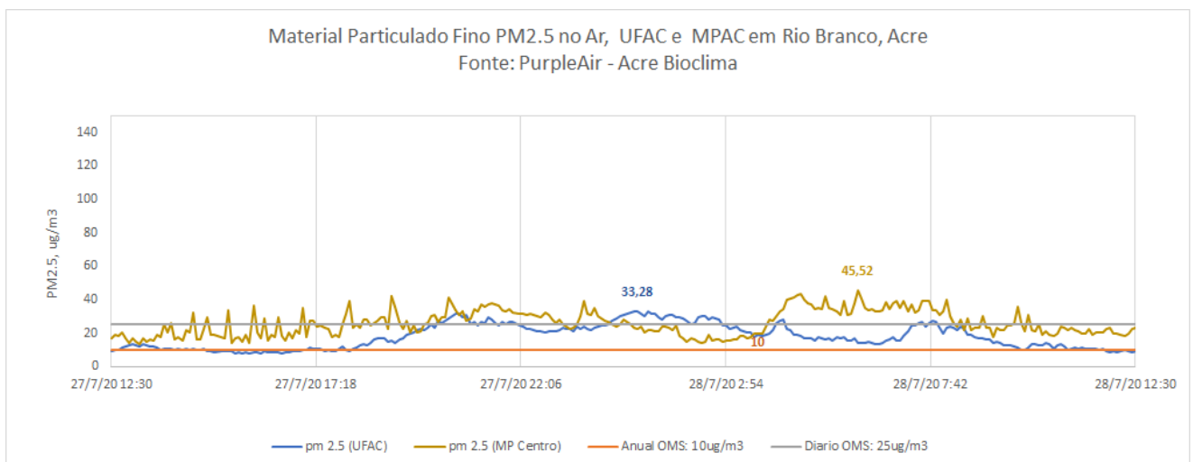
Figura 9 – Gráfico de material Particulado PM 2,5 \mu\text{g}/\text{m}^3
