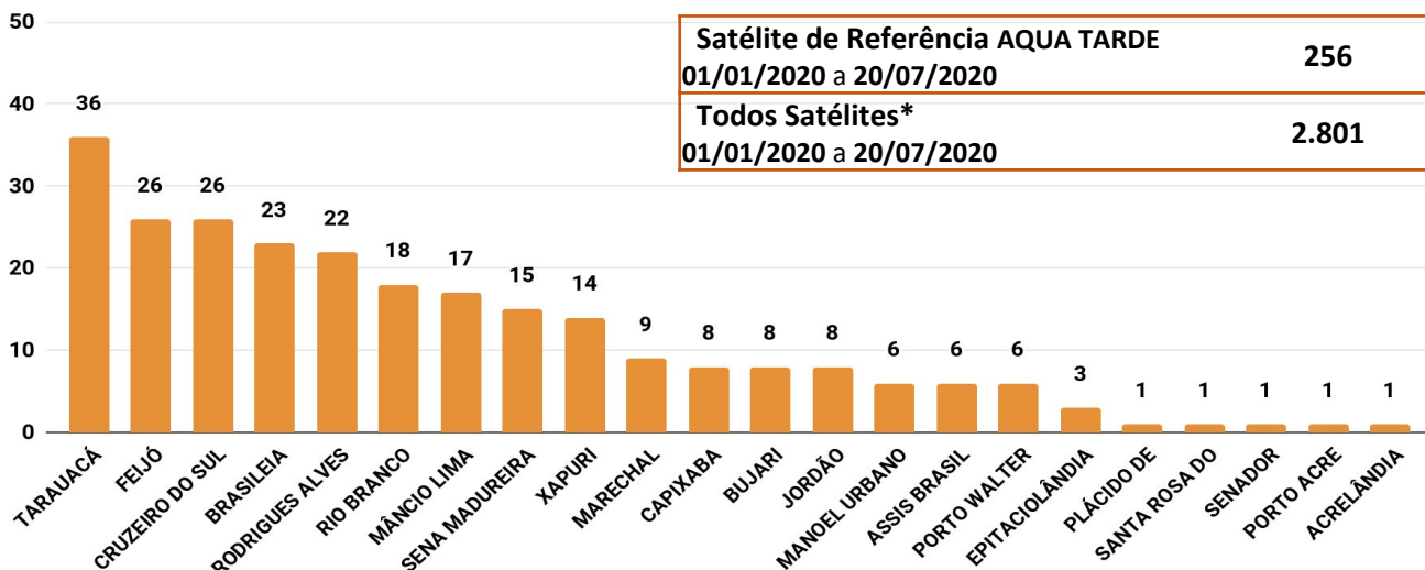
Figura 3 – Distribuição dos focos de queimadas acumulados de 01/01/2020 a 20/07/2020, no Estado do Acre. (Satélite de referência AQUA TARDE)
