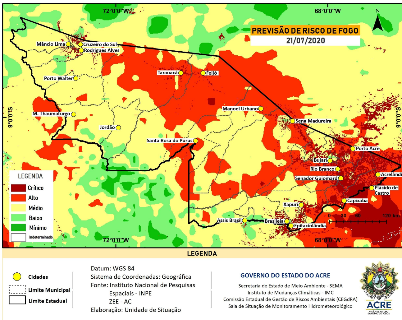
Figura 8 – Risco de Fogo para o estado do Acre em 21/07/2020
