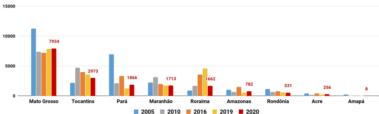
Figura 2 – Distribuição comparativa dos focos de queimadas acumulados de 01/01 a 20/07 na Amazônia legal, nos anos de 2005, 2010, 2016, 2019 e 2020 (Satélite de Referência AQUA Tarde)
