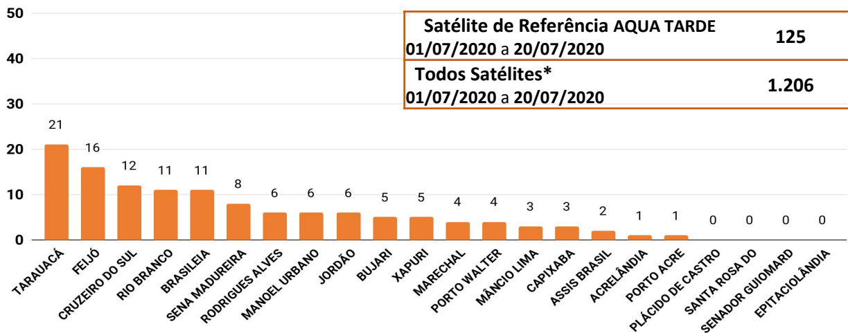
Figura 4 – Distribuição dos focos de queimadas acumulados de 01/07/2020 a 20/07/2020, no Estado do Acre. (Satélite de referência AQUA TARDE)
