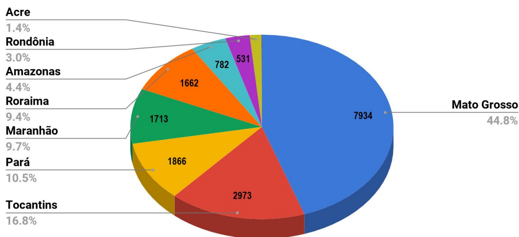
Figura 1 – Distribuição percentual dos focos de queimadas acumulados em 01/01/2020 a 20/07/2020 na Amazônia legal (Satélite de Referência AQUA Tarde)
