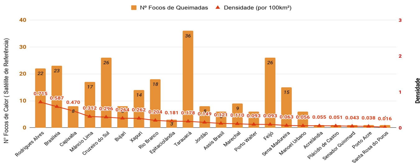
Figura 6 – Ocorrência de focos de queimadas e densidade por km 2 , por município em 01/01/2020 a 20/07/2020 (Satélite de referência AQUA TARDE)
