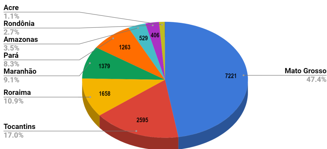
Figura 1 – Distribuição percentual dos focos de queimadas acumulados em 01/01/2020 a 09/07/2020 na Amazônia legal (Satélite de Referência AQUA Tarde)
