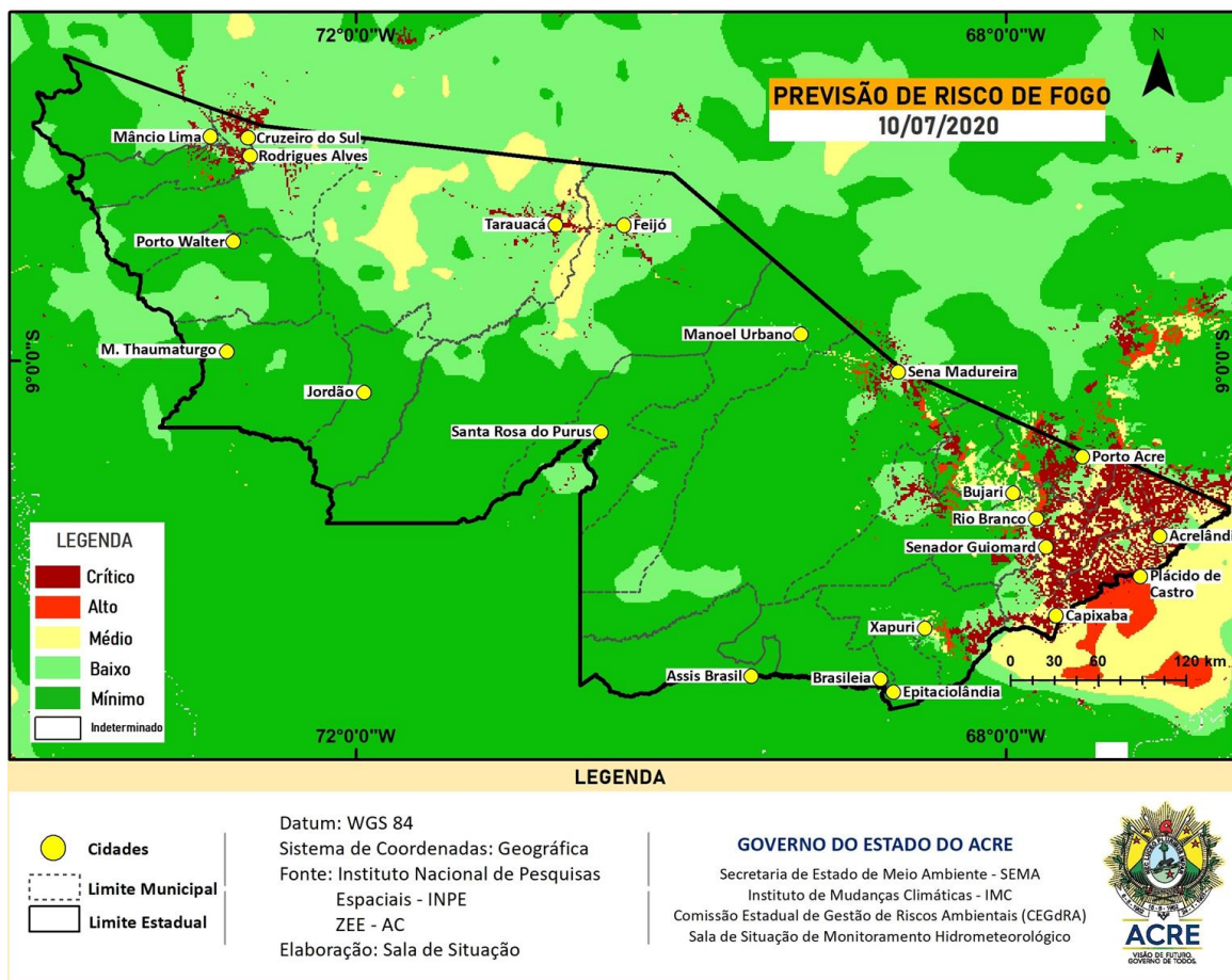
Figura 8 – Risco de Fogo para o estado do Acre em 10/07/2020
