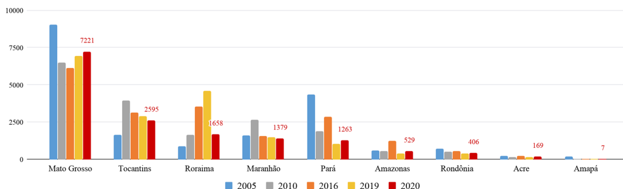
Figura 2 – Distribuição comparativa dos focos de queimadas acumulados de 01/01 a 09/07 na Amazônia legal, nos anos de 2005, 2010, 2016, 2019 e 2020 (Satélite de Referência AQUA Tarde)
