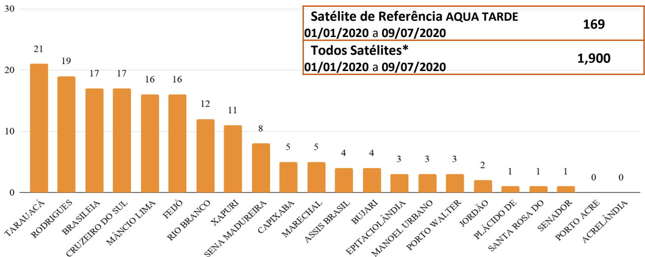
Figura 3 – Distribuição dos focos de queimadas acumulados de 01/01/2020 a 09/07/2020, no Estado do Acre. (Satélite de referência AQUA TARDE)
