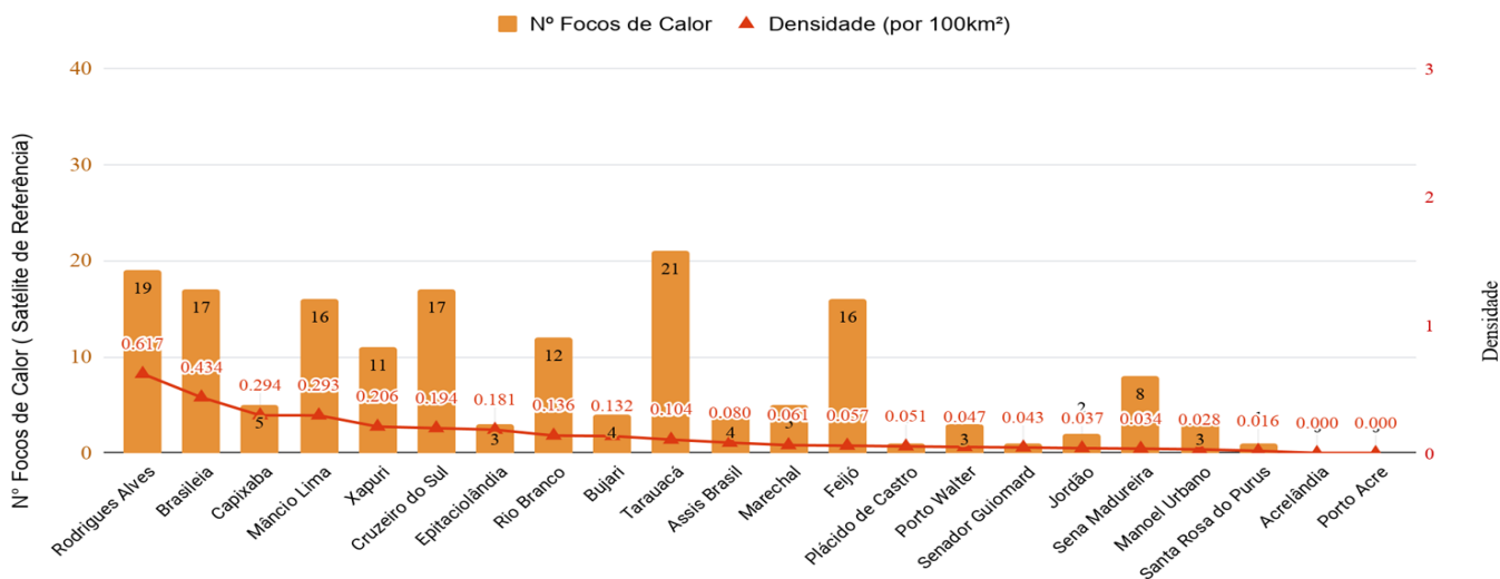
Figura 6 – Ocorrência de focos de queimadas e densidade por km 2 , por município em 01/01/2020 a 09/07/2020 (Satélite de referência AQUA TARDE)
