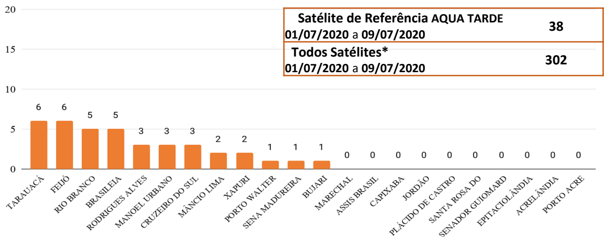
Figura 4 – Distribuição dos focos de queimadas acumulados de 01/07/2020 a 09/07/2020, no Estado do Acre. (Satélite de referência AQUA TARDE)
