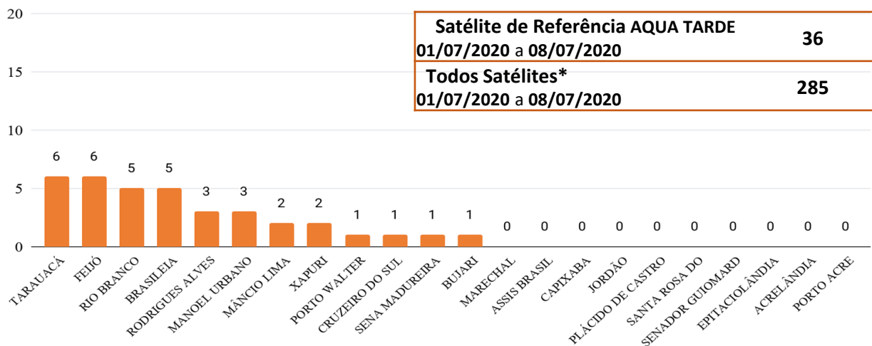
Figura 4 – Distribuição dos focos de queimadas acumulados de 01/07/2020 a 08/07/2020, no Estado do Acre. (Satélite de referência AQUA TARDE)
