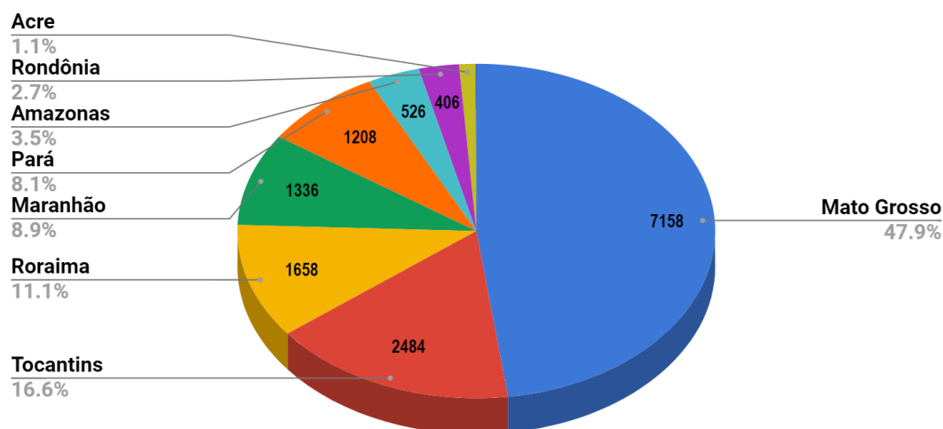
Figura 1 – Distribuição percentual dos focos de queimadas acumulados em 01/01/2020 a 08/07/2020 na Amazônia legal (Satélite de Referência AQUA Tarde)
