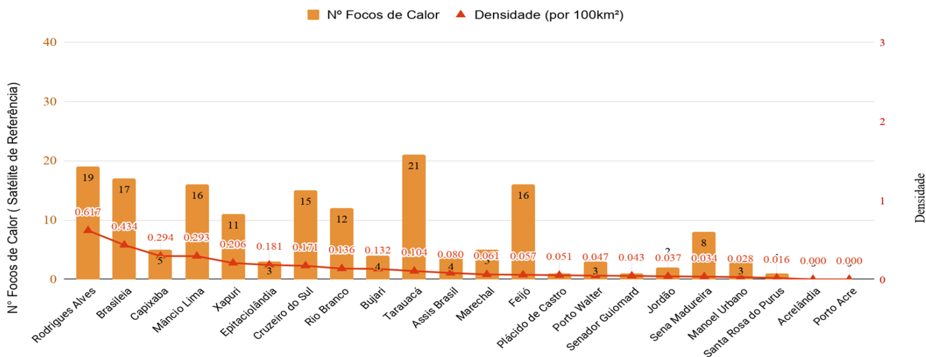
Figura 6 – Ocorrência de focos de queimadas e densidade por km 2 , por município em 01/01/2020 a 08/07/2020 (Satélite de referência AQUA TARDE)
