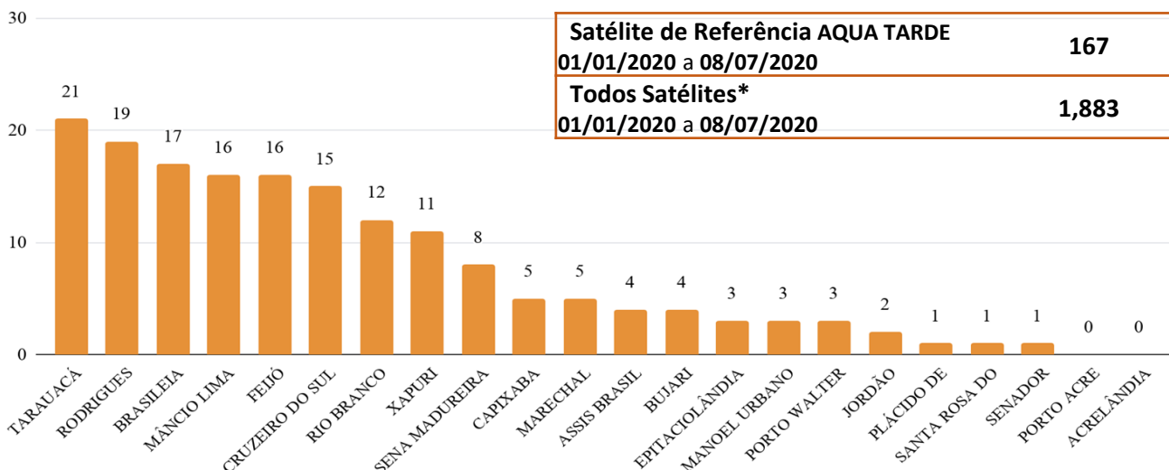
Figura 3 – Distribuição dos focos de queimadas acumulados de 01/01/2020 a 08/07/2020, no Estado do Acre. (Satélite de referência AQUA TARDE)
