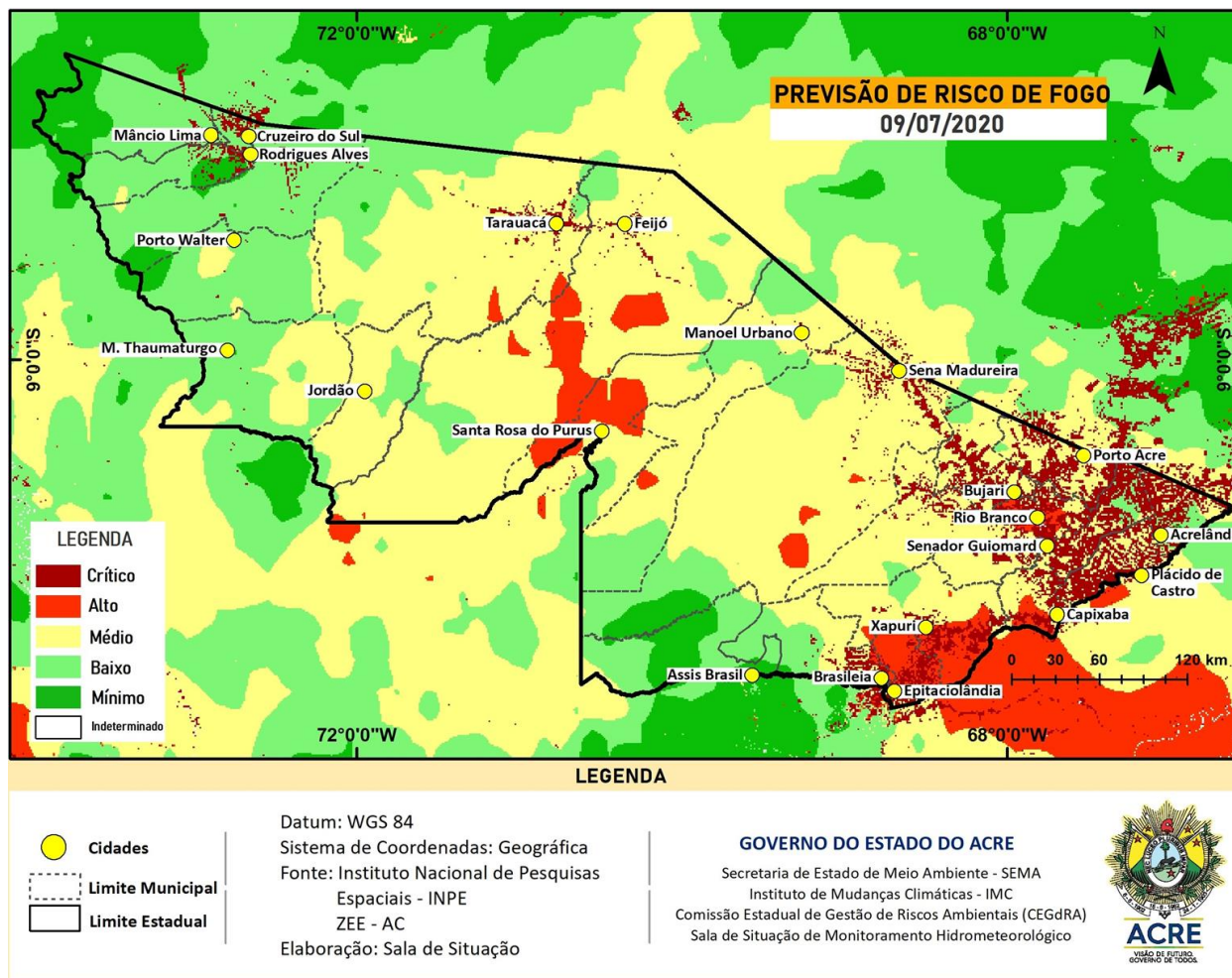
Figura 8 – Risco de Fogo para o estado do Acre em 09/07/2020
