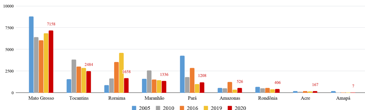
Figura 2 – Distribuição comparativa dos focos de queimadas acumulados de 01/01 a 08/07 na Amazônia legal, nos anos de 2005, 2010, 2016, 2019 e 2020 (Satélite de Referência AQUA Tarde)
