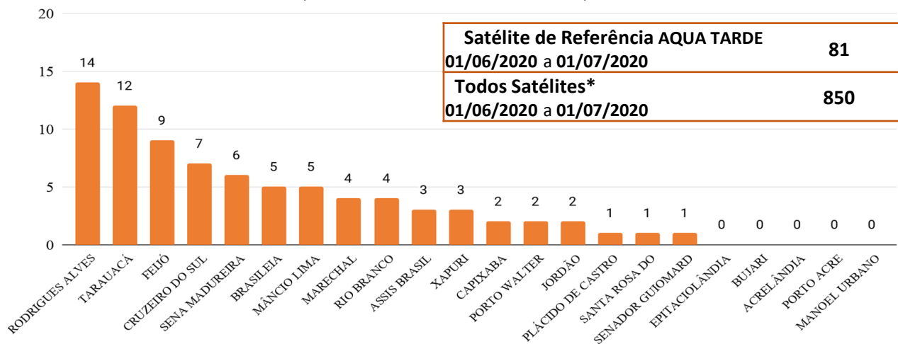
Figura 4 – Distribuição dos focos de queimadas acumulados de 01/06/2020 a 01/07/2020, no Estado do Acre. (Satélite de referência AQUA TARDE)
