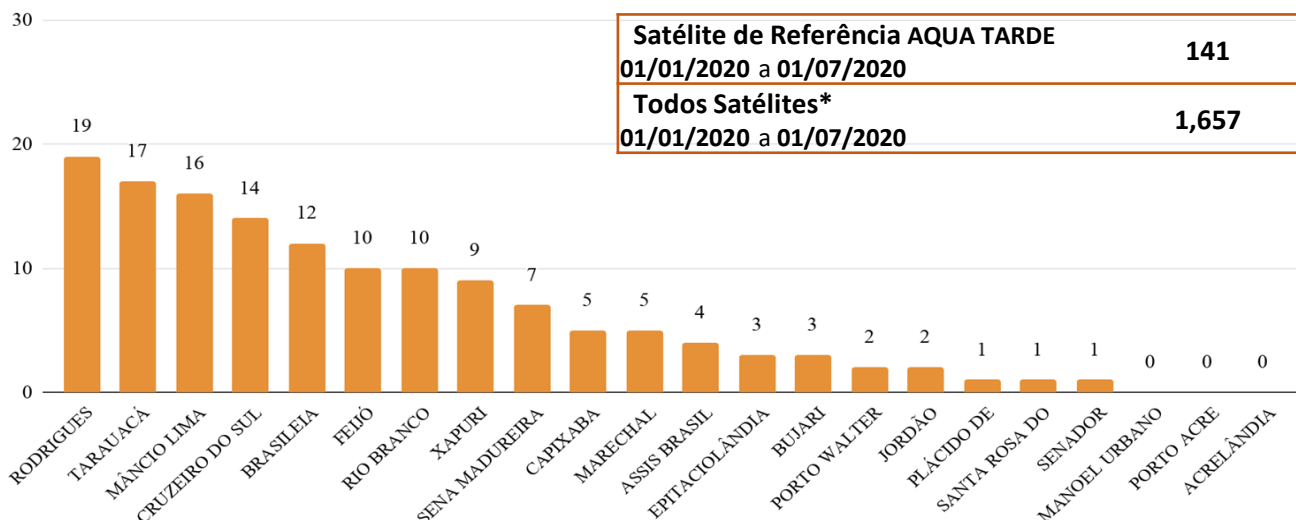
Figura 3 – Distribuição dos focos de queimadas acumulados de 01/01/2020 a 01/07/2020, no Estado do Acre. (Satélite de referência AQUA TARDE)
