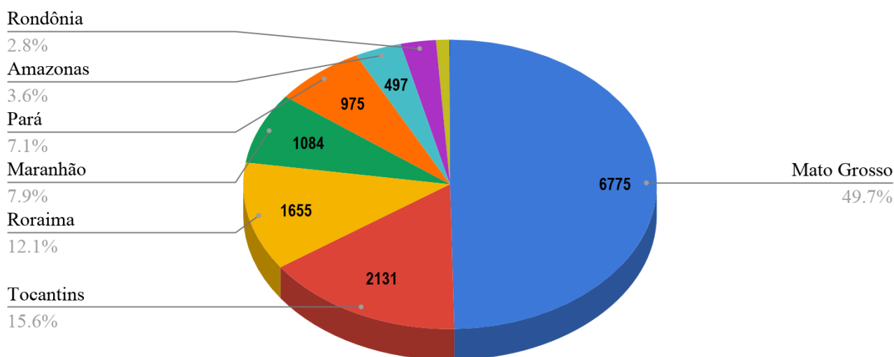
Figura 1 – Distribuição percentual dos focos de queimadas acumulados em 01/01/2020 a 01/07/2020 na Amazônia legal ( Satélite de Referência AQUA Tarde)
