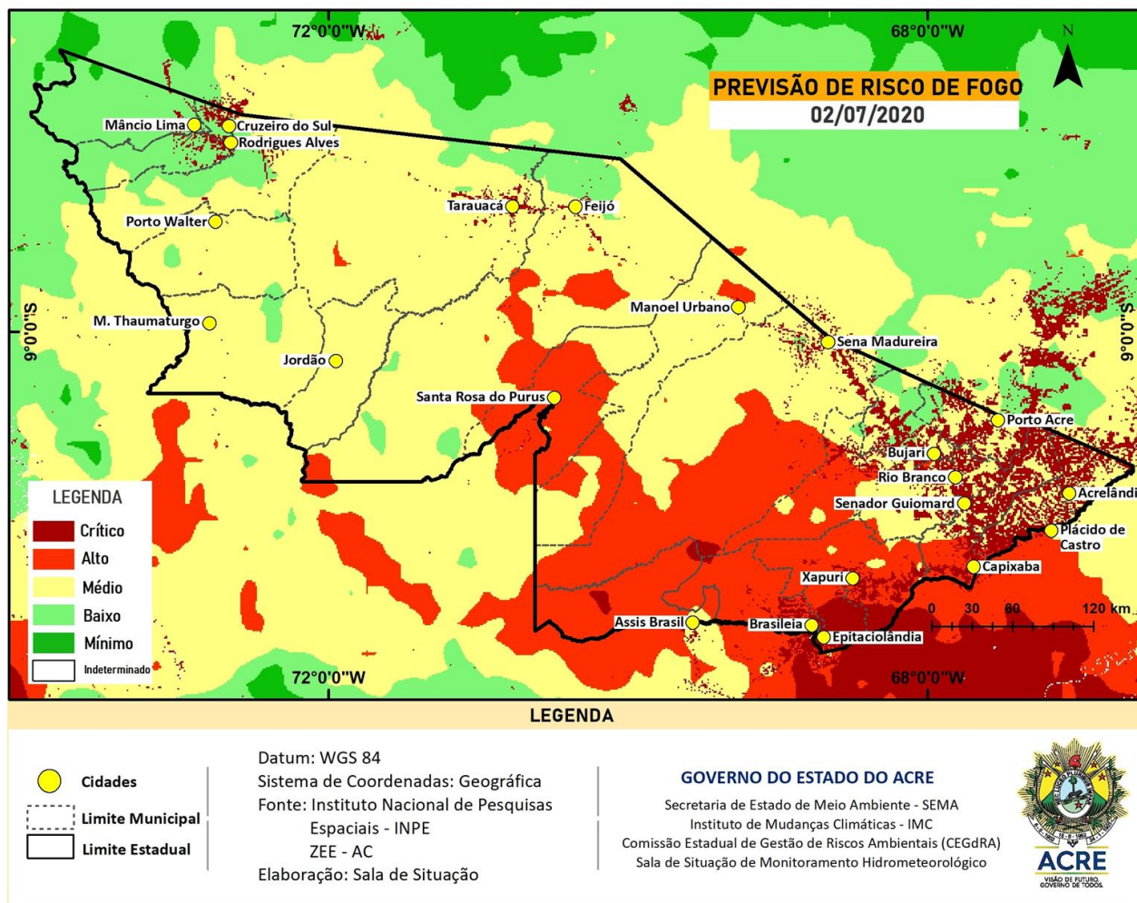
Figura 8 – Risco de Fogo para o estado do Acre em 02/07/2020
