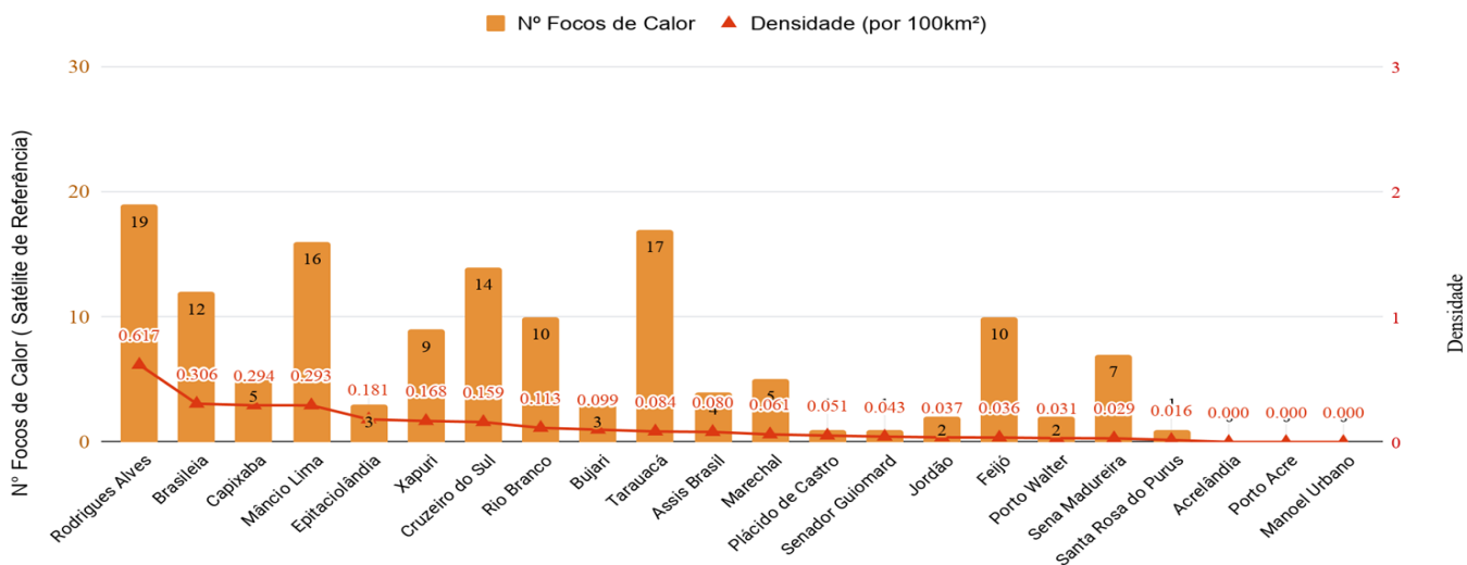
Figura 6 – Ocorrência de focos de queimadas e densidade por km 2 , por município em 01/01/2020 a 01/07/2020 ( Satélite de referência AQUA TARDE)
