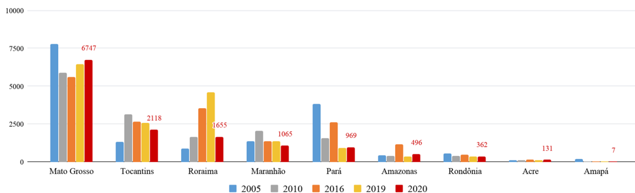
Figura 2 – Distribuição comparativa dos focos de queimadas acumulados de 01/01 a 01/07 na Amazônia legal, nos anos de 2005, 2010, 2016, 2019 e 2020 ( Satélite de Referência AQUA Tarde)
