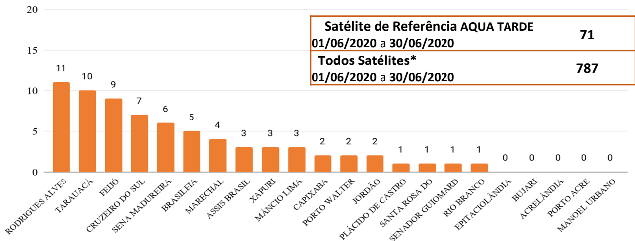
Figura 4 – Distribuição dos focos de queimadas acumulados de 01/06/2020 a 30/06/2020, no Estado do Acre. (Satélite de referência AQUA TARDE)
