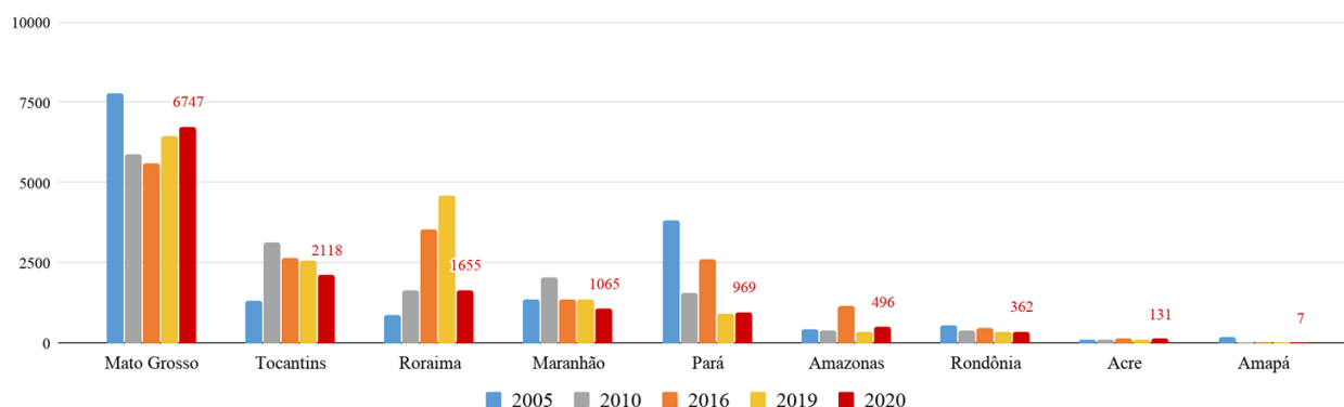
Figura 2 – Distribuição comparativa dos focos de queimadas acumulados de 01/01 a 30/06 na Amazônia legal, nos anos de 2005, 2010, 2016, 2019 e 2020 ( Satélite de Referência AQUA Tarde)
