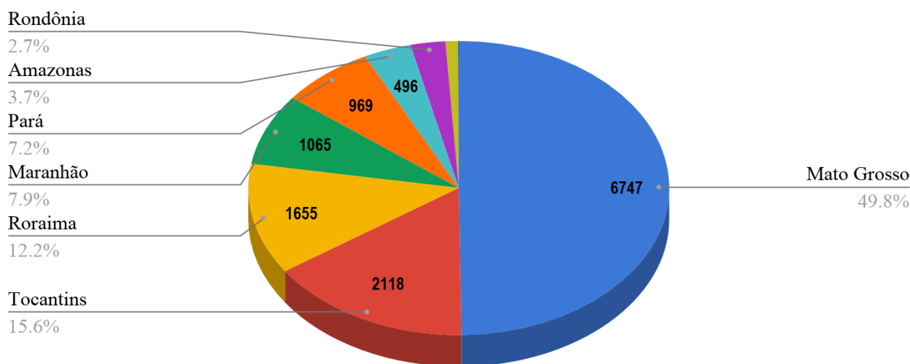
Figura 1 – Distribuição percentual dos focos de queimadas acumulados em 01/01/2020 a 30/06/2020 na Amazônia legal ( Satélite de Referência AQUA Tarde)
