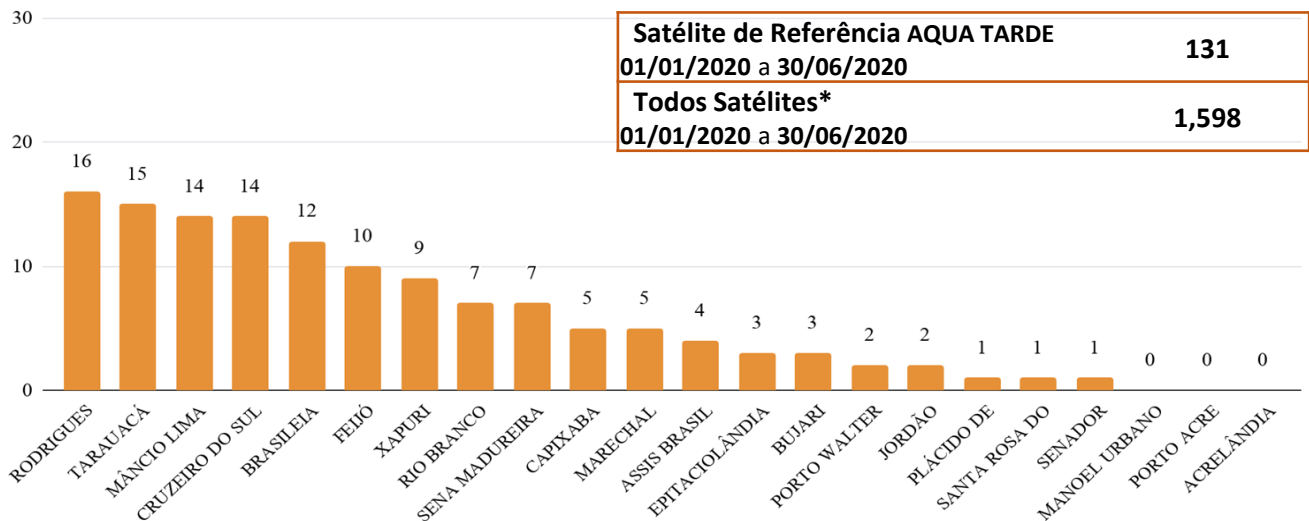
Figura 3 – Distribuição dos focos de queimadas acumulados de 01/01/2020 a 30/06/2020, no Estado do Acre. (Satélite de referência AQUA TARDE)
