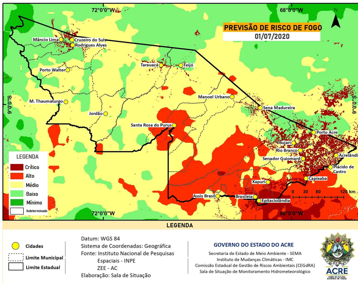
Figura 8 – Risco de Fogo para o estado do Acre em 01/07/2020
