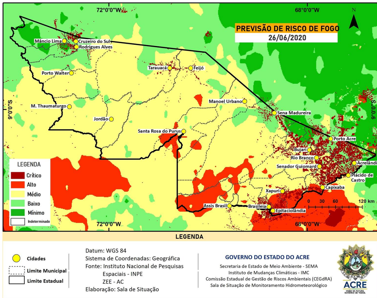
Figura 8 – Risco de Fogo para o estado do Acre em 26/06/2020
