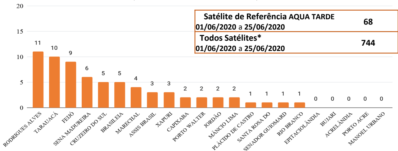
Figura 4 – Distribuição dos focos de queimadas acumulados de 01/06/2020 a 25/06/2020, no Estado do Acre. (Satélite de referência AQUA TARDE)
