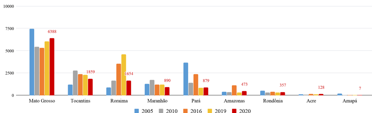
Figura 2 – Distribuição comparativa dos focos de queimadas acumulados de 01/01 a 25/06 na Amazônia legal, nos anos de 2005, 2010, 2016, 2019 e 2020 ( Satélite de Referência AQUA Tarde)
