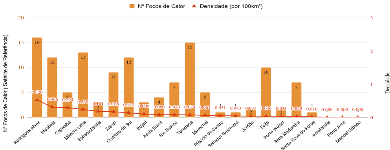
Figura 6 – Ocorrência de focos de queimadas e densidade por km 2 , por município em 01/01/2020 a 25/06/2020 ( Satélite de referência AQUA TARDE)
