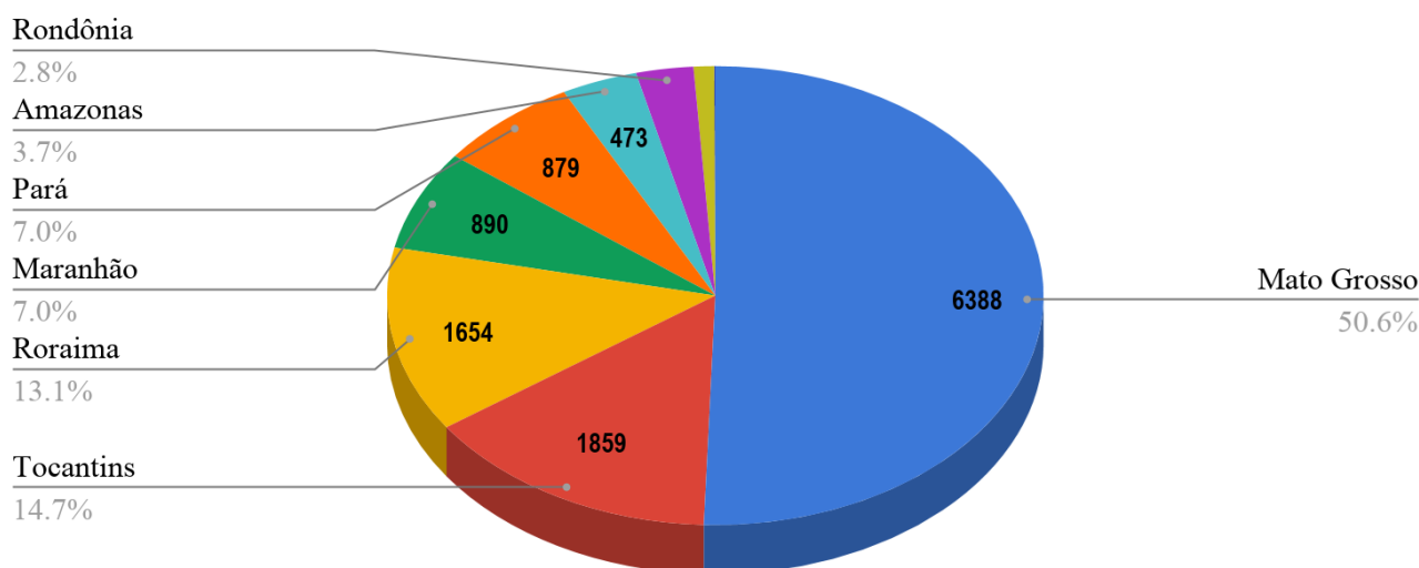
Figura 1 – Distribuição percentual dos focos de queimadas acumulados em 01/01/2020 a 25/06/2020 na Amazônia legal ( Satélite de Referência AQUA Tarde)
