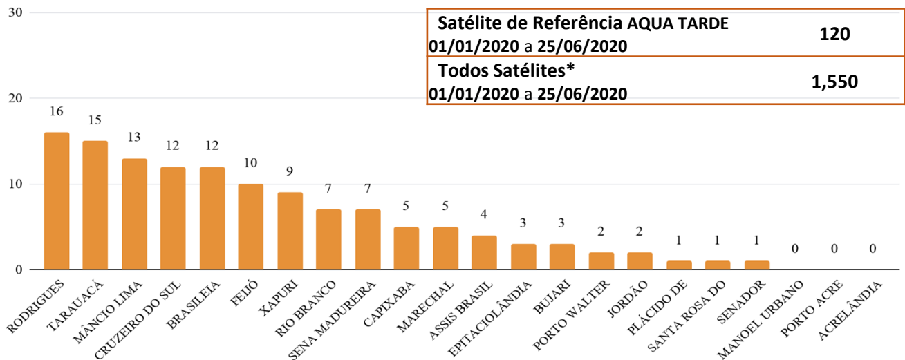
Figura 3 – Distribuição dos focos de queimadas acumulados de 01/01/2020 a 25/06/2020, no Estado do Acre. (Satélite de referência AQUA TARDE)
