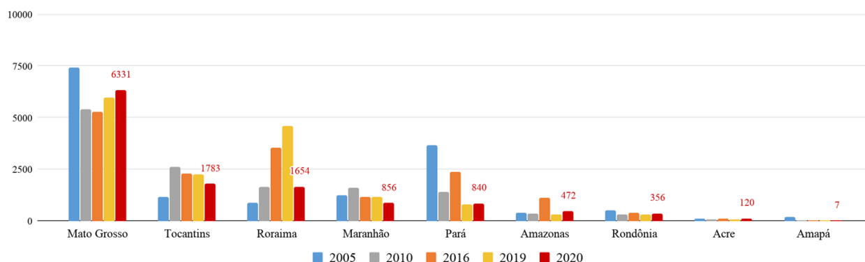
Figura 2 – Distribuição comparativa dos focos de queimadas acumulados de 01/01 a 24/06 na Amazônia legal, nos anos de 2005, 2010, 2016, 2019 e 2020 ( Satélite de Referência AQUA Tarde)
