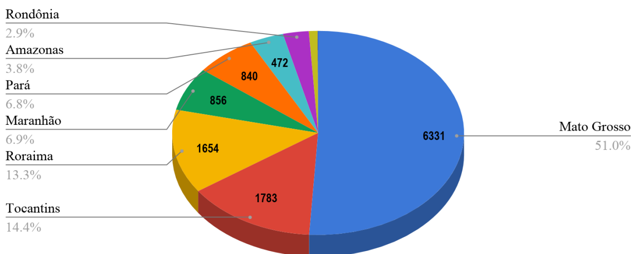
Figura 1 – Distribuição percentual dos focos de queimadas acumulados em 01/01/2020 a 24/06/2020 na Amazônia legal ( Satélite de Referência AQUA Tarde)
