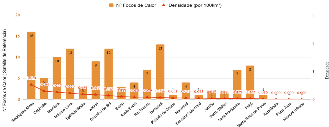
Figura 6 – Ocorrência de focos de queimadas e densidade por km 2 , por município em 01/01/2020 a 24/06/2020 ( Satélite de referência AQUA TARDE)
