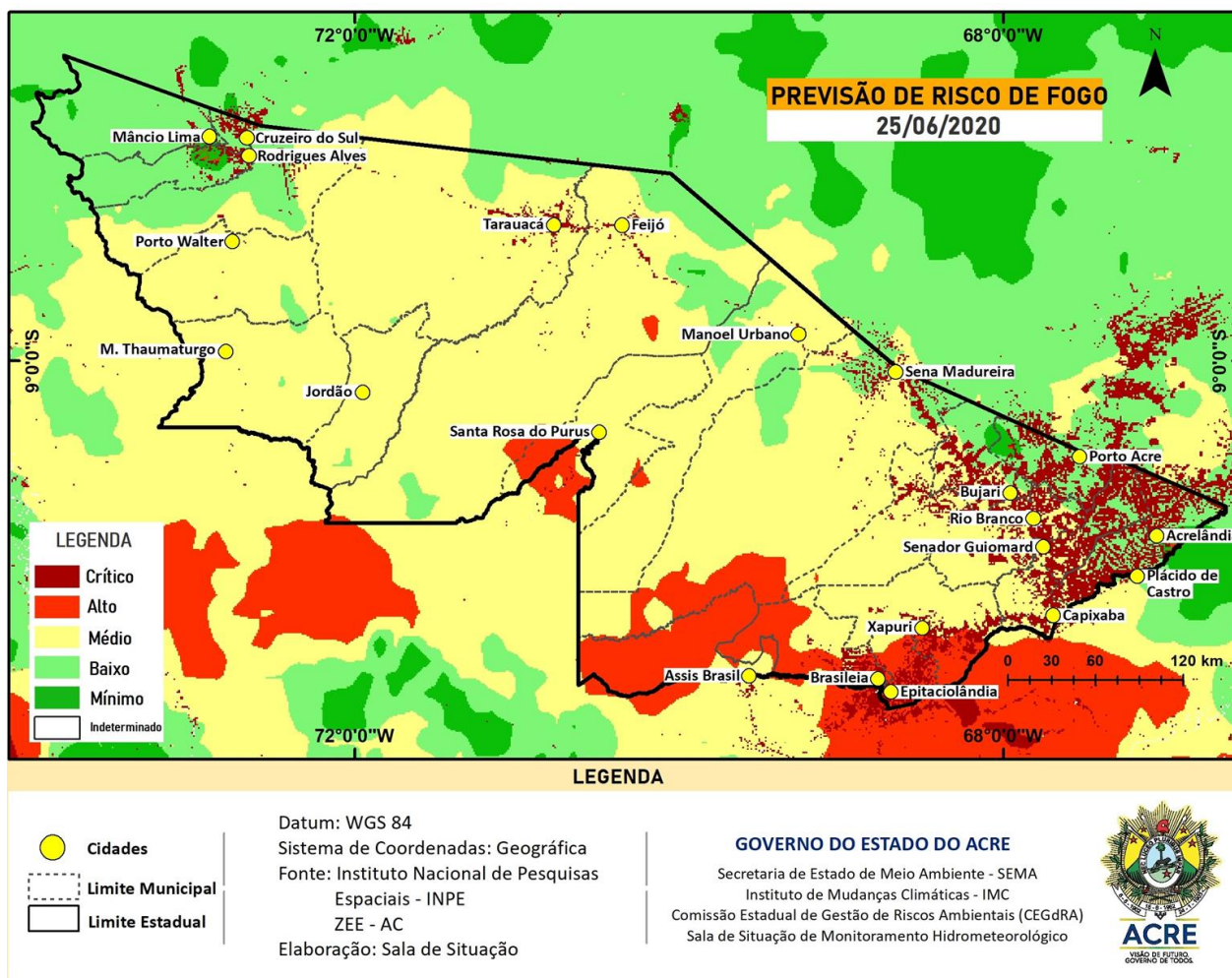
Figura 8 – Risco de Fogo para o estado do Acre em 25/06/2020
