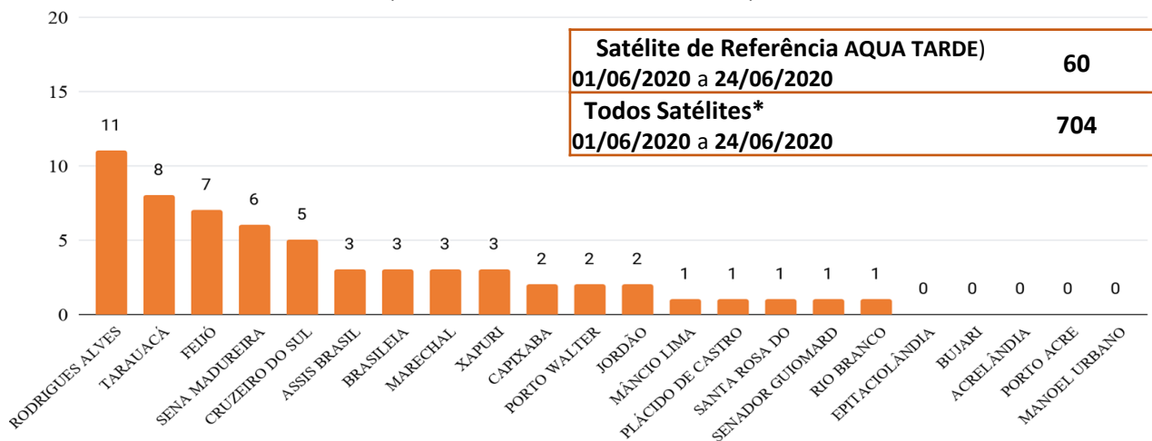
Figura 4 – Distribuição dos focos de queimadas acumulados de 01/06/2020 a 24/06/2020, no Estado do Acre. (Satélite de referência AQUA TARDE)
