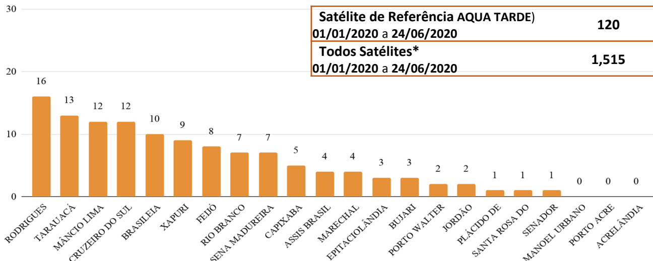
Figura 3 – Distribuição dos focos de queimadas acumulados de 01/01/2020 a 24/06/2020, no Estado do Acre. (Satélite de referência AQUA TARDE)
