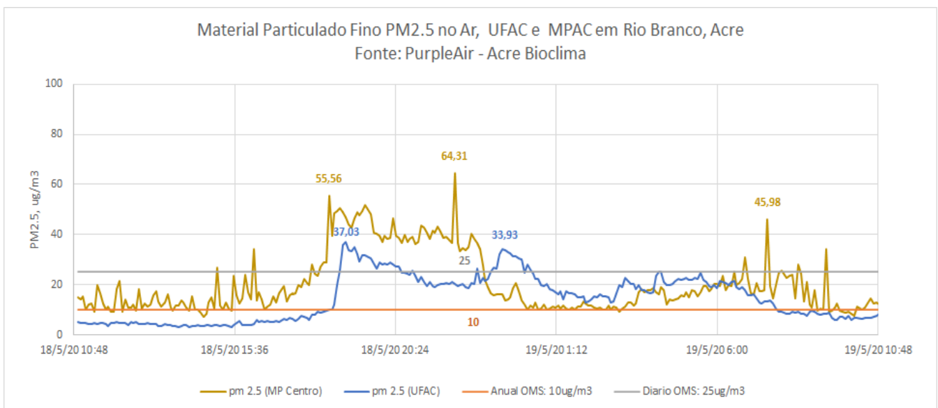
Figura 9 – Gráfico de material Particulado PM 2,5 \mu\text{g}/\text{m}^3
