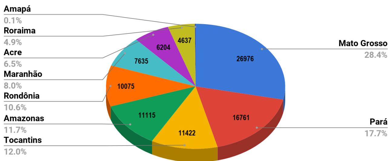
Figura 1 – Distribuição percentual dos focos de queimadas acumulados em 01/01/2019 a 25/09/2019 na Amazônia legal ( Satélite de Referência AQUA Tarde)
