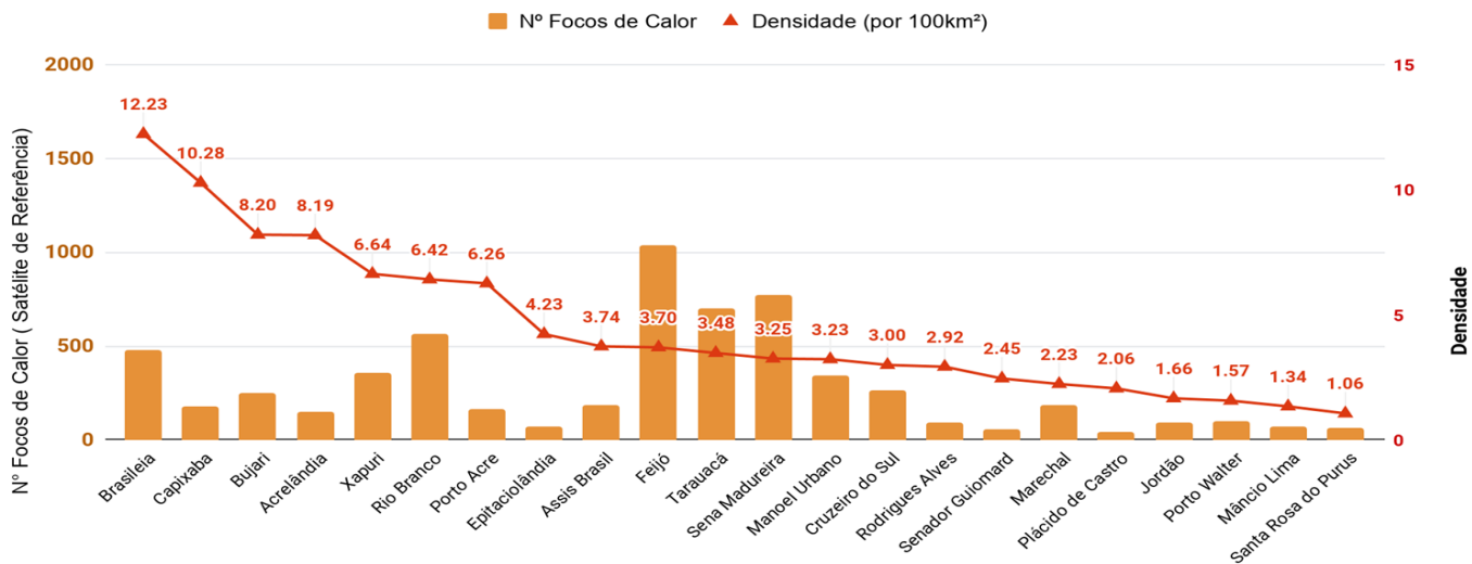
Figura 6 – Ocorrência de focos de queimadas e densidade por km 2 , por município em 01/01/2019 a 25/09/2019 ( Satélite de referência AQUA TARDE)
