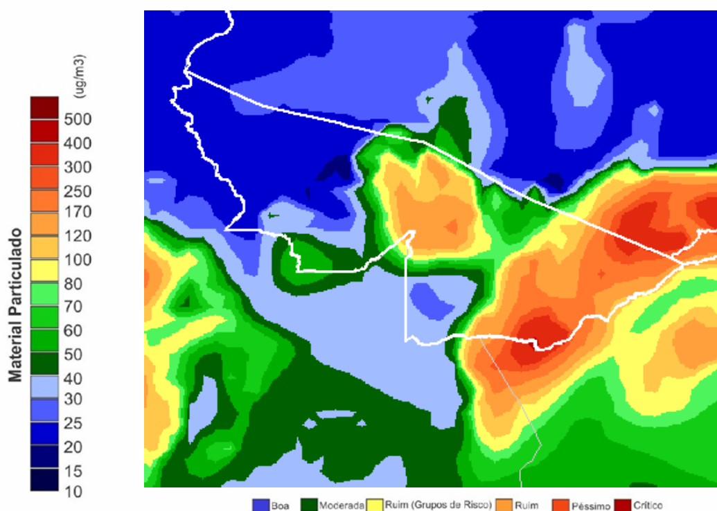
Figura 10 – Mapa de material Particulado CPTEC/INPE em 26/09/2019
