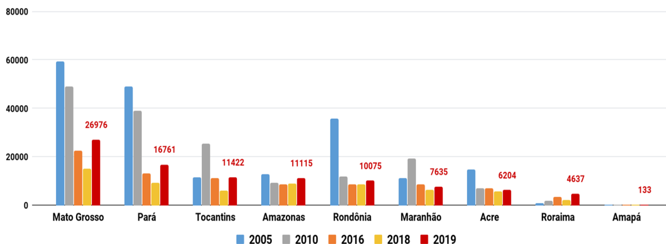
Figura 2 – Distribuição comparativa dos focos de queimadas acumulados de 01/01 a 25/09 na Amazônia legal, nos anos de 2005, 2010, 2016, 2018 e 2019 ( Satélite de Referência AQUA Tarde)
