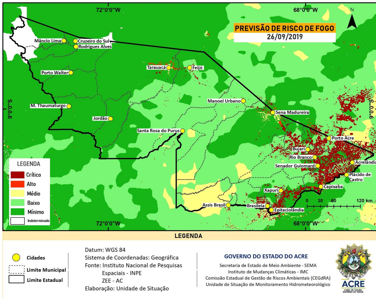
Figura 9 – Risco de Fogo para o estado do Acre em 26/09/2019
