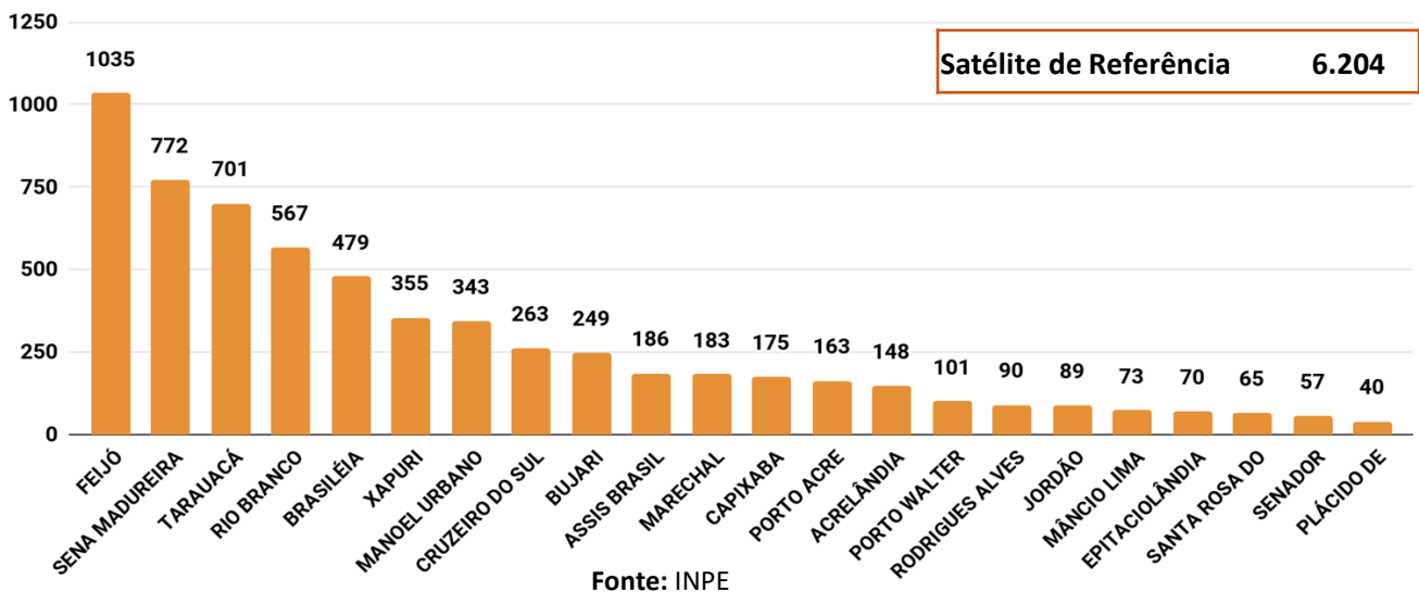
Figura 3 – Distribuição dos focos de queimadas acumulados de 01/01/2019 a 25/09/2019, no Estado do Acre. ( Satélite de referência AQUA TARDE)
