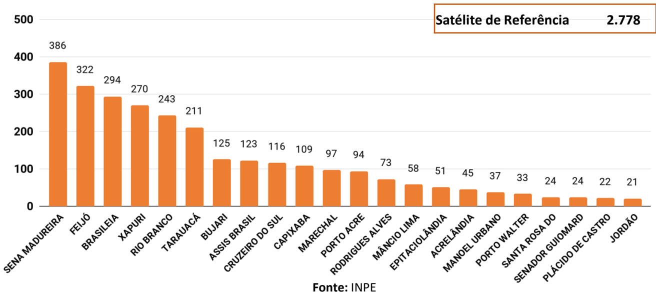
Figura 4 – Distribuição dos focos de queimadas acumulados no mês setembro de 01/09/2019 a 25/09/2019. ( Satélite de referência AQUA TARDE)
