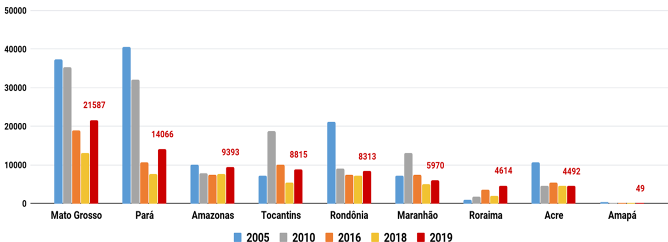
Figura 2 – Distribuição comparativa dos focos de queimadas acumulados de 01/01 a 10/09 na Amazônia legal, nos anos de 2005, 2010, 2016, 2018 e 2019 ( Satélite de Referência AQUA Tarde)
