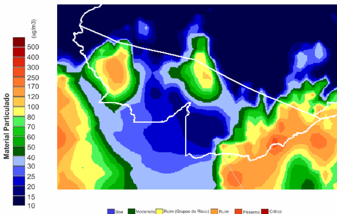
Figura 9 – Mapa de material Particulado CPTEC/INPE em 11/09/2019
