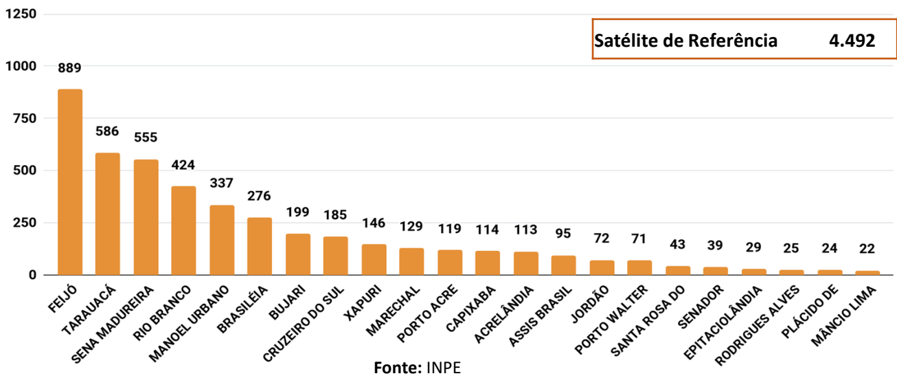
Figura 3 – Distribuição dos focos de queimadas acumulados de 01/01/2019 a 10/09/2019, no Estado do Acre. ( Satélite de referência AQUA TARDE)
