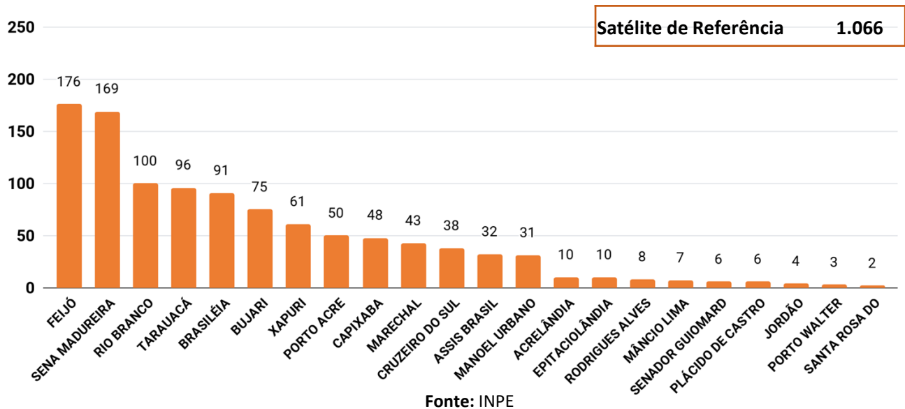
Figura 4 – Distribuição dos focos de queimadas acumulados no mês setembro de 01/09/2019 a 10/09/2019. ( Satélite de referência AQUA TARDE)
