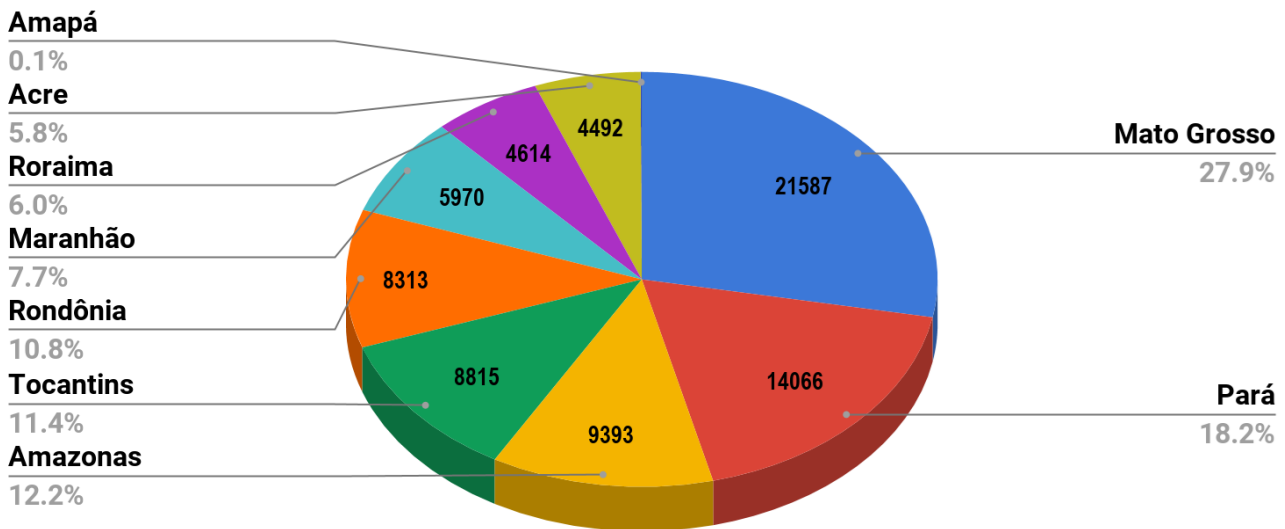
Figura 1 – Distribuição percentual dos focos de queimadas acumulados em 01/01/2019 a 10/09/2019 na Amazônia legal ( Satélite de Referência AQUA Tarde)
