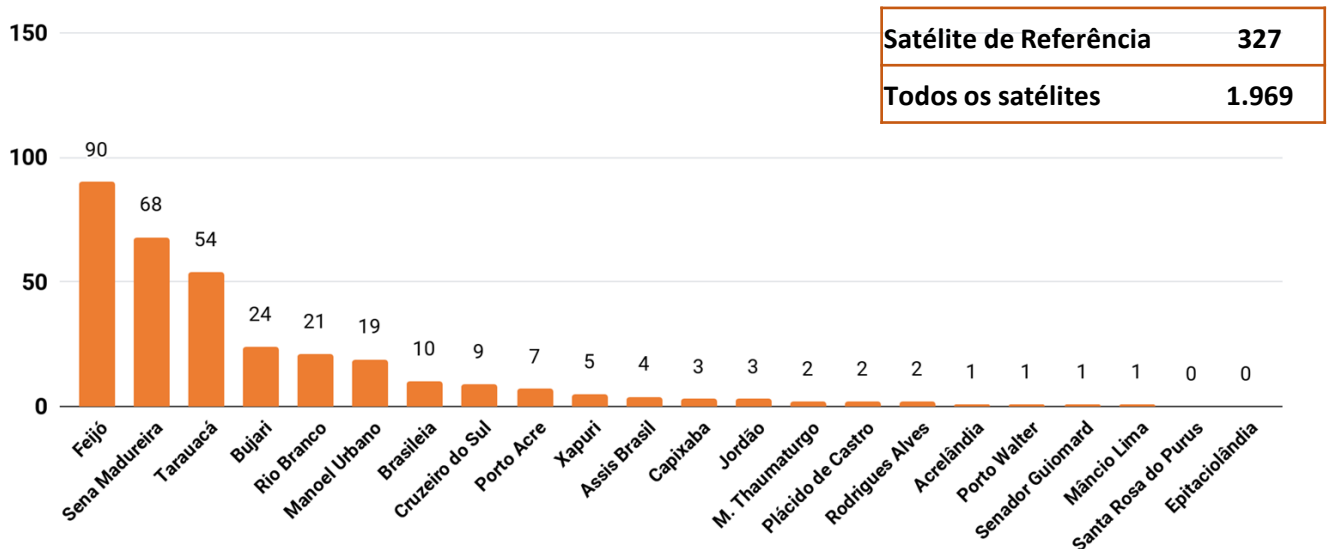
Figura 4 – Distribuição dos focos de queimadas acumulados no mês setembro de 01/09/2019 a 01/09/2019. ( Satélite de referência AQUA TARDE)
