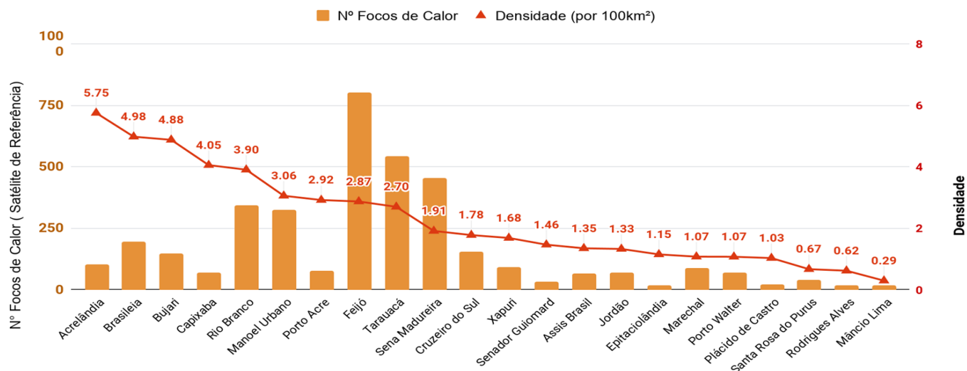
Figura 6 – Ocorrência de focos de queimadas e densidade por km 2 , por município em 01/01/2019 a 01/09/2019 ( Satélite de referência AQUA_TARDE)
