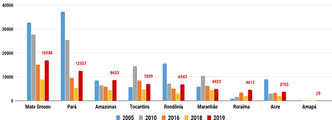
Figura 2 – Distribuição comparativa dos focos de queimadas acumulados de 01/01 a 01/09 na Amazônia legal, nos anos de 2005, 2010, 2016, 2018 e 2019 ( Satélite de Referência AQUA Tarde)
