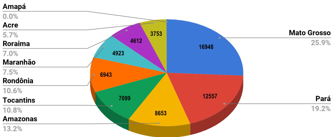
Figura 1 – Distribuição percentual dos focos de queimadas acumulados em 01/01/2019 a 01/09/2019 na Amazônia legal ( Satélite de Referência AQUA Tarde)
