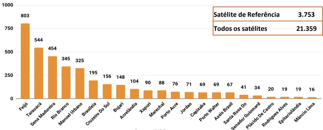
Figura 3 – Distribuição dos focos de queimadas acumulados de 01/01/2019 a 01/09/2019, no Estado do Acre. ( Satélite de referência AQUA TARDE)
