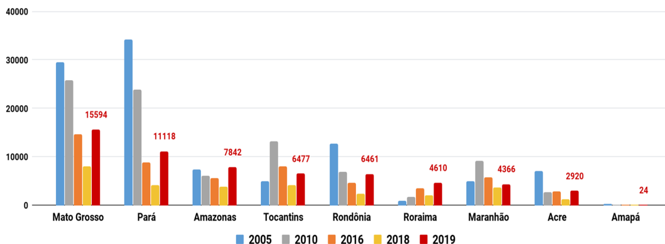
Figura 2 – Distribuição comparativa dos focos de queimadas acumulados de 01/01 a 27/08 na Amazônia legal, nos anos de 2005, 2010, 2016, 2018 e 2019 ( Satélite de Referência AQUA Tarde)
