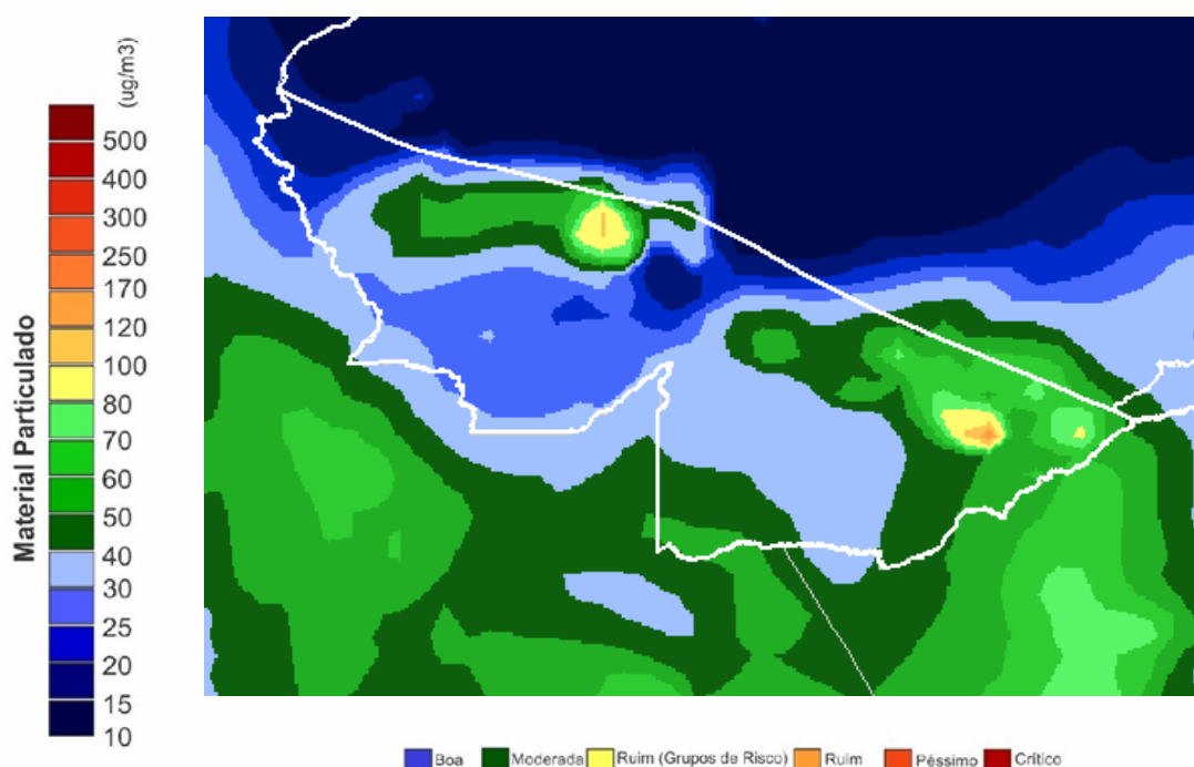
Figura 9 – Mapa de material Particulado CPTEC/INPE em 28/08/2019
