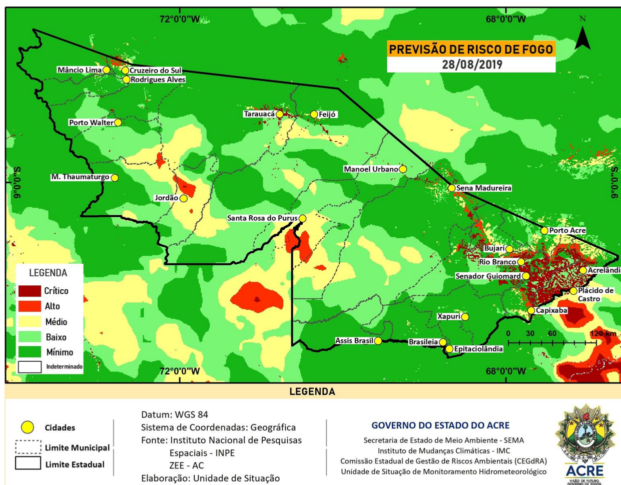
Figura 8 – Risco de Fogo para o estado do Acre em 28/08/2019
