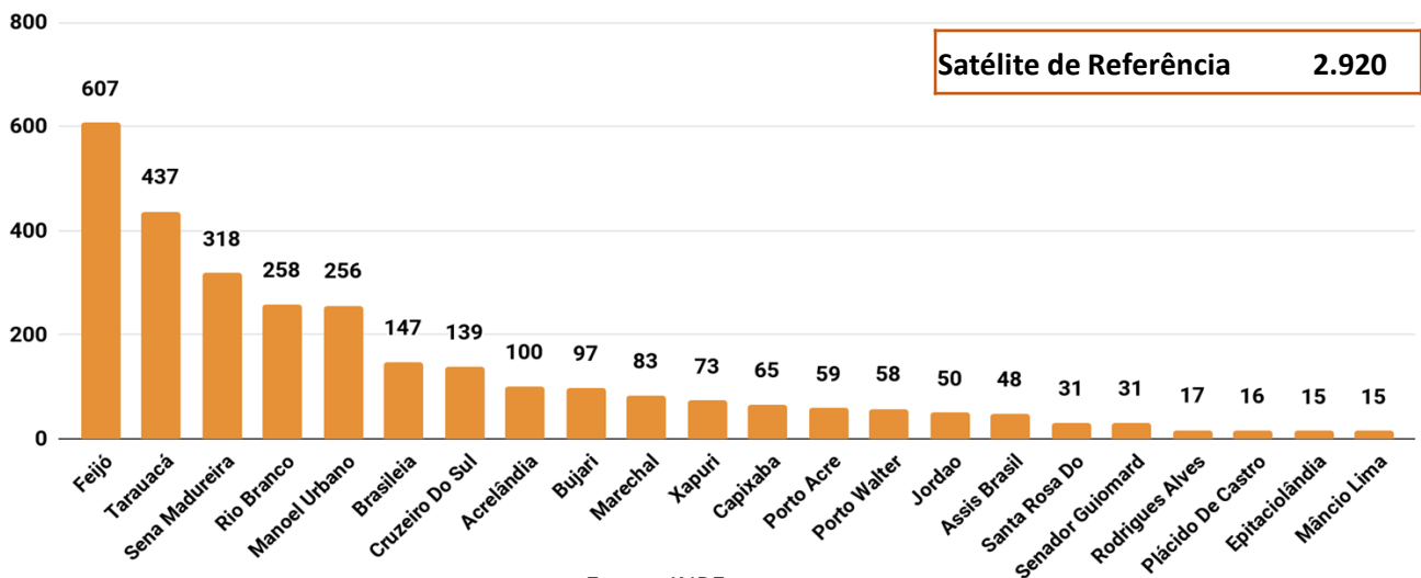
Figura 3 – Distribuição dos focos de queimadas acumulados de 01/01/2019 a 27/08/2019, no Estado do Acre. ( Satélite de referência AQUA TARDE)
