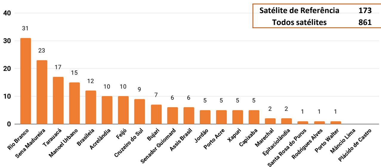
Figura 4 – Distribuição dos focos de queimadas acumulados no mês julho de 01/07/2019 a 29/07/2019. ( Satélite de referência AQUA_M-T)
