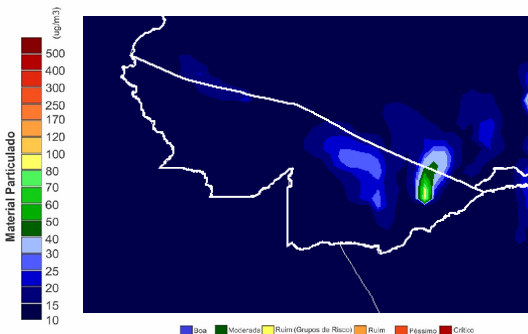
Figura 10 – Mapa de material Particulado CPTEC/INPE em 30/07/2019
