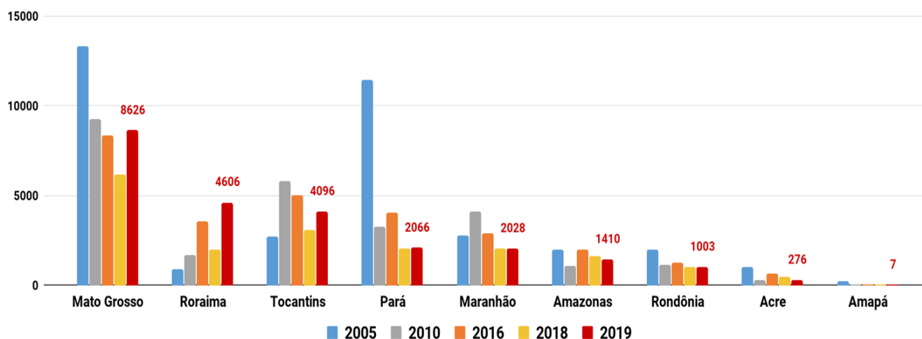
Figura 2 – Distribuição comparativa dos focos de queimadas acumulados de 01/01 a 29/07 na Amazônia legal, nos anos de 2005, 2010, 2016, 2018 e 2019 ( Satélite de Referência AQUA Tarde)
