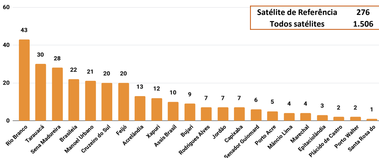
Figura 3 – Distribuição dos focos de queimadas acumulados de 01/01/2019 a 29/07/2019, no Estado do Acre. ( Satélite de referência AQUA_M-T)
