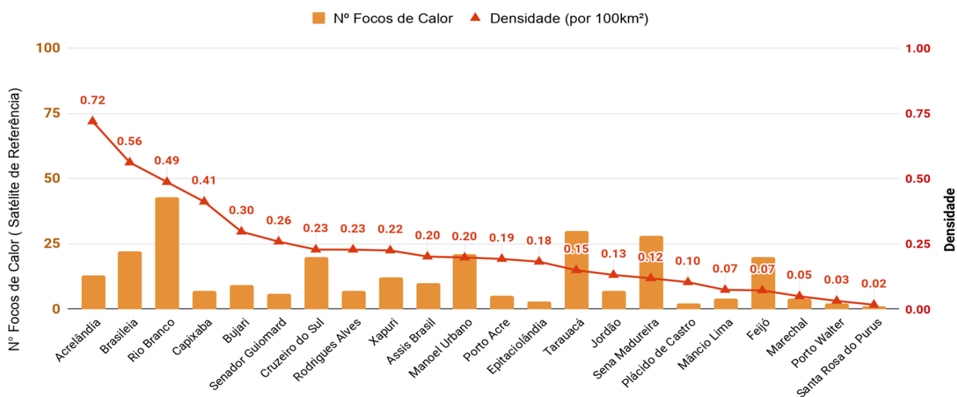
Figura 6 – Ocorrência de focos de queimadas e densidade por km 2 , por município em 01/01/2019 a 29/07/2019 ( Satélite de referência AQUA_M-T)
