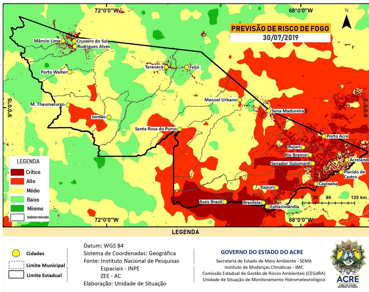
Figura 9 – Risco de Fogo para o estado do Acre em 30/07/2019
