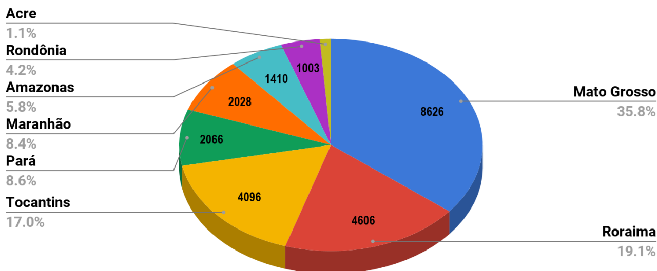
Figura 1 – Distribuição percentual dos focos de queimadas acumulados em 01/01/2019 a 29/07/2019 na Amazônia legal ( Satélite de Referência AQUA Tarde)
