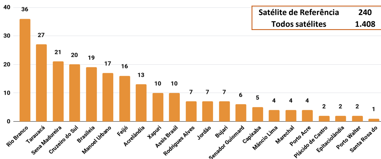
Figura 3 – Distribuição dos focos de queimadas acumulados de 01/01/2019 a 28/07/2019, no Estado do Acre. ( Satélite de referência AQUA_M-T)
