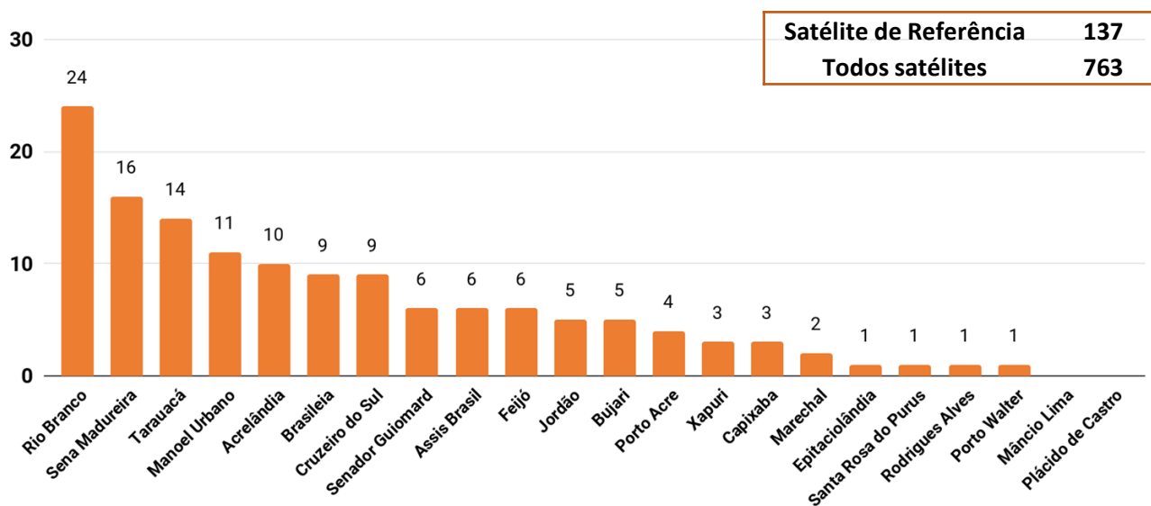
Figura 4 – Distribuição dos focos de queimadas acumulados no mês julho de 01/07/2019 a 28/07/2019. ( Satélite de referência AQUA_M-T)
