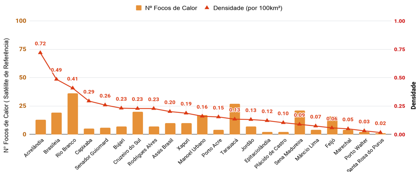
Figura 6 – Ocorrência de focos de queimadas e densidade por km 2 , por município em 01/01/2019 a 28/07/2019 ( Satélite de referência AQUA_M-T)
