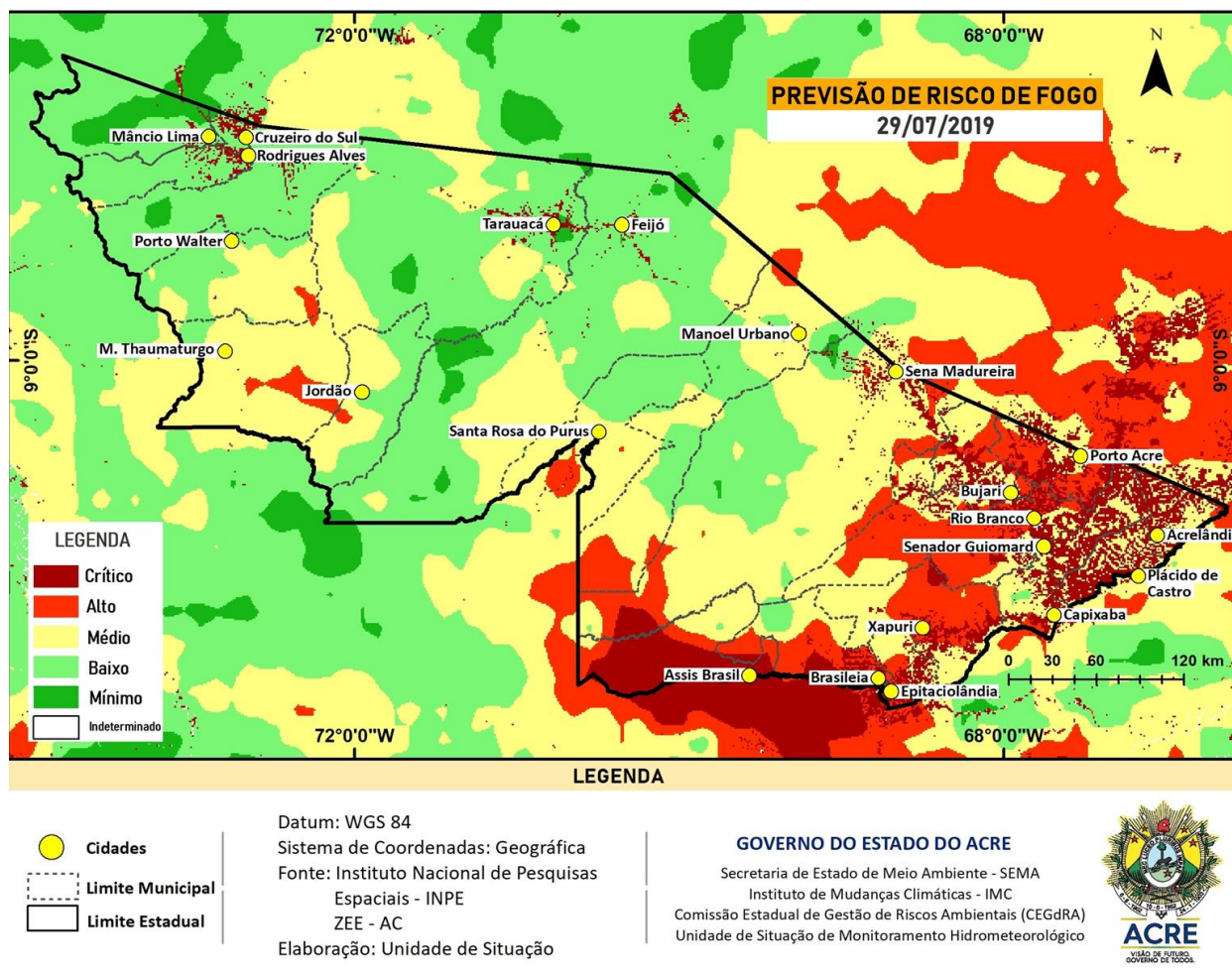
Figura 9 – Risco de Fogo para o estado do Acre em 29/07/2019
