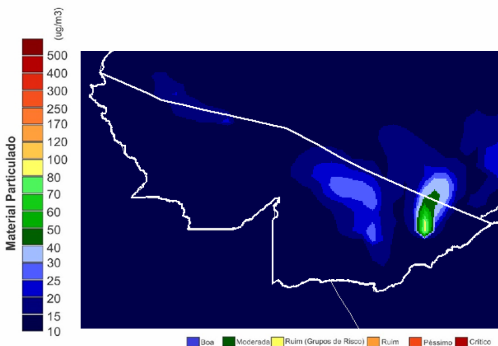
Figura 10 – Mapa de material Particulado CPTEC/INPE em 29/07/2019
