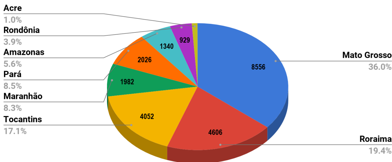
Figura 1 – Distribuição percentual dos focos de queimadas acumulados em 01/01/2019 a 28/07/2019 na Amazônia legal ( Satélite de Referência AQUA Tarde)
