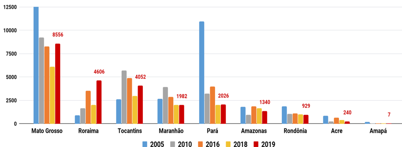
Figura 2 – Distribuição comparativa dos focos de queimadas acumulados de 01/01 a 28/07 na Amazônia legal, nos anos de 2005, 2010, 2016, 2018 e 2019 ( Satélite de Referência AQUA Tarde)
