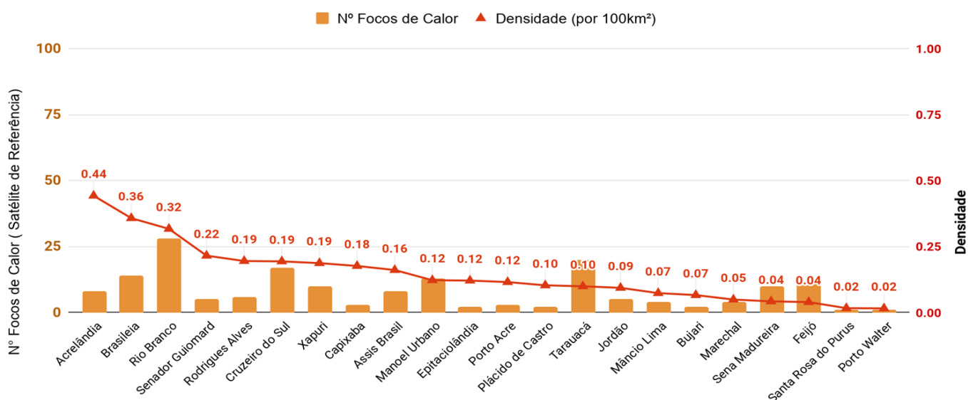
Figura 6 – Ocorrência de focos de queimadas e densidade por km 2 , por município em 01/01/2019 a 11/07/2019 ( Satélite de referência AQUA_M-T)
