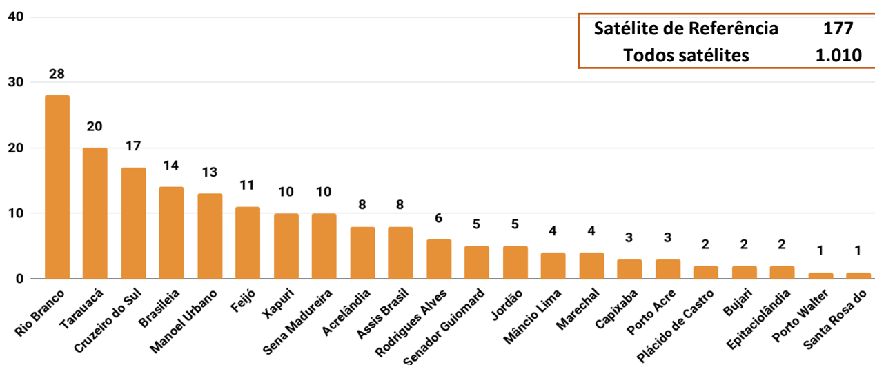
Figura 3 – Distribuição dos focos de queimadas acumulados de 01/01/2019 a 11/07/2019, no Estado do Acre. ( Satélite de referência AQUA_M-T)
