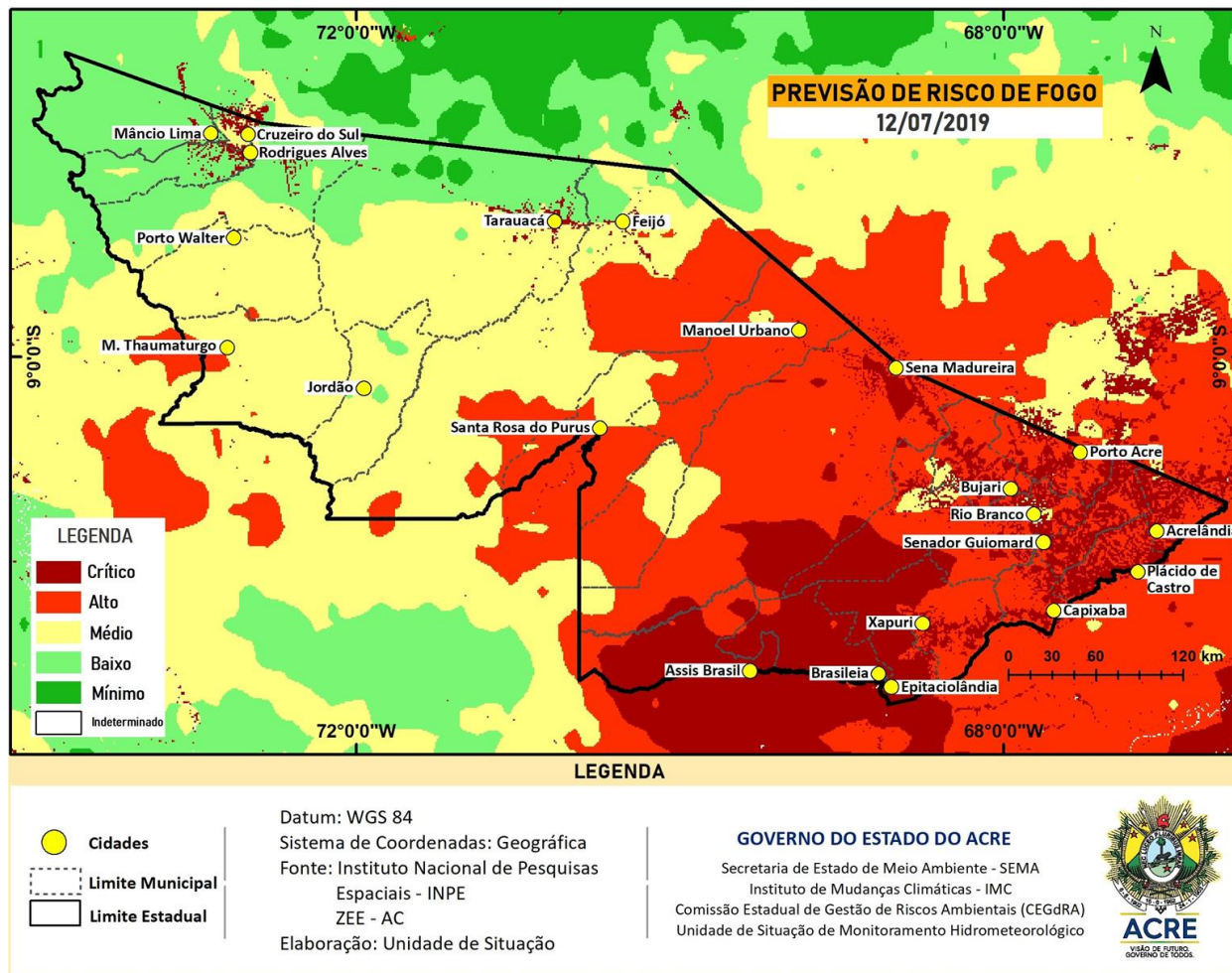
Figura 8 – Risco de Fogo para o estado do Acre em 12/07/2019
