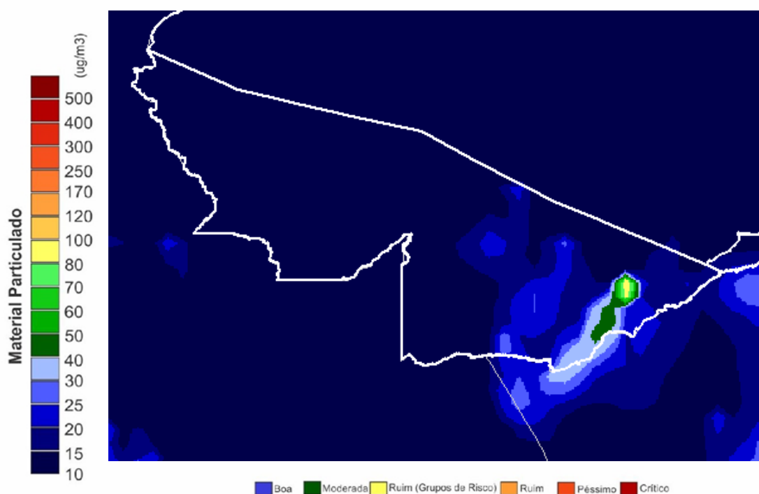
Figura 9 – Mapa de material Particulado CPTEC/INPE em 12/07/2019
