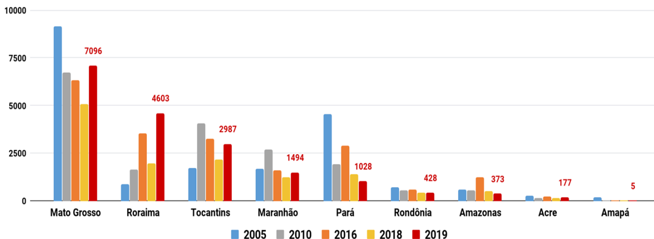
Figura 2 – Distribuição comparativa dos focos de queimadas acumulados de 01/01 a 11/07 na Amazônia legal, nos anos de 2005, 2010, 2016, 2018 e 2019 ( Satélite de Referência AQUA Tarde)
