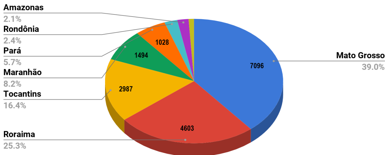
Figura 1 – Distribuição percentual dos focos de queimadas acumulados em 01/01/2019 a 11/07/2019 na Amazônia legal ( Satélite de Referência AQUA Tarde)
