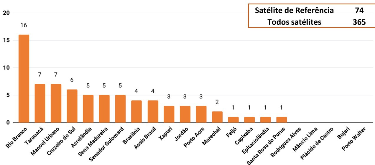
Figura 4 – Distribuição dos focos de queimadas acumulados no mês julho de 01/07/2019 a 11/07/2019. ( Satélite de referência AQUA_M-T)
