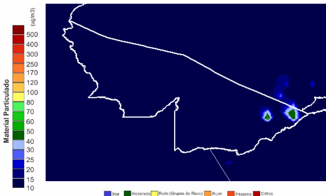
Figura 9 – Mapa de material Particulado CPTEC/INPE em 10/07/2019
