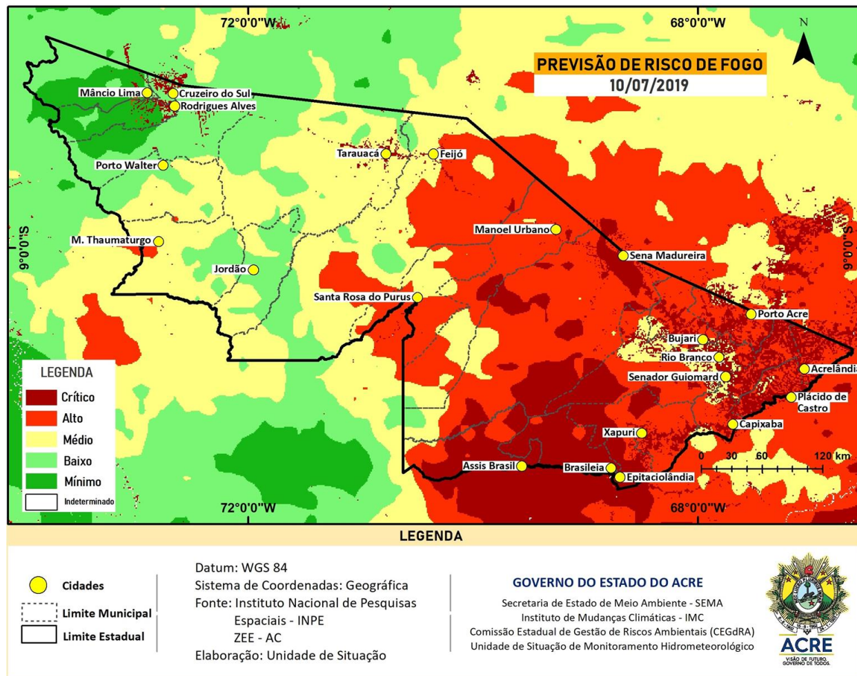
Figura 8 – Risco de Fogo para o estado do Acre em 10/07/2019
