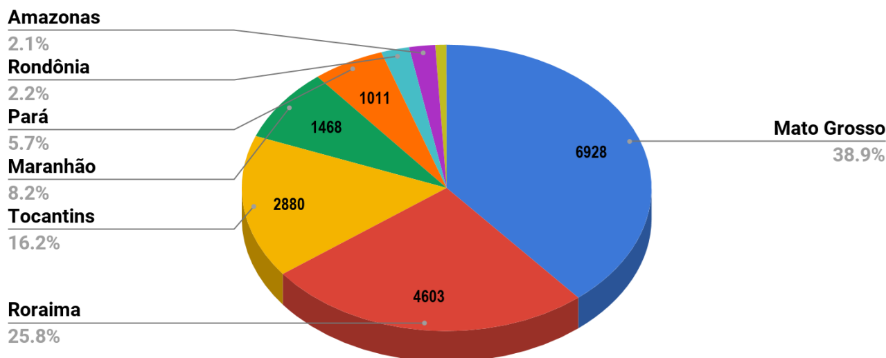
Figura 1 – Distribuição percentual dos focos de queimadas acumulados em 01/01/2019 a 09/07/2019 na Amazônia legal ( Satélite de Referência AQUA Tarde)
