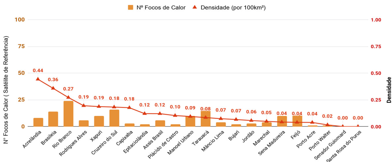
Figura 6 – Ocorrência de focos de queimadas e densidade por km 2 , por município em 01/01/2019 a 09/07/2019 ( Satélite de referência AQUA_M-T)
