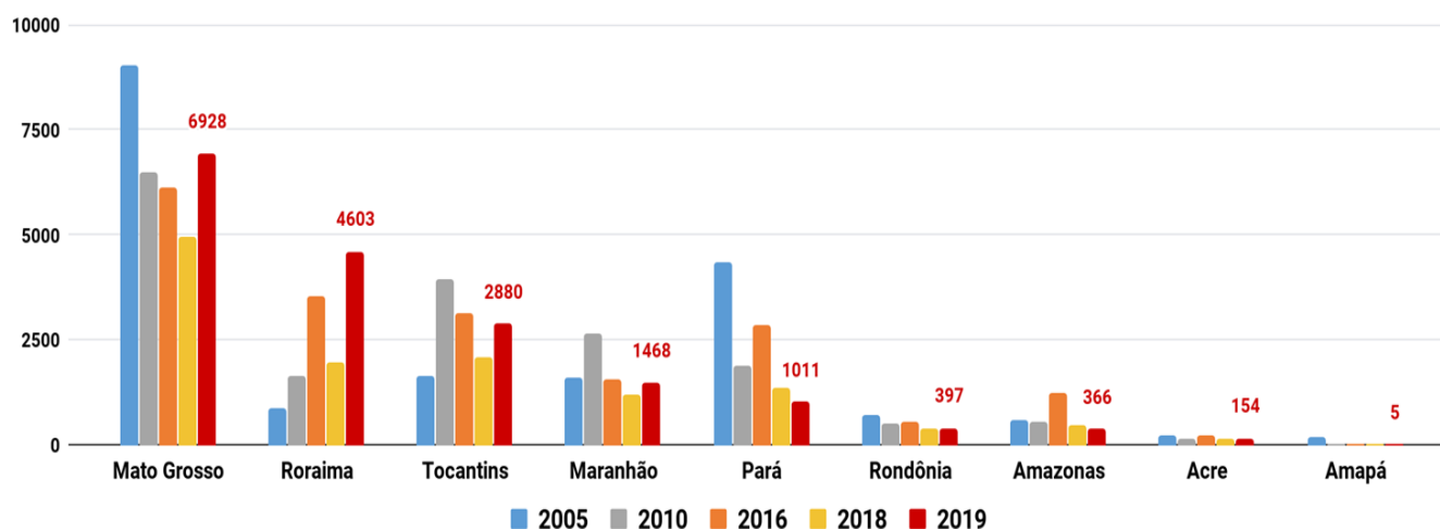
Figura 2 – Distribuição comparativa dos focos de queimadas acumulados de 01/01 a 09/07 na Amazônia legal, nos anos de 2005, 2010, 2016, 2018 e 2019 ( Satélite de Referência AQUA Tarde)
