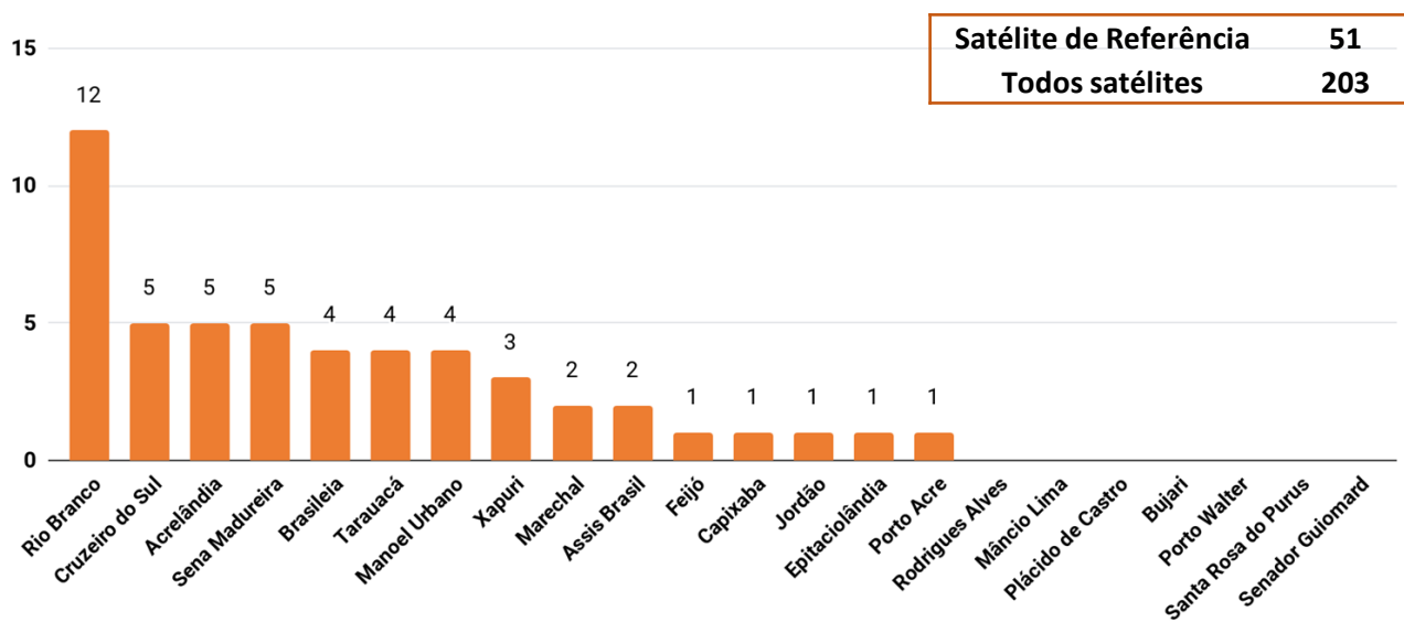
Figura 4 – Distribuição dos focos de queimadas acumulados no mês julho de 01/07/2019 a 09/07/2019. ( Satélite de referência AQUA_M-T)
