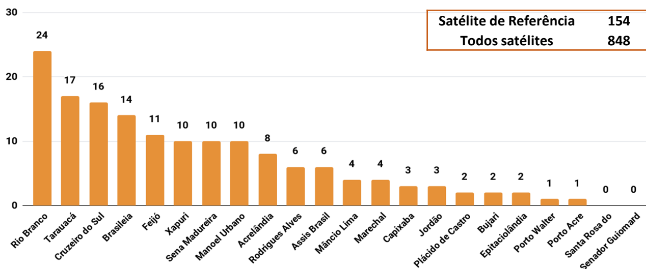
Figura 3 – Distribuição dos focos de queimadas acumulados de 01/01/2019 a 09/07/2019, no Estado do Acre. ( Satélite de referência AQUA_M-T)
